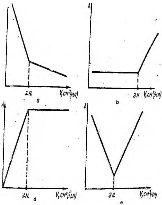
4.15-rasm. Fotometrik titrlash egri chiziqlari
