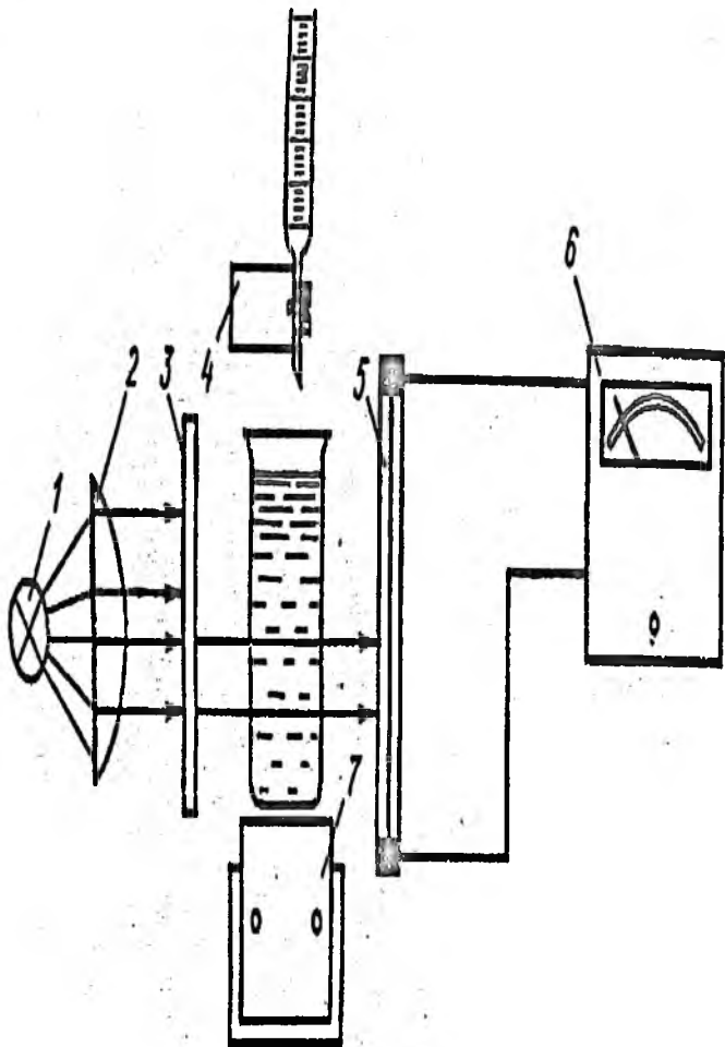
4.17-rasm. Fotometrik titrlash sxemasi
