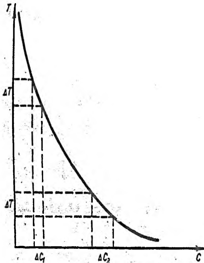
4.8-rasm. Yorug'lik o'tkazish koefitsiyentni T ning S ga bog'liqligi
