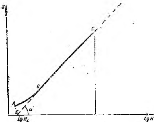
1.4-rasm. Fotoplastinka qorayishining yoritilishga bog'liqlik egri chizig'i
