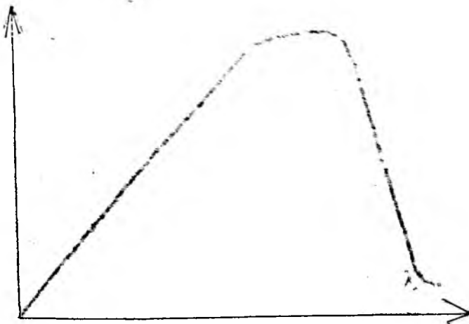
5.12-rasm. Lyuminetsensiya energetik to'liqin uzunliklari
