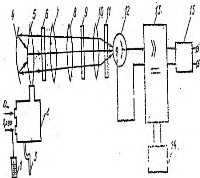
3.5.-rasm. Alangali fotometrning prinsipial sxemasi:
