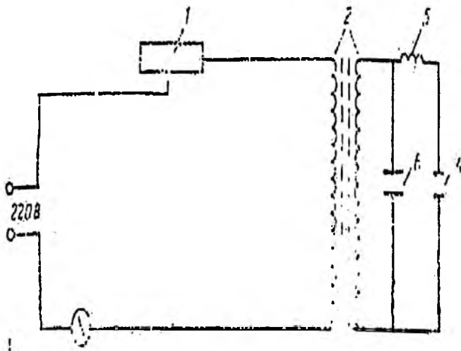
2.4-rasm. Yuqori kuchlanishli zichlangan uchqun bilan ta'minlash sxemasi:
