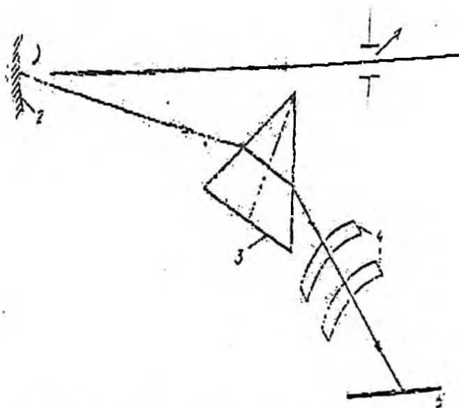
2.2-rasm. ISP - 28 spektrografining optik sxemasi:
