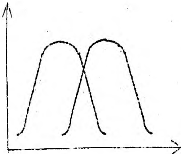
5.11-rasm. Yutilish (1) va lyuminesensiya unumining qo'zg'atuvchi to'lqin (2)spektrlarning qo'zgatuvchi nur uzunligiga bog'liqligi.
