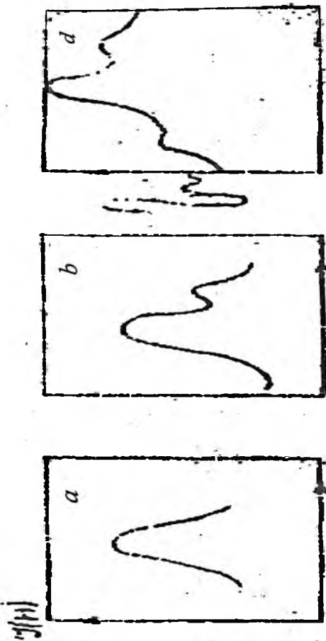
5.17-rasm. EPR-spektrlarining 3 xil ko‘rinishi: a, b, d – yutilish chiziqlari, e, f, g – yutilish spektr chiziqlarining kub. aksial va romb simetriyalarga uyg‘un hosilalari.
