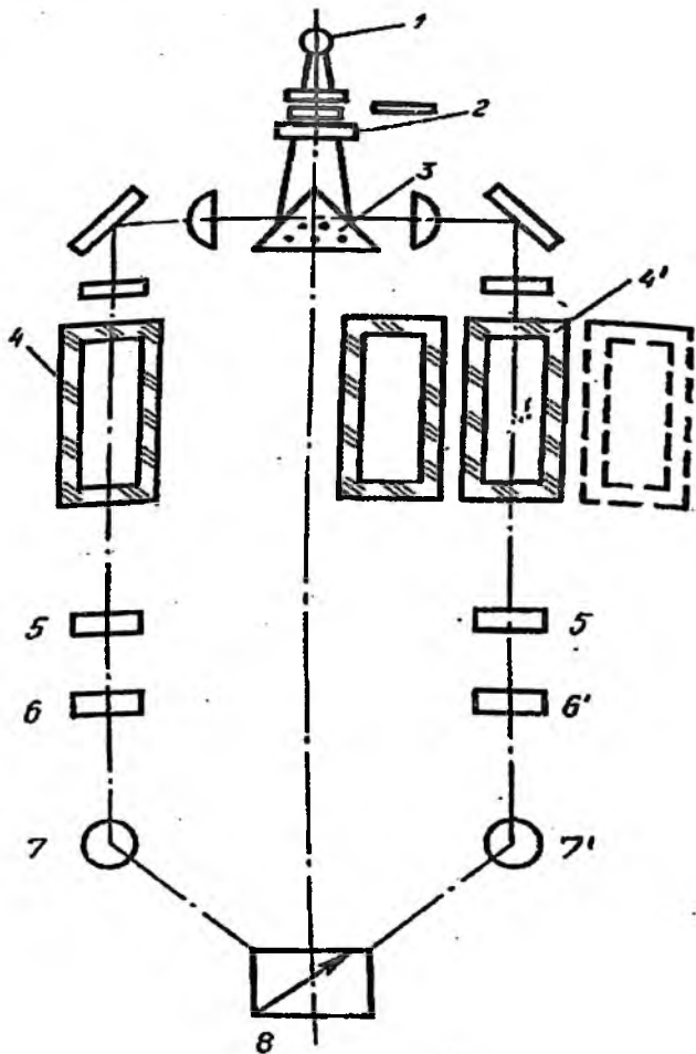
4.14-rasm. FEK-56M fotokalorimetrlarning optik sxemasi
