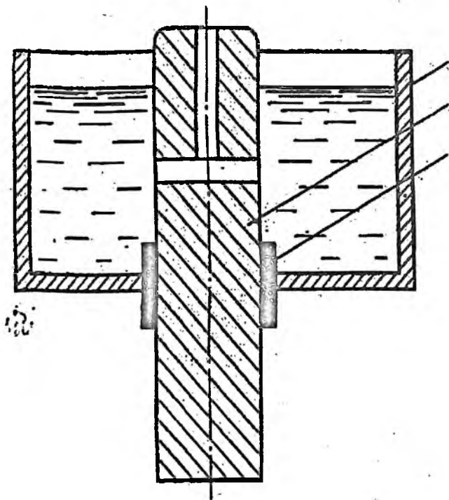
3.3-rasm. Fulgurator: 1—fulgurator idishi; 2—elektrod; 3— qistirma.
