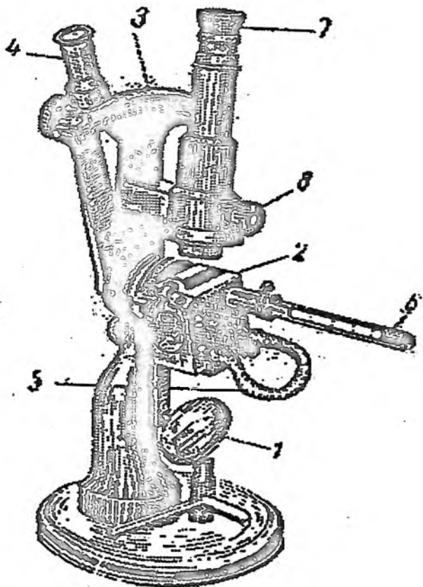
5. 7-rasm. Abbe refraktometrining umumiy ko'rinishi: 1 – ko'zgu; 2 – prizma; 3 – shkala; 4 – lupa; 5 – suv yuborish nayi; 6 – termometr; 7 – okulyar; 8 – kompensator.
