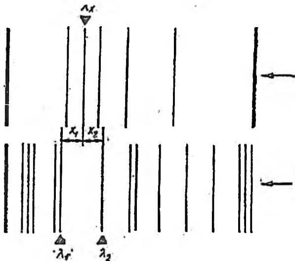
3.1-rasm. Spektral chiziqlar to‘lqin uzunligini interpolyatsiya qilish usuli bilan aniqlash (yuqorida nauna spektri, pastda temir spektri berilgan).
