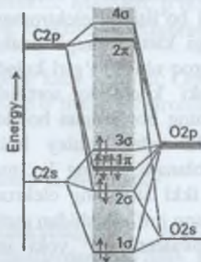
2.13-rasm. CO uchun molekulyar orbitalarning energetik holat diagrammasi.
