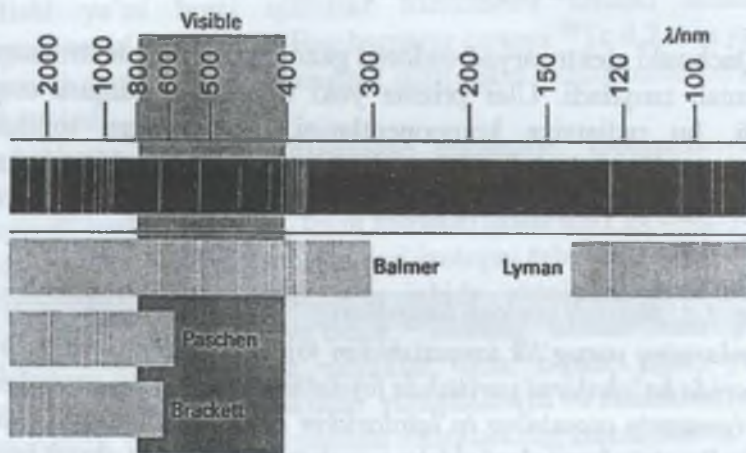
1.2 -rasm. Vodorod atomining spektri va seriyali analizlari
