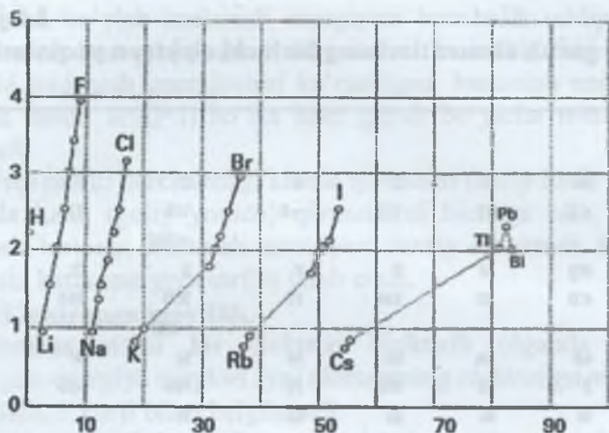
1.25-rasm. Pauli elektromanfiylikning davriy varianti
