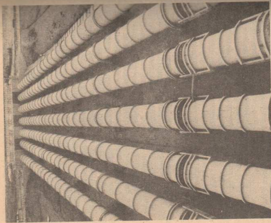
«Искра» насос станцияси Сурхон—Шеробод даштларини сув билан таъминлайди.
