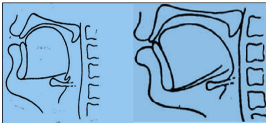
Расми 15. Рентгенограммаи ҳамсадоҳои [ж] ва [ш].
