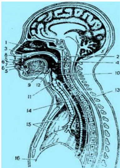
Расми 1. Дастгоҳи гуфтор: 1 – ковокии бинӣ, 2 – коми сахт, 3 – дандонҳо, 4 – лабҳо, 5 – нӯги забон, 6 – рӯи забон, 7 – беҳи (решай) забон, 8 – танояки забоншакл, 9 – халқ, 10 – нои нафас, 11 – шуш, 12 – диафрагма, 13 – ковокии бинӣ, 14 – пардачаи ком (коми нарм), 15 – гулӯ, 16 – сурхрӯда.
