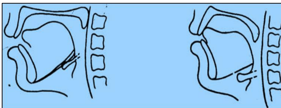
Расми 16. Рентгенограммаи ҳамсадои [p] ва [л]
