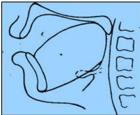
Расми 20. Рентгенограммаи ҳамсадои [қ]
