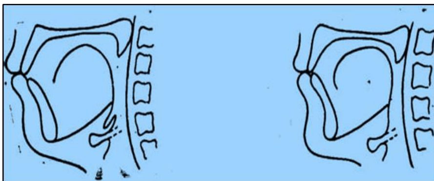
Расми 11. Рентгенограммаҳои ҳамсадоҳои [в] ва [ф]
