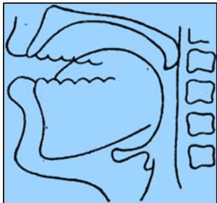
Расми 5. Рентгенограммаи садоноки [ū].
