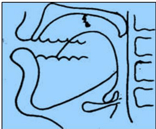
Расми 8. Рентгенограммаи садонокӣ [o].
