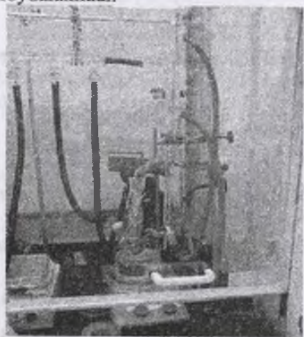
Eterifikatsiya reaksiyasida qo'llaniladigan Din-Stark apparati
