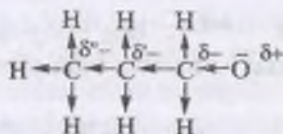
kislorod anionining +I ta'siri
