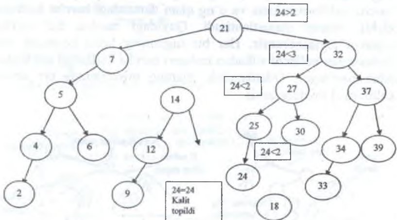
15-chizma. Binar daraxt bo'yicha qidiruv
