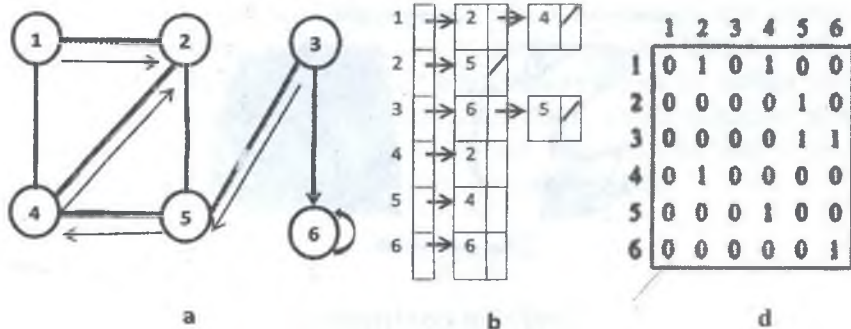
24-chizma. Ikkita oriyentirlangan graf tasviri
