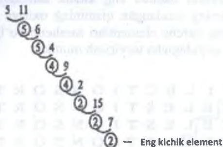
2-chizma. Tanlash usulida saralash
