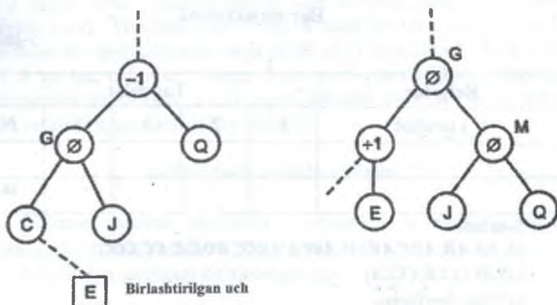
17-chizma. Muvozanatlashgan tugunga ega ko'rsatkichli daraxt
