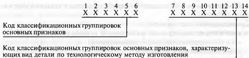
Рис. 18.13. Структура общего кода детали по методу изготовления
