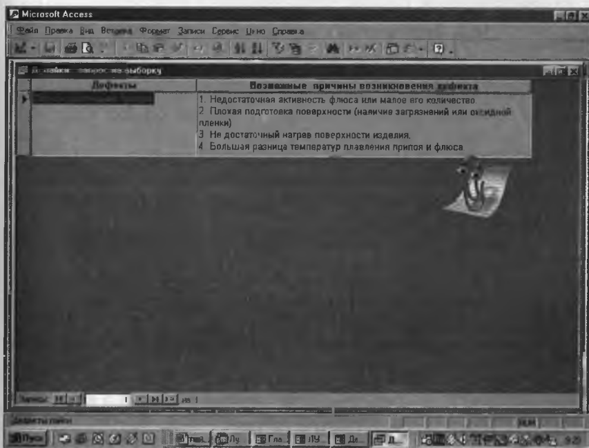
Рис. 18.12. Возможные причины дефекта паяного соединения
