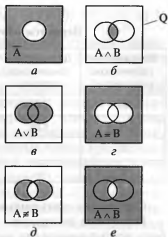
Рис. 1.4. Графическое изображение булевых функций:
