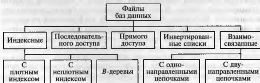
Рис. 3.2. Классификация файловых структур
