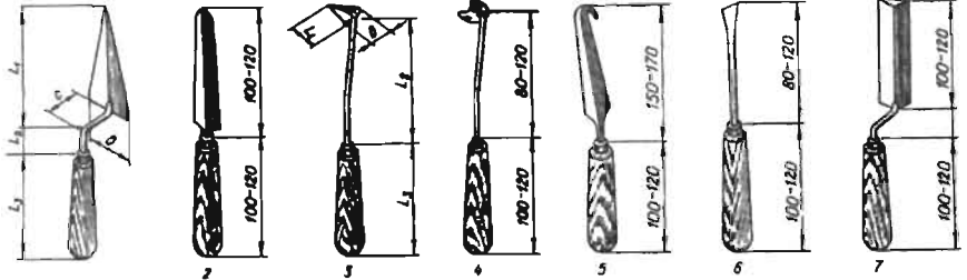
Ganch o'ymakorligida asboblarning o'lchamlari: 1. Shuturgardon; 2. Qalamtoq; 3. Minqor; 4. Morpech; 5. Pux qalam; 6. Iskana; 7. Patak binni.
