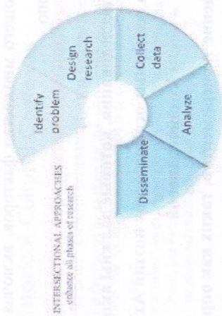
Рисунок 3.4. Межсекционный анализ.
