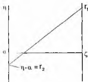
22-rasm. Kelen-Tyudiyosh usuli bilan r_1 va r_2 ni aniqlash grafigi.
