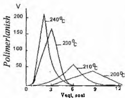
30-rasm. \epsilon -kaprolaktamning 2,0% suv ishtirokida har xil haroratdagi polimerlanish tezligi.
