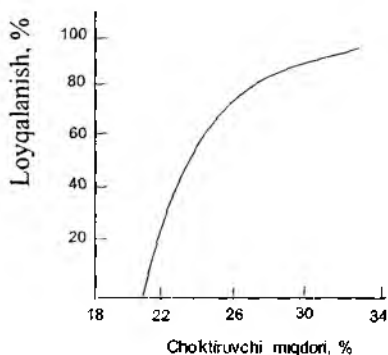
60-rasm. Turbidimetrik titrlashning tipik egrisi
