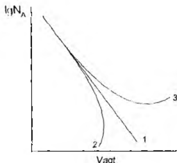
121-rasm. «Qo'shni effekti» kuzatiladigan reaksiyalarning kinetik egri chiziqdaru:
