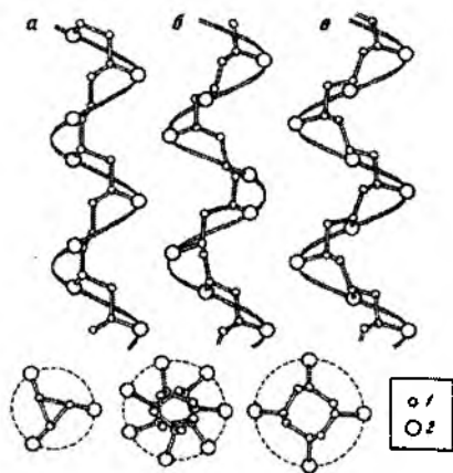
96 - rasm. Izotaktik vinil polimerlarning spiral strukturasi. a - 3_1 - spiral; b - 7_2 - spiral; c - 4_1 - spiral; 1 - asosiy zanjirni hosil qiluvchi uglerod atomlari; 2 - takroriy uglerod atomlariga birikkan R - o'rindosh. Tasvirni soddalashtirish uchun uglerod atomlariga birikkan vodorod atomlari ko'rsatilmagan.
