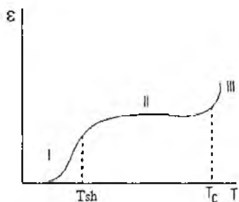
105 – rasm. Amorf polimerning termomexanik egri chizig'i. 1-shishasimon holat; 2 – yuqori elastik holat va 3– qovushqoq – oquvchan holat oralig'qlari.
