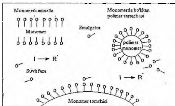
16-rasm. Emulsion polimerlanuvchi sistemaning soddalashtirilgan sxematik tasyiri.
