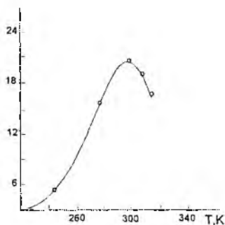
122-rasm. Xlormetil reaksiyasi boshlang'ich tezligining haroratga bog'liqligi.
