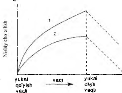
109-rasm. Doiniy kuch ta'sirida polimer namunasi nisbiy uzayishining o'zgarishi (B-kuch qo'yilish daqiqasi; A-kuchning olinish vaqti). 1-chiziqsimon polimer; 2-to'rsimon polimer.
