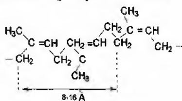
Sis-izomer (kauchuk)
