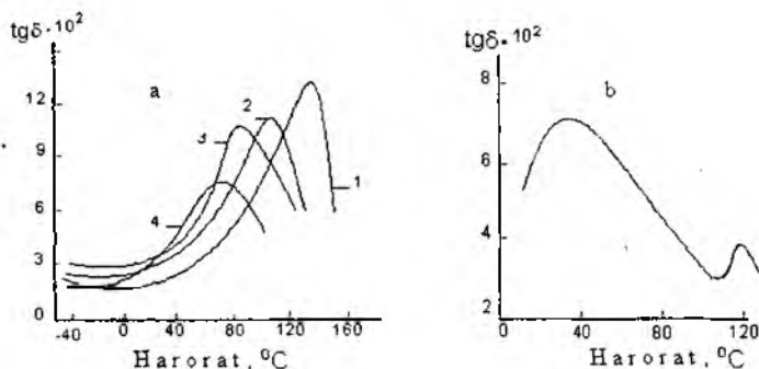
132-rasm. Polivinil spirtining ba'zi atsetallari (a) va polimetilmetakrilat (b) uchun tg\delta ning haroratga bog'liqligi: 1 – etilal; 3 – propilal; 3 – butiral; 4 – oktital.
