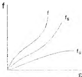
108 – rasm. Tabiiy kauchukka 20°C da ta'sir etuvchi kuch ( f ) va uning energetik ( f_u ) hamda entropiya ( f_s ) omillarining deformatsiya darajasi ( \varepsilon ) ga bog'liqligi
