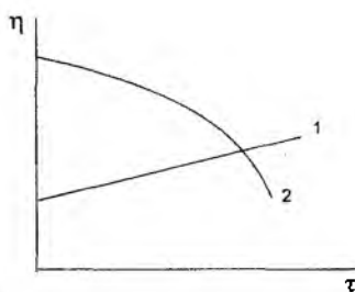
112 – rasm. Polimerlar qovushqoqligi-ning siljish kuchlanishiga bog‘liqlik turlari. 1 – Nyuton suyuqligi; 2 – psevdoplastik suyuqlik uchun.
