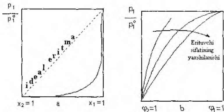
48-rasm. Polimer eritmasi ustidagi erituvchi bug' bosimining komponentlar mo'l (a) va \varphi -hajmiy (b) ulushlariga bog'liqligi.
