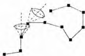
38-rasm. Belgilangan (fiksatsiyalangan) valent burchakli zanjir konformatsiyalari.
