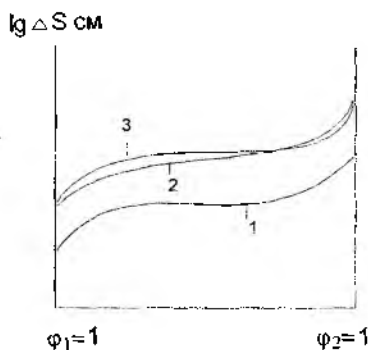
52-rasm. Tabiiy kauchuk-benzol sistemasi uchun aralashish entropiyasining eritma tarkibiga bog'liqligi:
