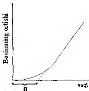
126-rasm. Yacheyka ichiga parda orqali diffuziyalangan gaz bosimining vaqtga bogʻliqligi.
