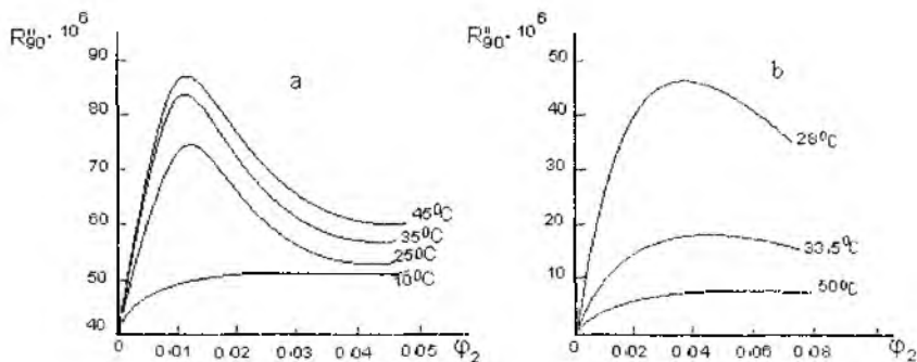
76-rasm. Ortiqcha yorug'lik yoyilishning ( R_{90}'' ) eritmada polimerning hajmiy ulushiga bog'liqligi: a – polistirol yaxshi erituvchi – benzolda; b – polistirol yomon erituvchi – siklogeksanda.
