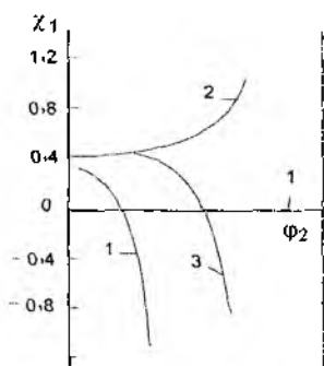
54-rasm. \chi_1 parametrning polimerning hajmiy ulushiga bog'liqligi: 1-nitrat tsellyulozaning asetondagi eritmasi; 2-nog'ovak polimer eritmasi; 3-g'ovak polimer eritmasi.
