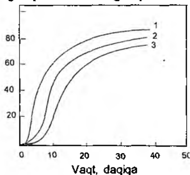
123-rasm. Polimetilmetakrilat depolimerlanishining qizdirish vaqtiga bog'liqligi:
