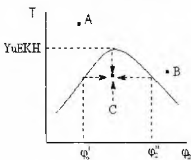
45-rasm. YuKEH li sistema uchun harorat – tarkib egrisi.
