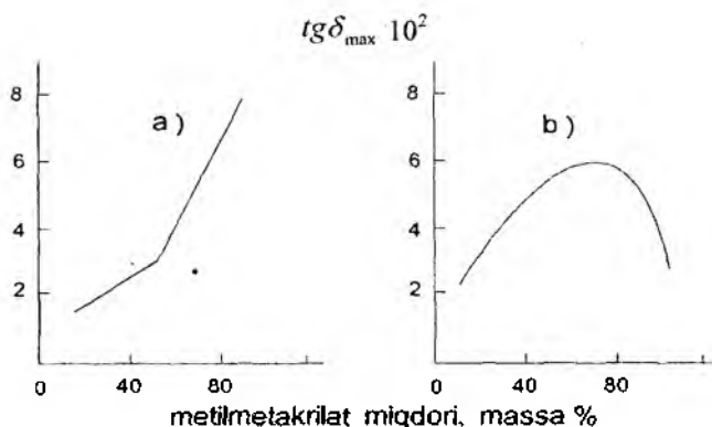
133-rasm. tg\delta_{\max} ning sopolimerdagi stirok-metilmetakrilat nisbatiga bog'liqligi: a – 400 Gts dagi dipol-guruhli yo'qotish; b – 20 Gts dagi dipol-segmental yo'qotish.
