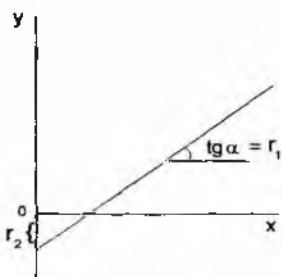
21-rasm. Sopolimerlanish konstantalari r_1 va r_2 larni Faynemann-Ross usuli bilan aniqlash.
