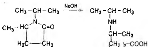
N-izopropil- \gamma - valerofaktam
