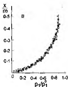
131-rasm. n-geksanning yuqorielastik polimerlarga sorbsiyalanish izotermasi: o – tabiiy kauchuk; x – butadien sintetik kauchugi; • – izopren sintetik kauchugi (SKI); Δ – SKI ning yuqori-molekulyar fraksiyalari; + – sintetik kauchuk SK-1; ○ – CK-2.
