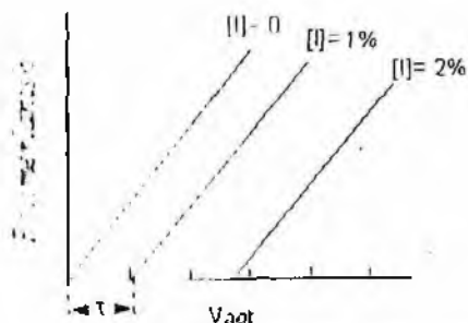
10-rasm Polimerlanish tezligiga ingibitor konsentratsiyasining ta'siri.
