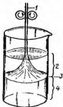
28-rasm. Fazalar orasidagi sirtidan hosil bo'lgan poliamid tolasini uzluksiz chiqarib olish: 1 – yassi parda; 2 – diamin va asosning suvli eritmasi; 3 – fazalar orasida hosil bo'lgan polimer parda; 4 – dioxlorangidridning organik erituvchidagi eritmasi.
