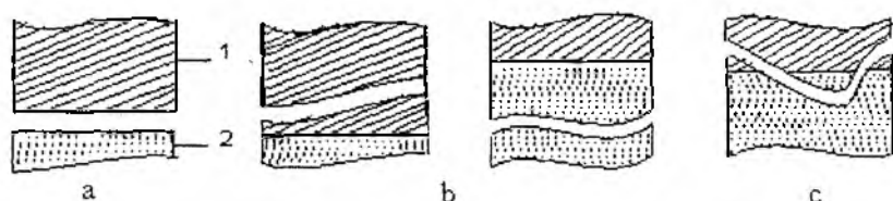
119 – rasm. Adgezion birikmaning emirilish sxemasi: 1 – adgeziv; 2 – substrat; a – adgezion emirilish; b – kogezion emirilish; c – aralash emirilish.
