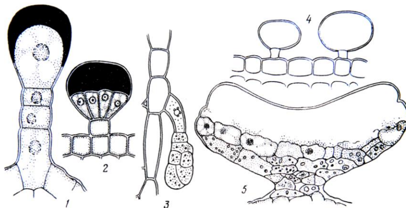
17-rasm. Bezli tukchalar:
