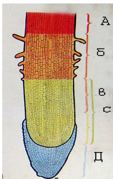
19 - rasm. Ildizning zonalari:
