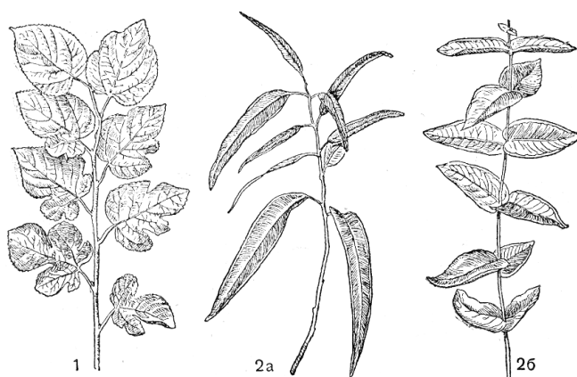
39-rasm. Geterofilliya: 1 – tut; 2a - 2b – evkalipt.
