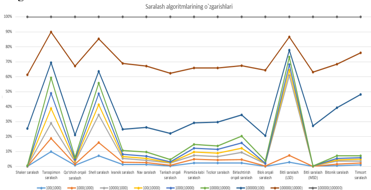
8.4-rasm. Saralash algoritmlarini o'zini tutishi.
