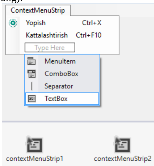
10.14-rasm. Oynada kontekst menyuga ishlov berish.
