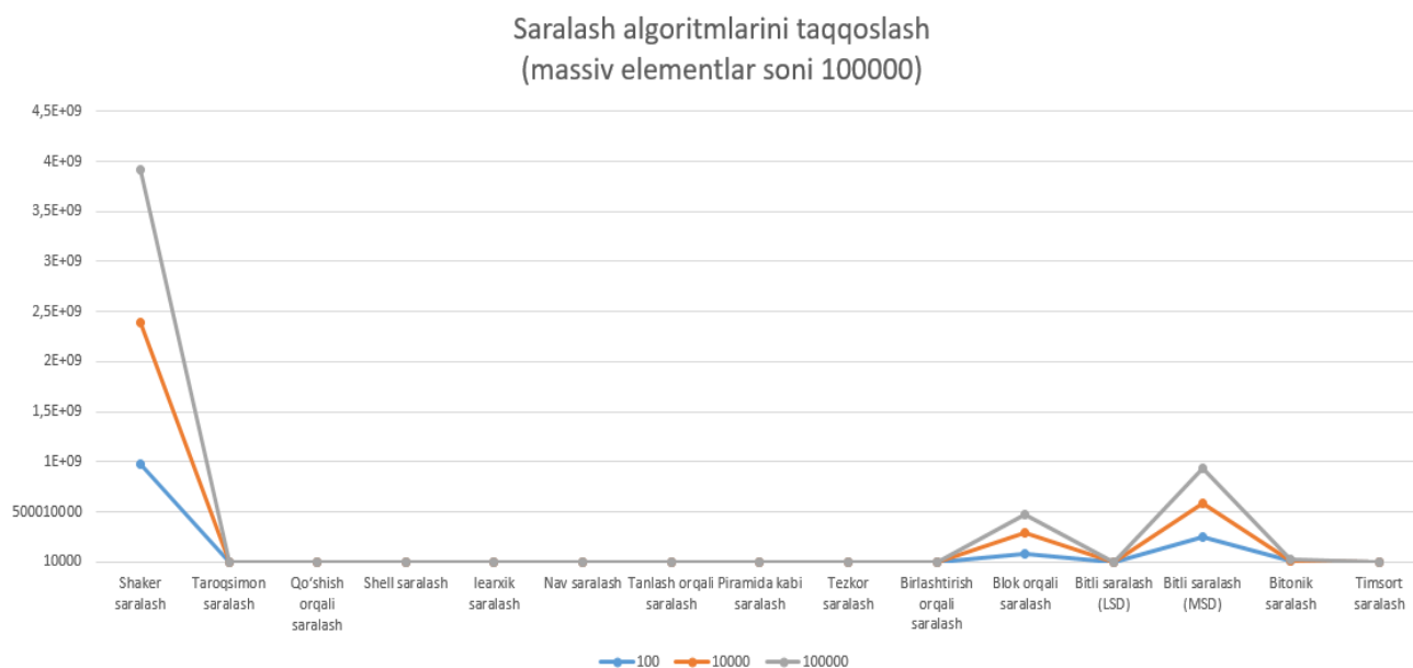
8.3-rasm. Saralash algoritmlarini taqqoslash.
