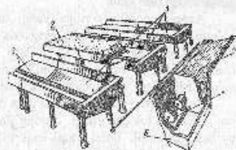
42-rasm. Ekiniga bosim ostida eritmani berish shag'alni moslamasi shakli. 1 - me'yordan; 2 - shag'al to'liq shag'al; 3 - suv va oziqali eritma rezervuari; 4 - oziqali eritma qochiruvchi nasos; 5 - nazorat paneli; 6 - namlik qadag'i
