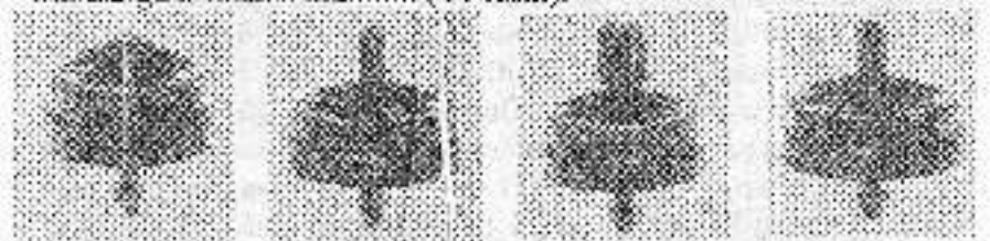
Bosimni kompensatsiyalaydigan (tiklaydigan) tomchilatib sug'orish moslamasi. Suv sarfi: 2, 4, 8, 5 l/s Bosimni kompensatsiyalaydigan (tiklaydigan) «dyatels» tipidagi tomchilatib sug'orish moslamasi. Suv sarfi: 2, 4, 8, 5 l/s Bosimni kompensatsiyalaydigan, ko'pikli tomchilatib sug'orish moslamasi. Suv sarfi: 25 l/s C.A.L. YUqori bosimni kompensatsiyalaydigan tomchilatib sug'orish moslamasi. Suv sarfi: 3, 6, 12 l/s. O'zgaruvchi bosim: 4 m.
