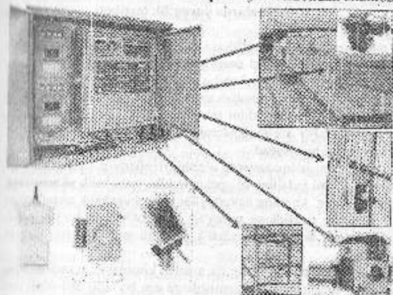
18-rasm. Issiqxonalarda mikroiklimni avtomatik sozlash
