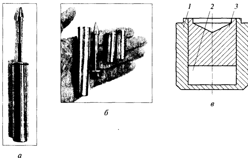
Рис. 10.8. Источник нейтронного излучения:
