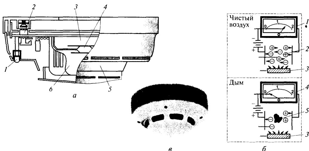
Рис. 10.7. Детектор дыма:
