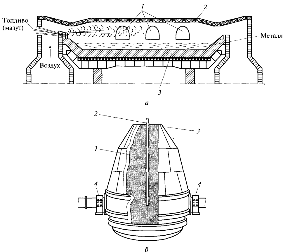
Рис. 6.7. Сталелитейное производство:
