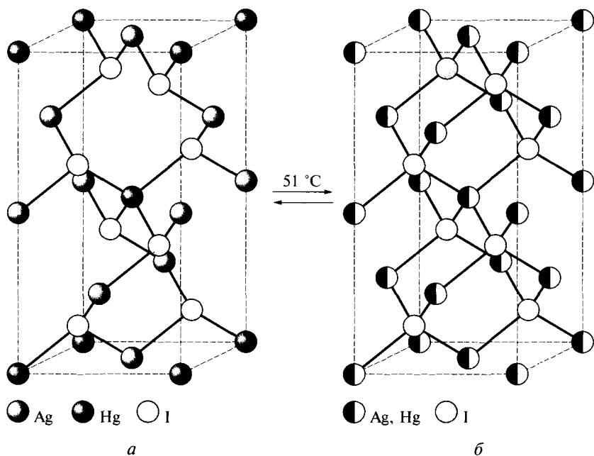
Рис. 8.21. Взаимные превращения желтой \beta ( a ) и красной \alpha ( b ) модификаций \text{Ag}_2[\text{HgI}_4]
