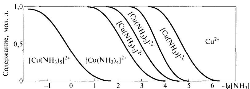
Рис. 7.26. Зависимость содержания различных аммиокомплексов меди(II) в водных растворах от молярной концентрации аммиака
