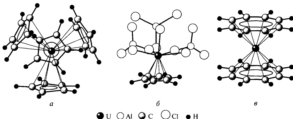
Рис. 10.17. Строение молекул:
