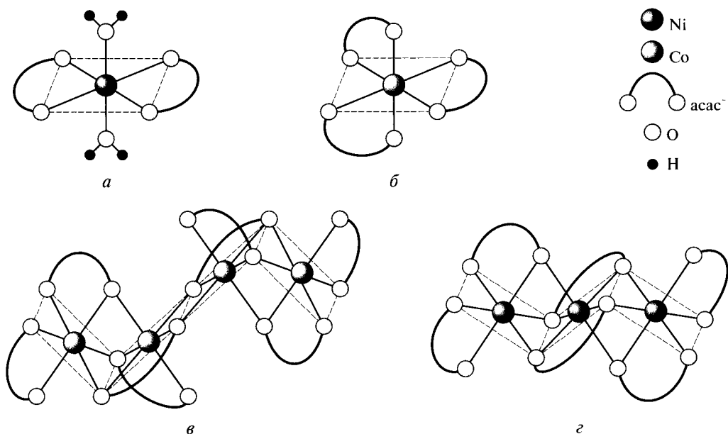
Рис. 6.40. Структура ацетилацетонатов кобальта и никеля: a - M(acac)_2(H_2O)_2 ( M = Co, Ni ); b - Co(acac)_3 ; в - Co_4(acac)_8 ; г - Ni_3(acac)_6
