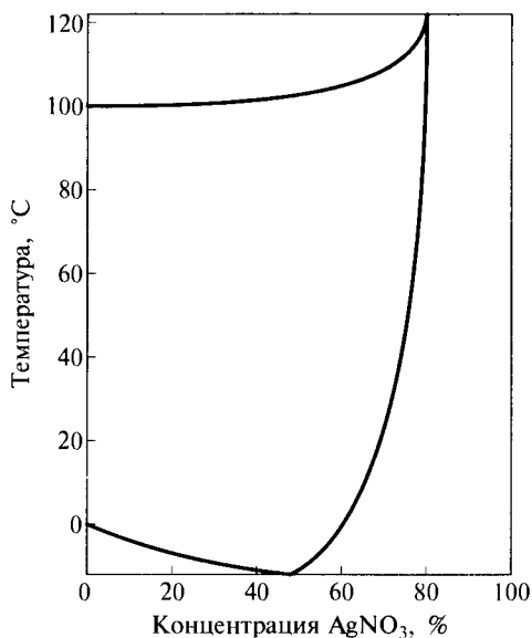
Рис. 7.15. Растворимость нитрата серебра в воде
