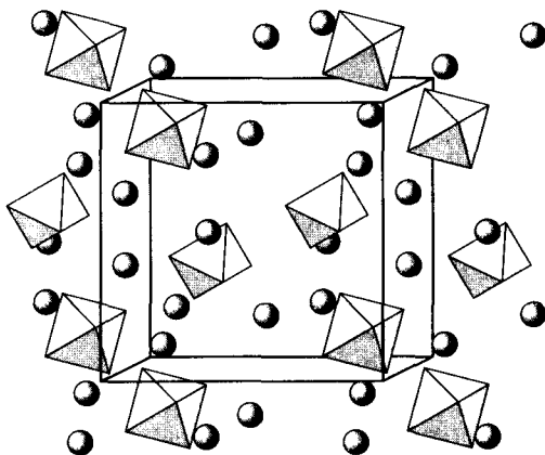
Рис. 6.13. Строение комплексного гидрида \text{Li}_3[\text{RhH}_6]
