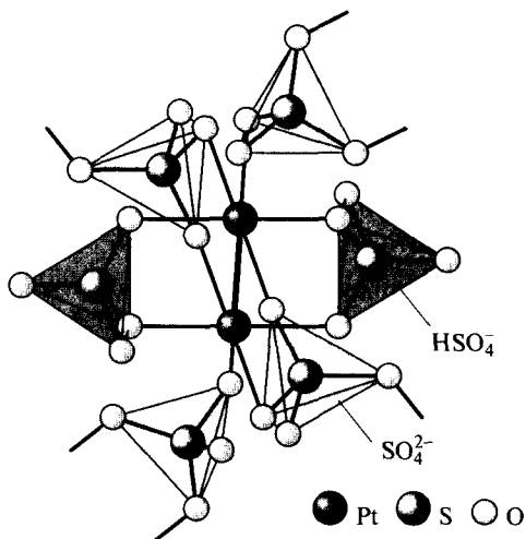
Рис. 6.61 Строение комплекса \text{Pt}_2(\text{HSO}_4)_2(\text{SO}_4)_2
