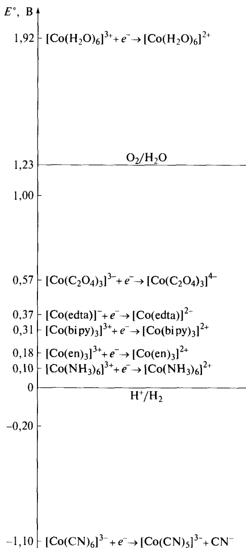
Рис. 6.39. Зависимость стандартного электродного потенциала Co^{3+}/Co^{2+} от природы лиганда (показана область термодинамической устойчивости воды)
