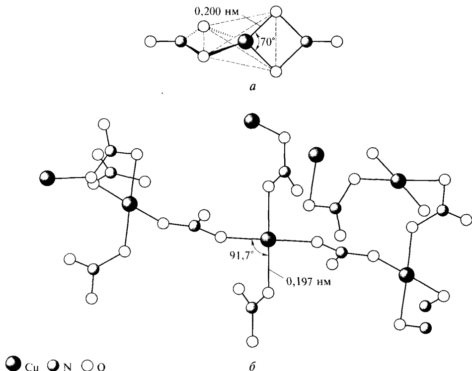
Рис. 7.24. Строение нитрата меди(II): а — в парях; б — в кристалле (β-модификация)
