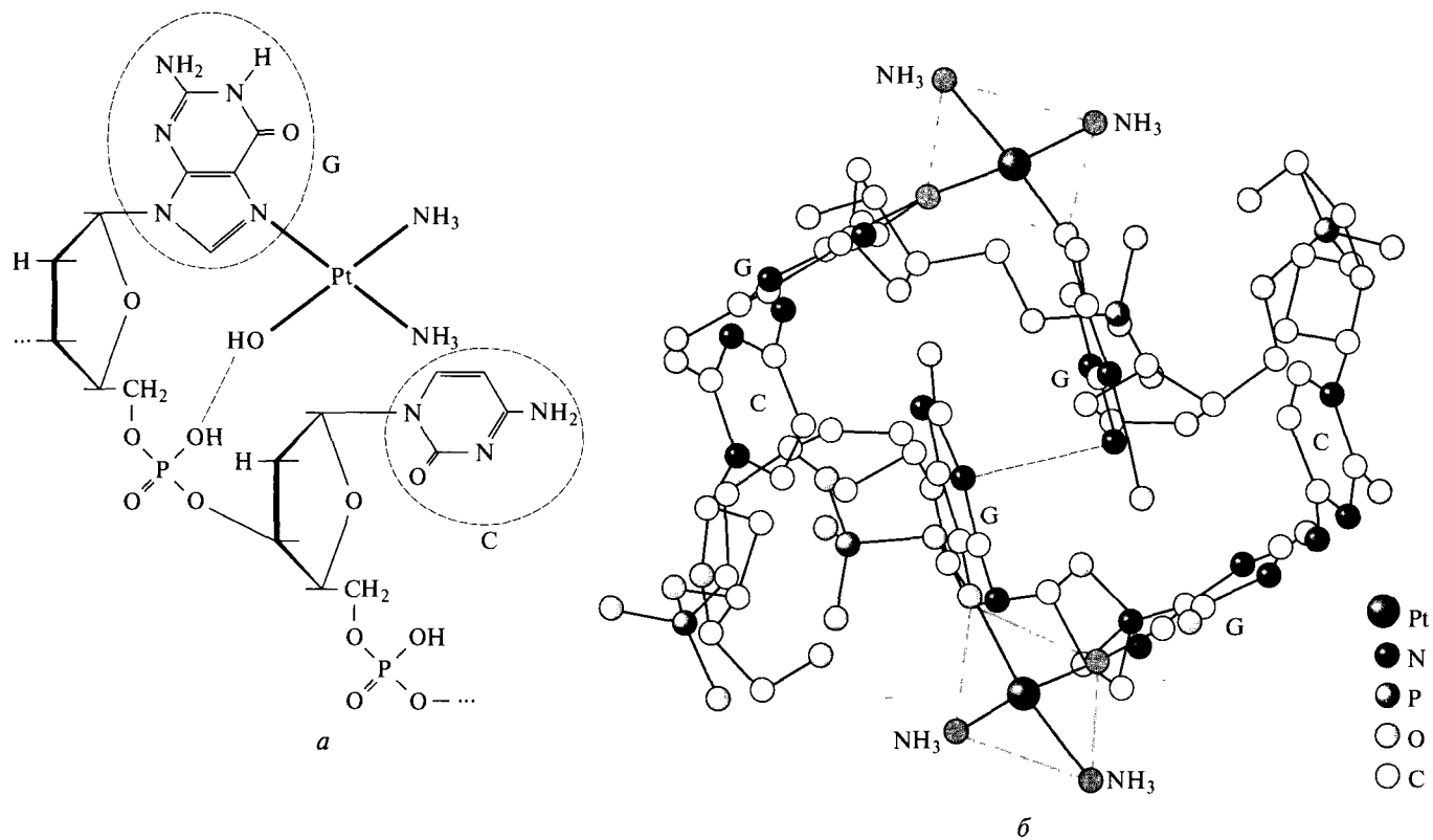
Рис. 6.54. Структура комплекса гуанина с цис -диамминдихлороплатиной(II):
