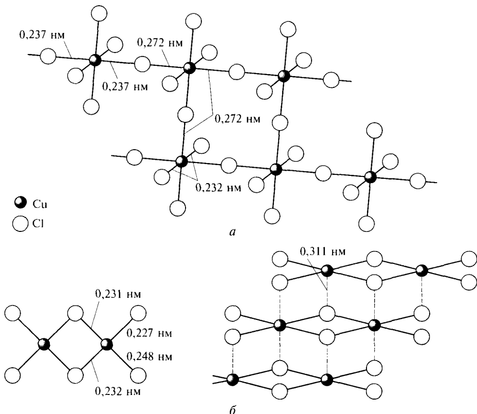
Рис. 7.29. Строение хлорокупратов(II):
