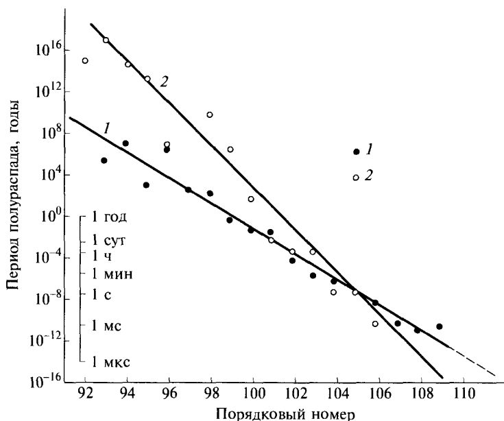
Рис. 10.28. Времена жизни актиноидов и трансактиноидов при \alpha -распаде (1) и спонтанном делении ядра (2)
