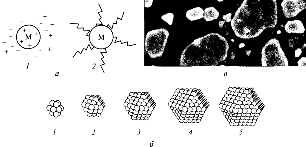
Рис. 7.42. Кластеры металлов:
