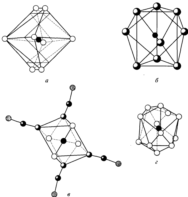
Рис. 9.5. Координационные полиэдры в соединениях лантаноидов: а — куб ( \text{La}_2\text{Zr}_2\text{O}_7 ); б — трехшапочная тригональная призма ( [\text{Nd}(\text{H}_2\text{O})_9]^{3+} в кристаллической структуре бромата неодиима); в — прямоугольная антипризма ( \text{K}_4[\text{Nd}(\text{NCS})_7(\text{H}_2\text{O})_4] ); г — икосаэдр ( \text{La}_2(\text{SO}_4)_3 \cdot 9\text{H}_2\text{O} )
