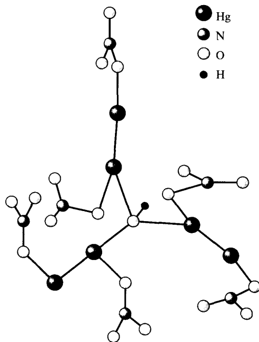
Рис. 8.8. Фрагмент структуры \text{Hg}_4(\text{OH})(\text{NO}_3)_3
