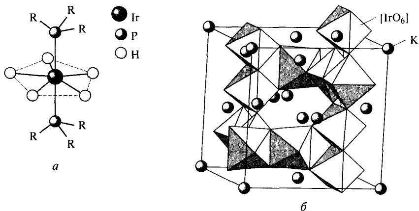
Рис. 6.45. Строение соединений иридия(V): а — \text{IrH}_5(\text{PR}_3)_2 ; б — \text{KIrO}_3
