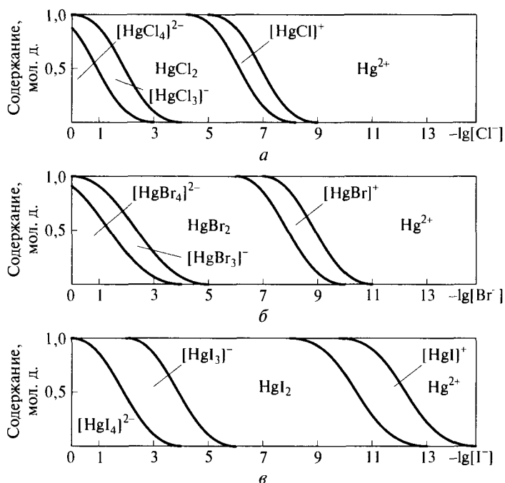
Рис. 8.20. Содержание различных форм в насыщенных растворах хлорида (а), бромид-а (б) и иодида (в) ртути(II) при температуре 25 °С в зависимости от концентрации галогенид-ионов
