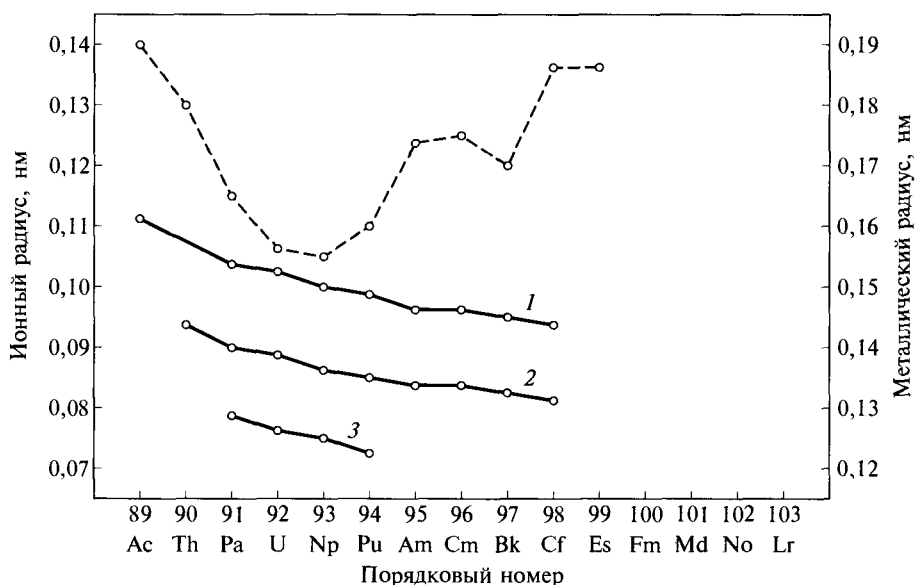
Рис. 10.5. Изменение металлического (пунктирная линия) и ионных (сплошные линии) радиусов актиния и 5f-элементов:
