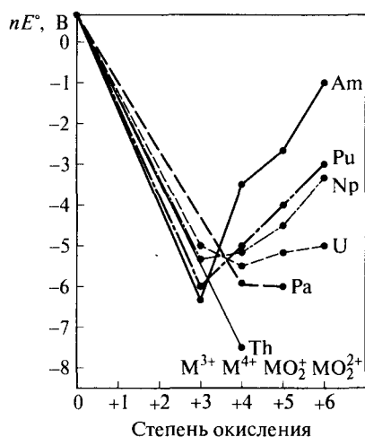
Рис. 10.3. Диаграмма Фроста для актиноидов
