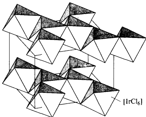
Рис. 6.64. Строение α-IrCl 3
