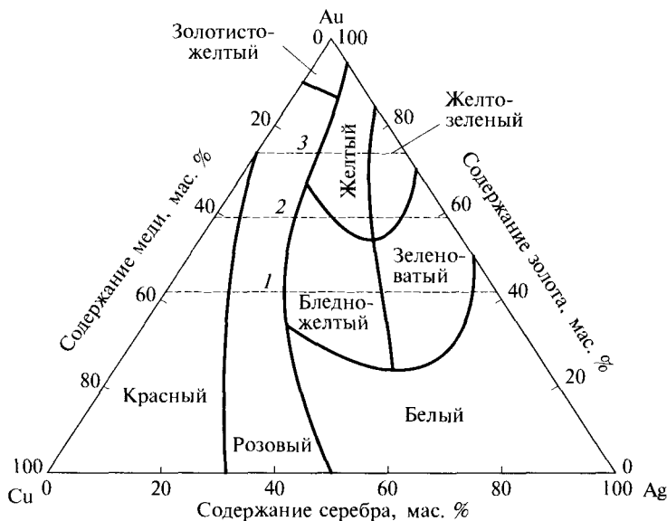
Рис. 7.5. Окраска твердых растворов в тройной системе золото—серебро—медь (пунктирными линиями показаны сплавы, содержащие 10 (1), 14 (2), 18 (3) карат золота)
