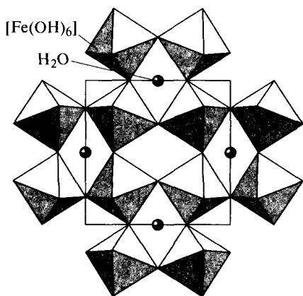
Рис. 6.25. Структура минерала берндтита \text{Fe}(\text{OH})_3(\text{H}_2\text{O})_{1/4}
