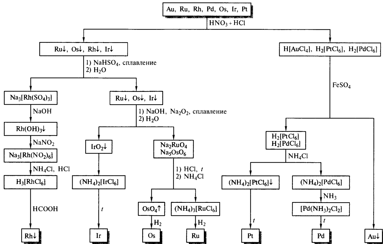
Рис. 6.9. Упрощенная схема аффинажа благородных металлов
