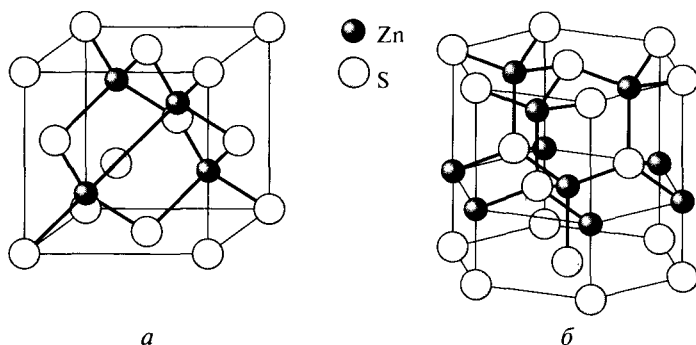
Рис. 8.25. Полиморфные модификации сульфида цинка ZnS :
