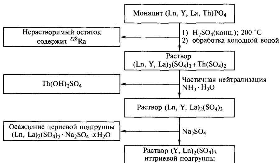
Рис. 9.8. Принципиальная схема сернокислотного вскрытия монацита
