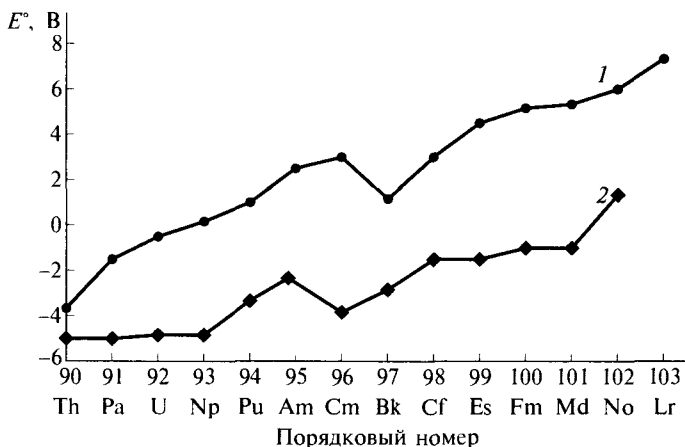
Рис. 10.2. Изменение стандартных электродных потенциалов E^\circ(\text{An}^{4+}/\text{An}^{3+}) (1), E^\circ(\text{An}^{3+}/\text{An}^{2+}) (2) в ряду 5f-элементов
