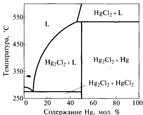
Рис. 8.23. Фазовая диаграмма состояния системы \text{HgCl}_2\text{—Hg} (с упрощениями)
