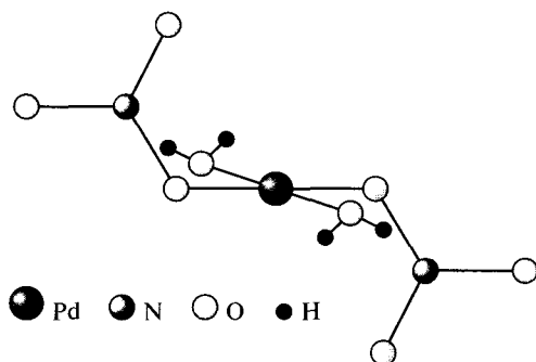
Рис. 6.51. Строение \text{Pd}(\text{NO}_3)_2(\text{H}_2\text{O})_2
