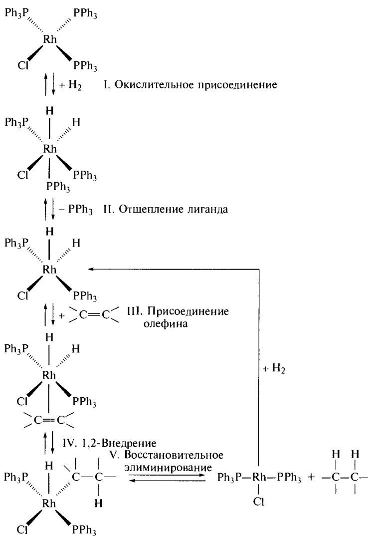
Рис. 6.33. Схема каталитического цикла гидрирования олефинов с помощью катализатора Уилкинсона
