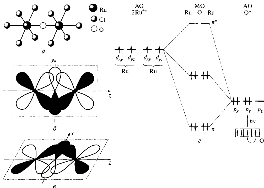
Рис. 6.29. Строение иона [Cl_5Ru—O—RuCl_5]^{4+} (а); перекрывание орбиталей в плоскостях yz (б) и xz (в); диаграмма молекулярных орбиталей, объясняющая образование трехцентровой связи Ru—O—Ru (г) (показаны лишь d -орбитали атомов рутения, участвующие в образовании трехцентровых связей)
