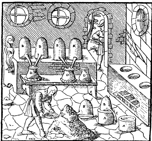
Рис. 8.1. Получение ртути (гравюра из трактата Г. Агриколы «De re metallica»). Горшки с рудой (А) помещены в отверстия печи. Каждый горшок закрыт крышкой (В) с длинной насадкой (С) и замазан. Ртуть собирают в тыквообразные глиняные сосуды (D)
