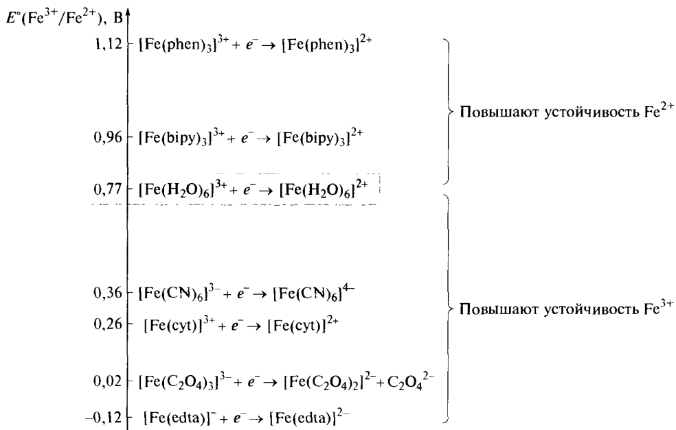
Рис. 6.23. Изменение потенциала пары \text{Fe}^{3+}/\text{Fe}^{2+} в различных комплексных соединениях (cyt — цитохром c)
