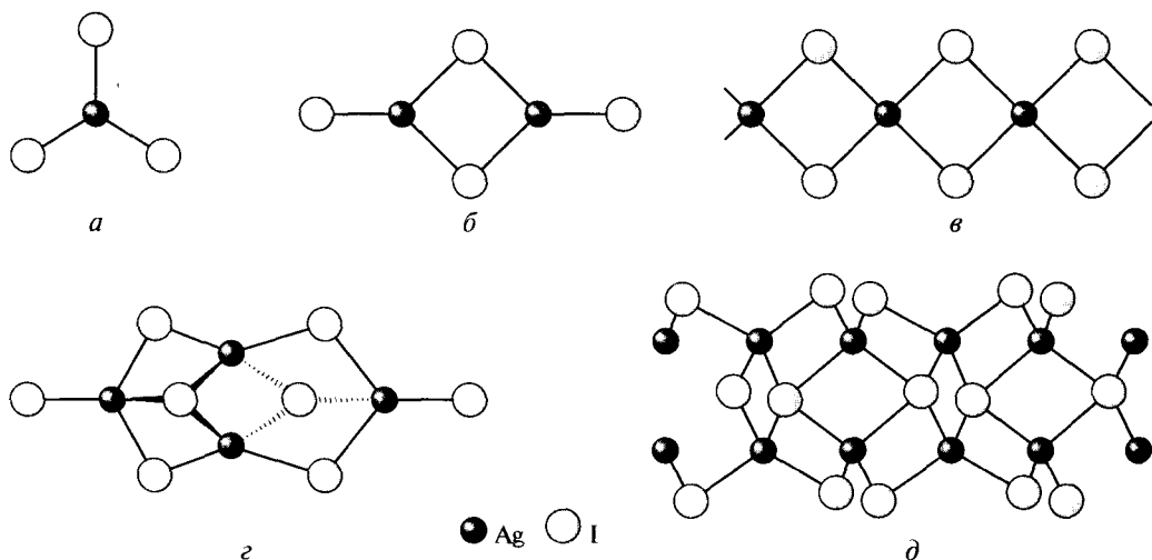
Рис. 7.17. Строение иодоаргентатов(I):
