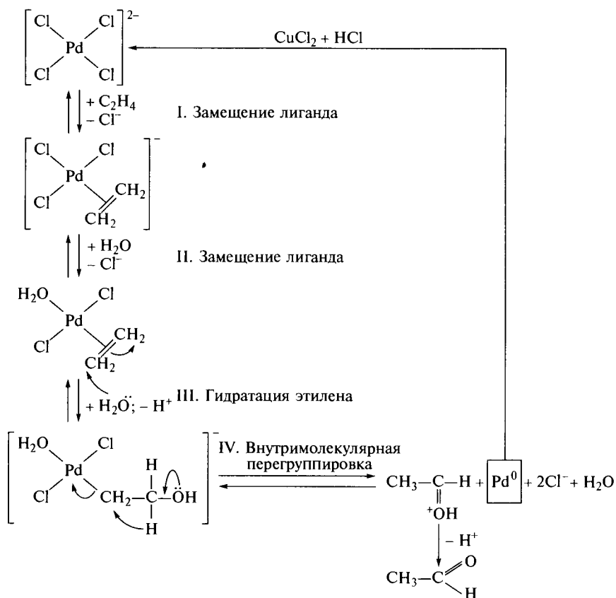
Рис. 6.57. Механизм Вакер-процесса
