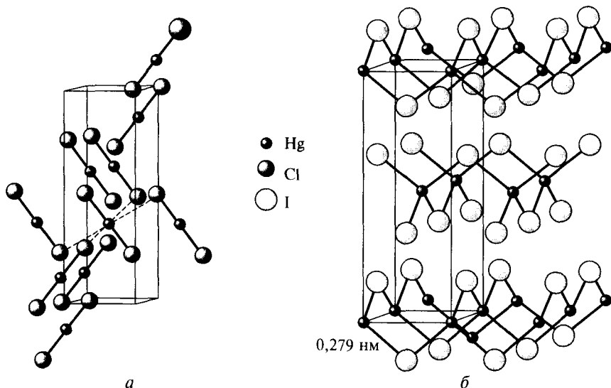
Рис. 8.18. Строение галогенидов ртути(II): \text{HgCl}_2 (а); \alpha\text{-HgI}_2 (б)
