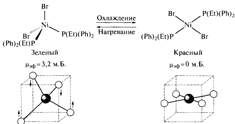
Рис. 6.49. Изомеризация бромидного комплекса никеля(II) с этилдифенилфосфином [NiBr 2 (P(Эт)(Ph) 2 ) 2 ]
