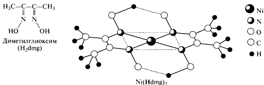
Рис. 6.48. Строение диметилглиоксимата никеля Ni(Hdmg) 2
