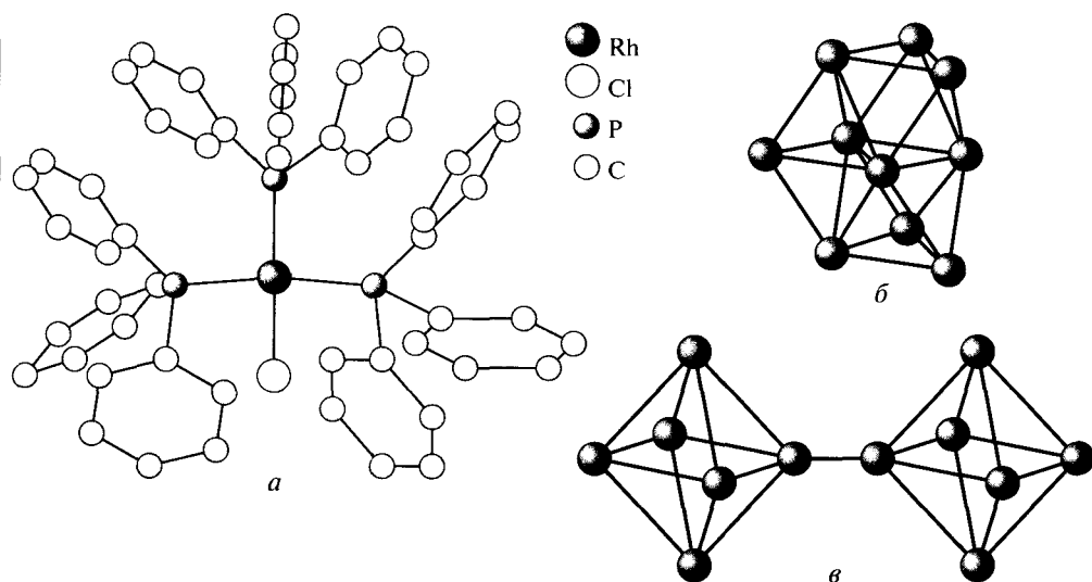
Рис. 6.32. Строение катализатора Уилкинсона (а); каркас из атомов родия в карбонилах [\text{Rh}_{10}(\text{CO})_{21}]^{2-} (б) и [\text{Rh}_{12}(\text{CO})_{30}]^{2-} (в)
