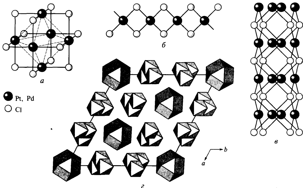
Рис. 6.65. Строение хлоридов палладия и платины: a — \beta - MCl_2 ( M = Pd, Pt ); б — \alpha - PdCl_2 ; в — \alpha - PtCl_2 ; г — PtCl_3
