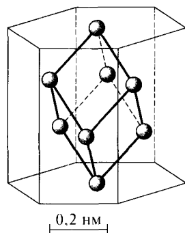
Рис. 8.3. Строение α-ртути
