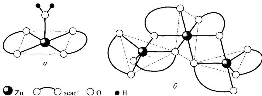
Рис. 8.11. Строение ацетилацетоната цинка: а — \text{Zn}(\text{acac})_2(\text{H}_2\text{O}) ; б — \text{Zn}_3(\text{acac})_6
