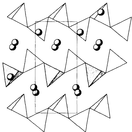
Рис. 7.16. Строение \text{Ag}_2\text{SiO}_3
