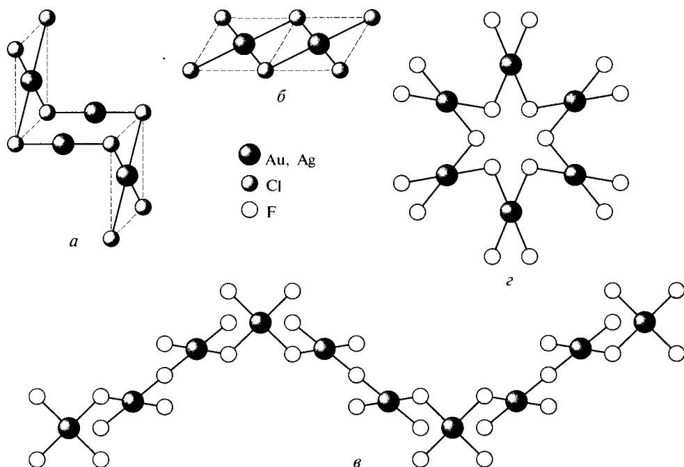
Рис. 7.40. Строение галогенидов золота и серебра:
