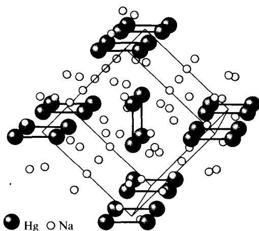
Рис. 8.5. Строение амальгамы натрия Na 3 Hg 2
