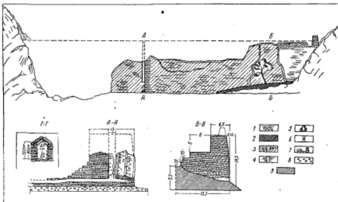
Abdullaxonbandining fasadi va ko'ndadalong kesimlari 27
