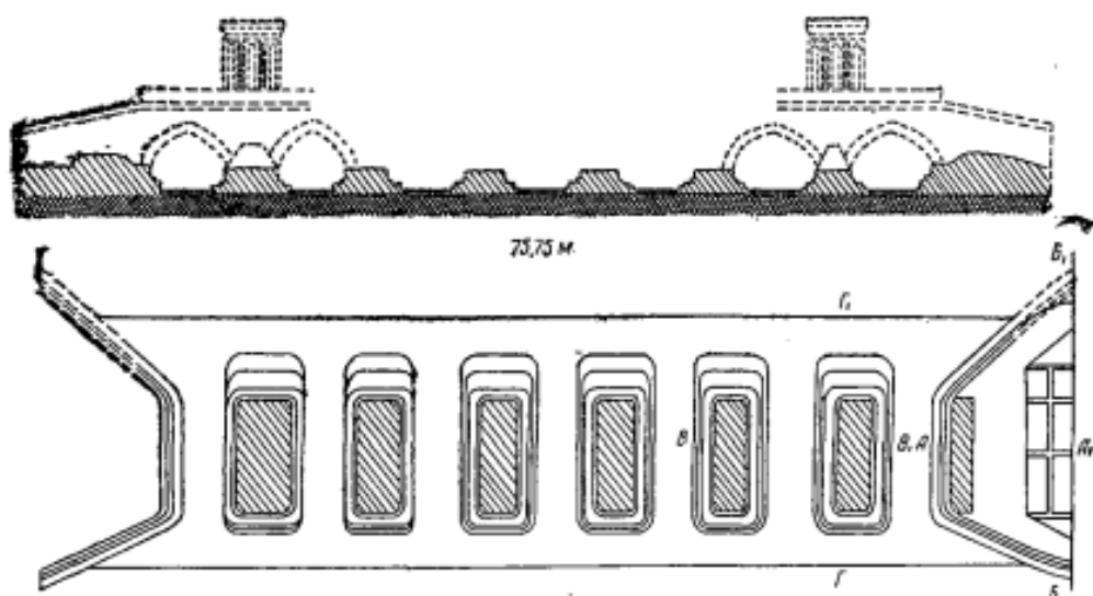
Chahor Minor ko'prigining plani va ko'ndalang kesimi. 28
