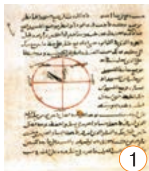
Qiblani aniqlash chizmasi. VIII asr. Muhammad ibn Muso Xorazmiy
