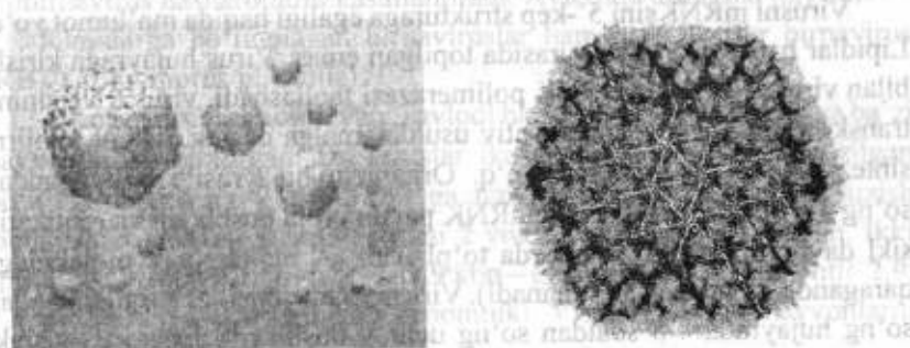
37-rasm. Bursa yuqumli kasalligi virusi va birnaviruslar strukturasi. (85)
