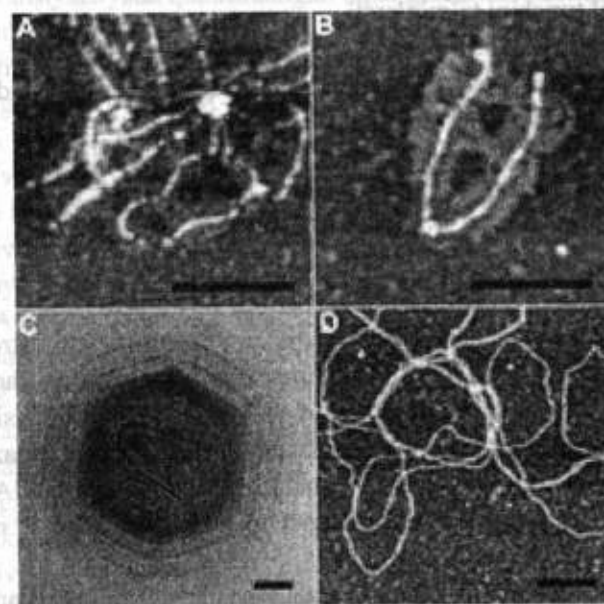
66-rasm. Mimiviruslarning oqsil iplari. A, B — ipning tashqi yuzasi, (atomno-silovaya mikroskopiya); S — lizotsim va bromelayn bilan ishlov berilgan mimivirus (krioElektron mikroskop); D — ichki oqsil iplar (atomno-silovaya mikroskopiya) (121)
