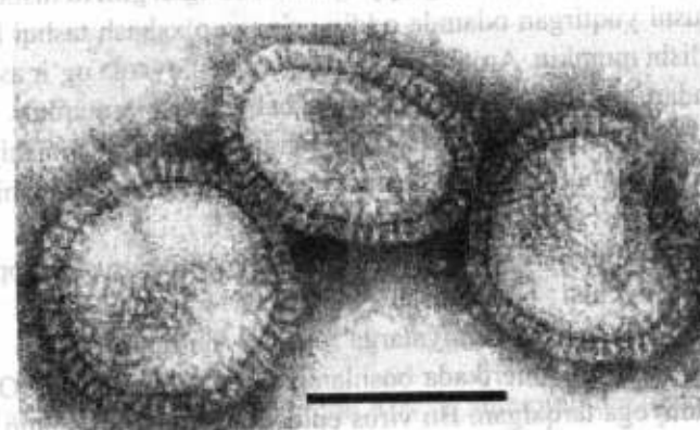
47-rasm. A gripp virusi (elektronmikrofotografiya) (100)
