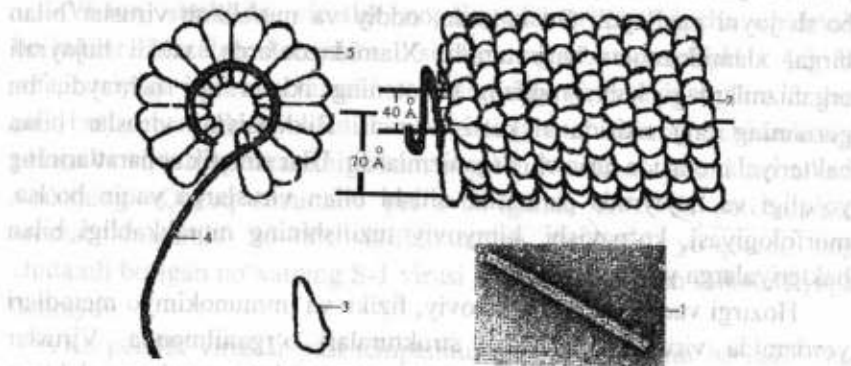
9-rasm. Tamaki mozaikasi virusining tuzilishi: 1-virion; 2-virionning ultrastrukturasi; 3-oqsil subbirliqi; 4-RNK; 5-virionning bir qavatida joylashgan subbirliklar (1).
