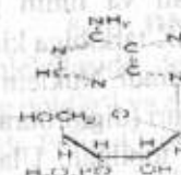
Adenozin-3-fosfat
