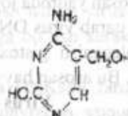
5-oksimitilsitozin
