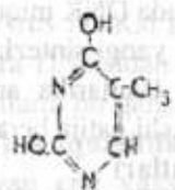
Timin (5-metiluratsil)
