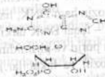
Guanozin-3-fosfat
