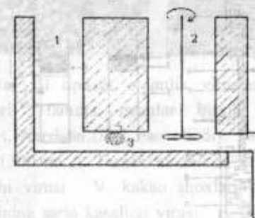
Ilova, 11-rasm. «Chiziqli» saxaroza yoki sulfat seziy konsentratsiyalari gradientlarini tayyorlashda ishlatiladigan qurilma: 1-rezervuar, 2-aralashtirgich, 3-jo'mrak, 4-ajratadigan truba.
