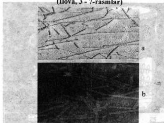
Ilova, 3-rasm. Arpa shtrixli mozaikasi virusining elektron mikrofotografiyasi: A – palladiy bilan changlatilgan (kattalashtirilishi 60 000 x); B – fosfor - volfram kislotali bilan kontrastirlangan (kattalashtirilishi 150 000 x)
