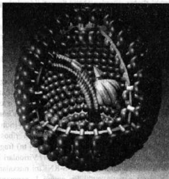
57-rasm. Bornavirusnig kesmasi (molekulyar strukturasi) (109)
