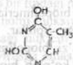
Timin (5-metiluratsil)
