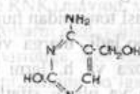
5-oksimetiltstozin
