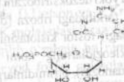
Sitodin-5-fosfat
