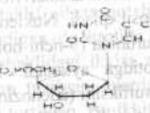
Timidin-5-fosfat
