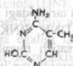
5-metiltstozin
