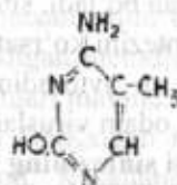
5-metilsitozin
