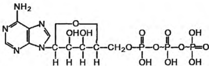
AMF (adenozin-5-monofosfat)
