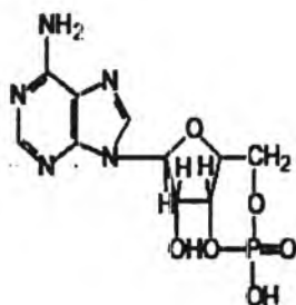
Siklik-3'-5'-adenozinmonofosfat (s-3',5'-AMF)
