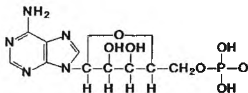
AMF (adenozin-5-monofosfat)
