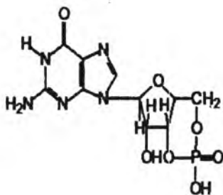
Siklik-3'-5'-guanozinmonofosfat (s-3',5'-GMF)
