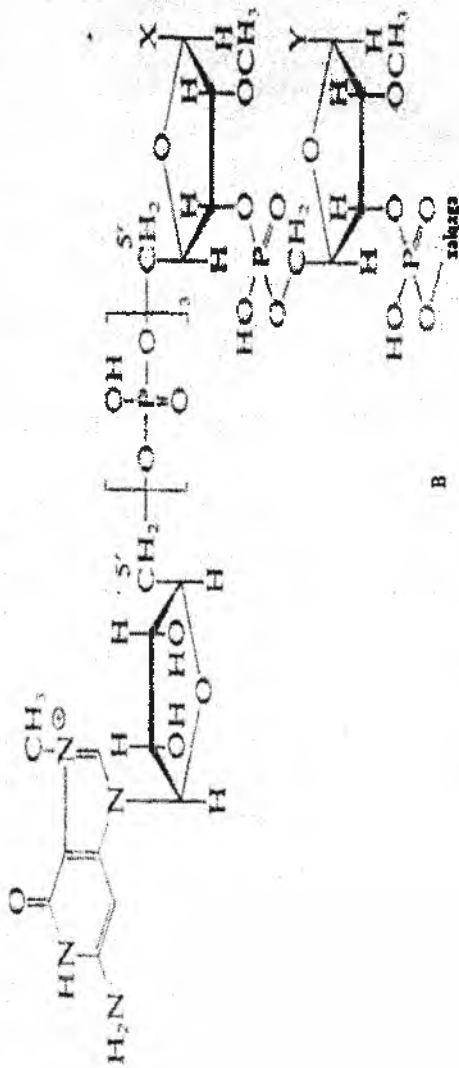
21-rasm. Eukariot i-RNK umumlashgan strukturasi. A-rasmda NTB-notranslyatsiya bo'limi; AUG-qismi esa inistirlovchi kodon. B-rasmda i-RNK molekulasini bir bo'lagi.
