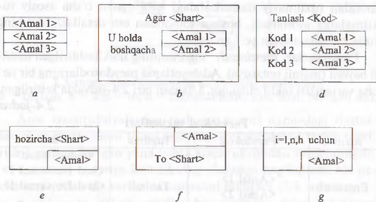
2.4-rasm. Asosiy konstruksiyalar uchun Flow-shakl shartli belgilari: a – ergashish; b – tarmoqlanish; d – tanlash; e – sikl-hozircha; f – sikl-to; g – hisobli sikl.
