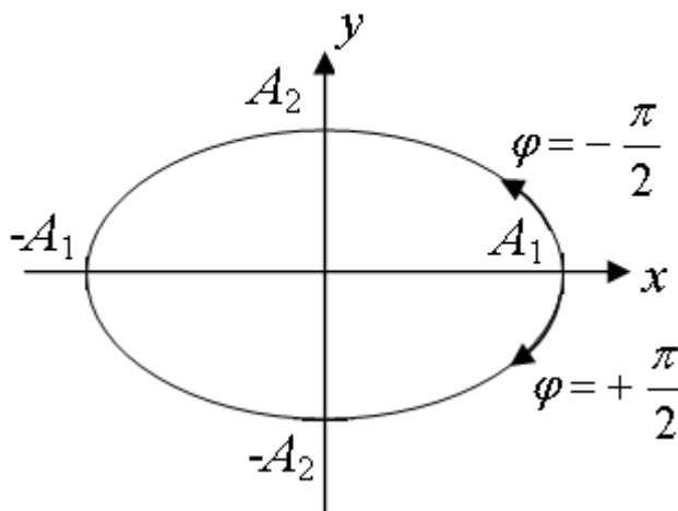
95 -расм. Фазалар фарқи \pm\frac{\pi}{2} га тенг бўлган тебранишлар қўшилишидаги натижавий тебраниш
