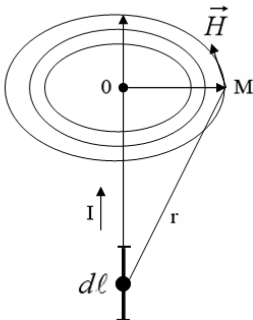
62 - расм. Тоқли ўтказгич магнит майдон кучланганлигининг йўналиши
