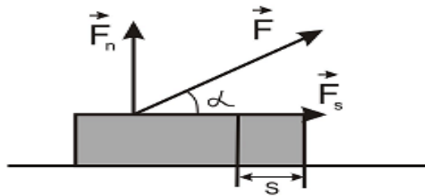
13 - расм. F куч таъсирида тўғри чизикли ҳаракат қилаётган жисмнинг кўчиши
