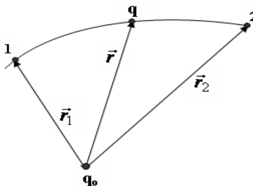
28 - расм. Қўзғалмас нуқтавий q_0 заряд майдонида q синовчи заряднинг ҳаракат траекторияси
