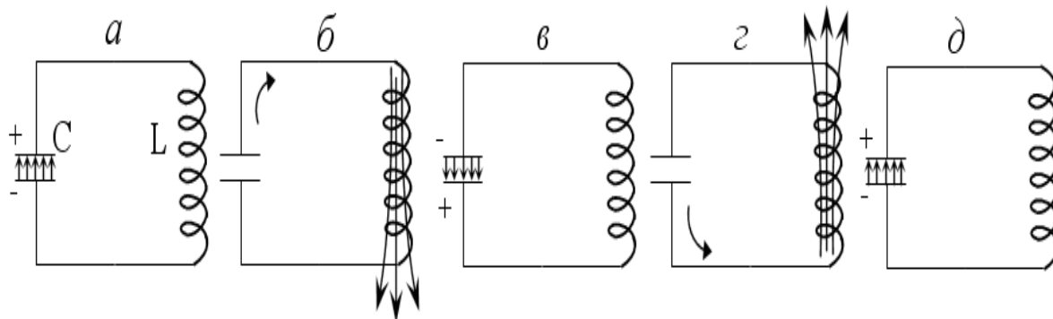
89 - расм. Ёпиқ электр занжирда электромагнит тебранишлар
