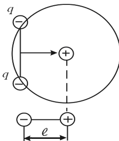
32 - расм. Қутбли молекула диполи
