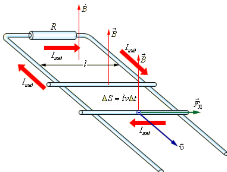
57 - расм. Токи цилиндри ўтказгичга магнит майдони таъсири
