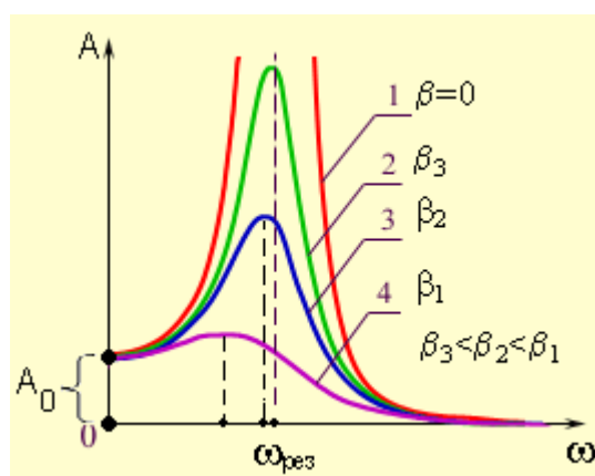
102 - расм. Мажбурий тебранишлар амплитудаларининг резонанс чизиклари
