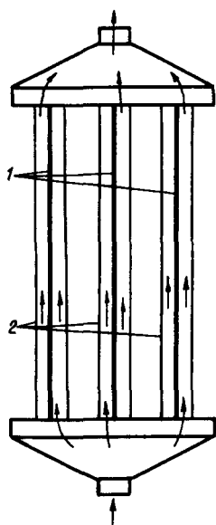
62-р а с м. Электрофильтр схемаси:
