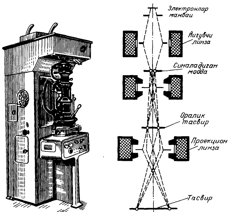
11-р а с м . Электрон микроскоп схемаси
