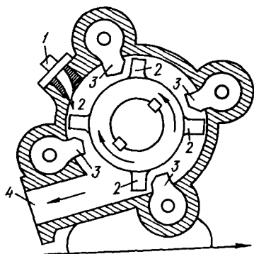
1-р а с м . Коллоид тегирмон.
