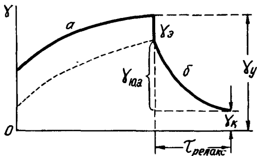
47-р а с м . Полимер парчасининг ўзгармас юк таъсирида чўзилиши
