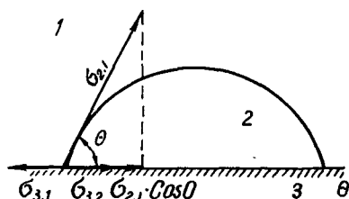
14-расм. Чет бурчак билан \sigma_{3,1} , \sigma_{2,3} ва \sigma_{2,1} орасидаги боғланиш 1 — ҳаво, 2 — суюклик, 3 — қаттиқ жисм
