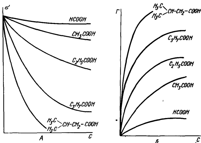
24-расм А — сувга турли кислоталар қўшилганда сув сирт таранглигининг кислота таркибига қараб камайиши В — сувга турли кислоталар қўшилганида кислота концентрацияси ортиши билан адсорбциянинг ўзгариши
