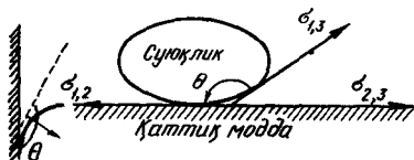
13-расм. Каттик жисмни хўлламайдиган суюқлик.
