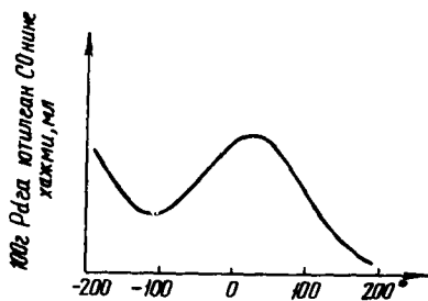
28-расм. Углерод (II)-оксиднинг палладийга адсорбиланиш диаграммаси.
