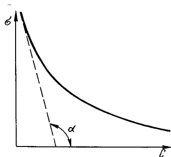
29-расм Сирт-актив модданинг ҳажмий концентрацияси билан унинг сирт таранглик ора-сидagi боғланиш
