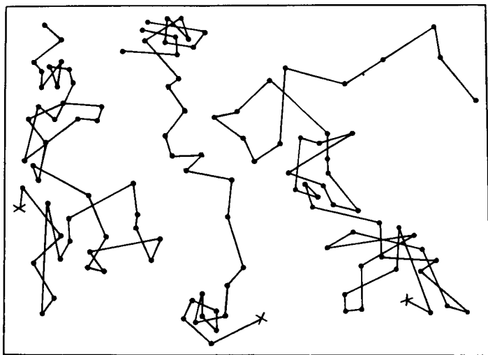
7-р а с м Мاستика суспензияси зарраларининг Броун ҳаракати проекцияси.
