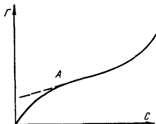
19-р а с м . Полимолекуляр адсорбцияни характерловчи изотерма чизиги
