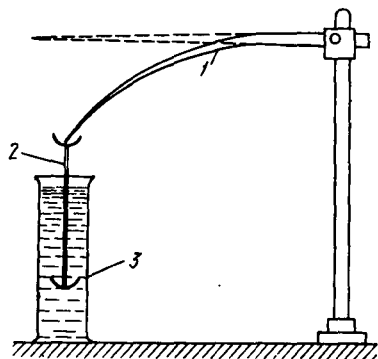
8-расм. Фигуровский тарозис: 1 — кварцдан ясалган шайн, 2 — шиша ил. 3 — тарози паллачаси
