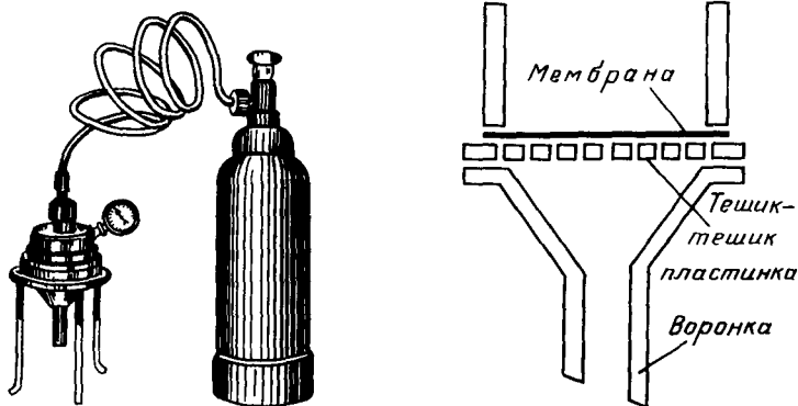
5-расм Ультрафилтр.
