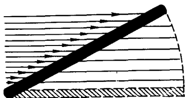
49-расм. Чўзикрок заррача суюкликнинг оқишига кўндаланг жойлашганида суюклик ҳаракатига ҳалал беради
