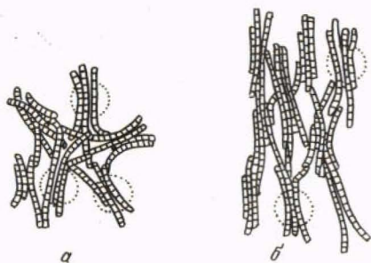
54-расм. Эластик ивик:
