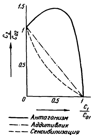
45-расм. Електролитлар аралашмаси таъсири остида бўладиган коагуляция.
