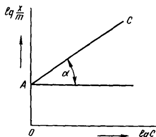
17-р а с м . Фрейндлих формуласининг логарифмик координаталарда чизилган графиги.
