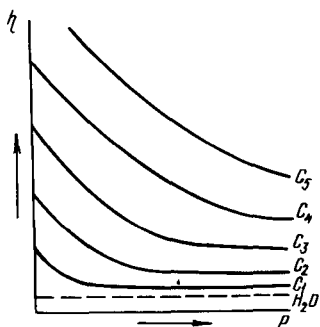
51-расм Турли концентрациядаги золь қовушоклигининг босимга қараб ўзгариш диаграммаси.
