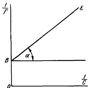
18-р а с м . Ленгмюр тенгламасининг графиги
