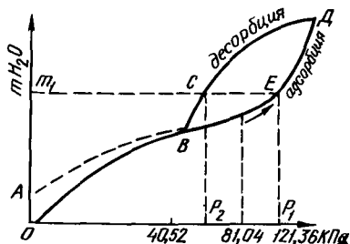
23-расм. Адсорбланиш гистерезиси (силикагелга сувнинг ютилиши).
