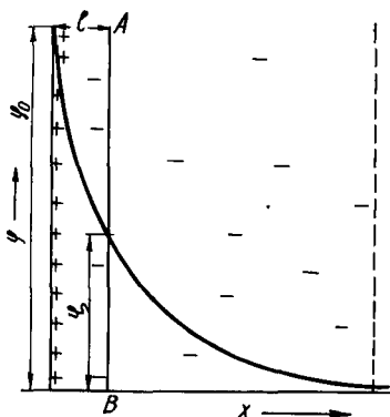
36-р а с м. Гуи-Чепменнинг кўш электр кават схемаси:
