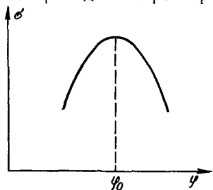
30-расм. Электрокапилляр диаграмма.
