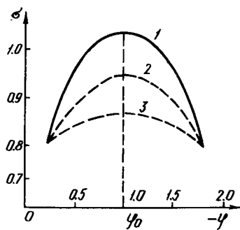
32-р а с м. Электрокапилляр эгри чизикнинг нононоген сирт-актив модда иштирокида ўзгариши:
