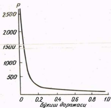
57-расм. Бўқиш босими билан бўқиш даражаси орасидаги боғланиш.
