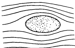
50-расм. Босим ортиганда заррачалар суюкликнинг оқиш йўлига параллел вазиятни эгаллайди
