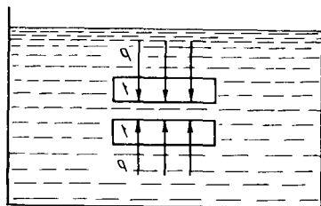
43-расм. Сольват қават билан бир-биридан ажралган икки пластинка орасидаги масофа кискартирилганда ерувчи босимнинг бунёдга келиши.
