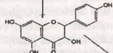
Digidrokversetin (digidroflavonol)
