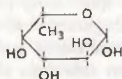
\alpha -L-fukoza
