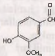
Vanilin
