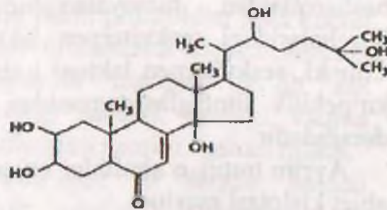
\alpha - Ekdizon
