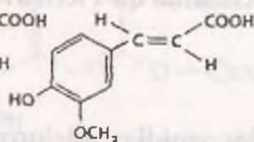
Ferul kislotasi
