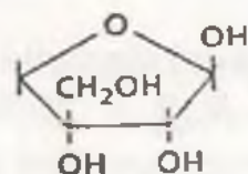
\alpha -D-apioza
