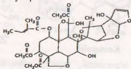
Azadiraxtin
