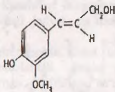
Koneferil
