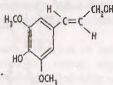
Sinon spirti
