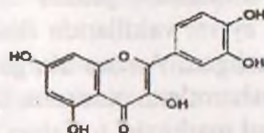
Kversetin (flavonol)
