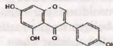
Genistein (izoflavonoid)
