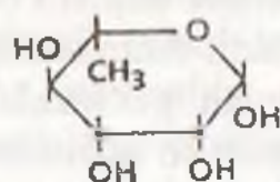
\alpha -L-ramnoza
