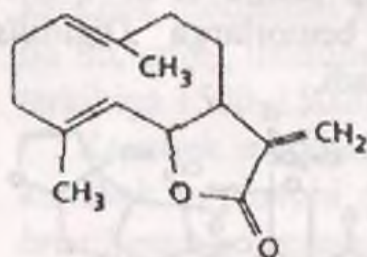
Kostunolid
