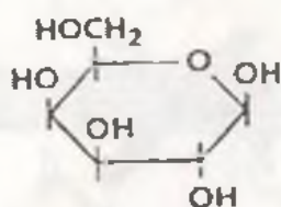
\beta -D-galaktoza
