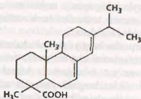
Abiet kislotasi
