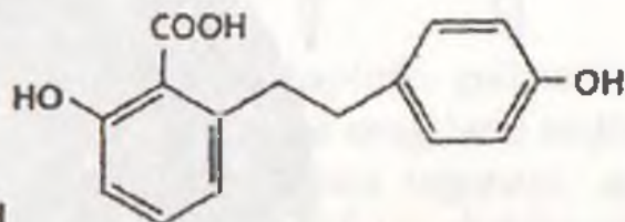
Lunular kislota
