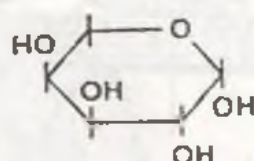
\alpha -L-arabinoza
