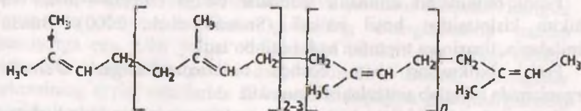
Kauchukning formulasi.
