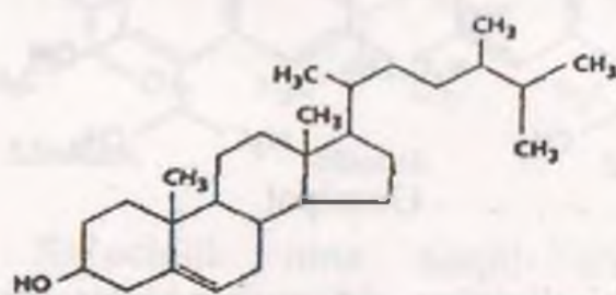
Sitosterol
