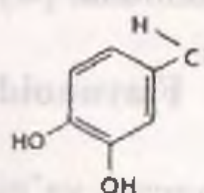
Kofe kislotasi
