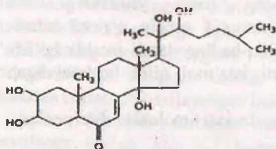
Ponasteron A
