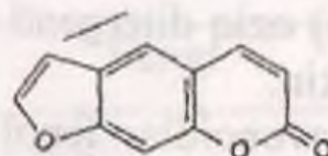
Psoralen
