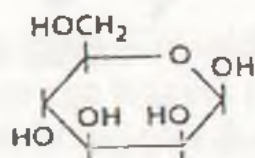
\beta -D-mannoza
