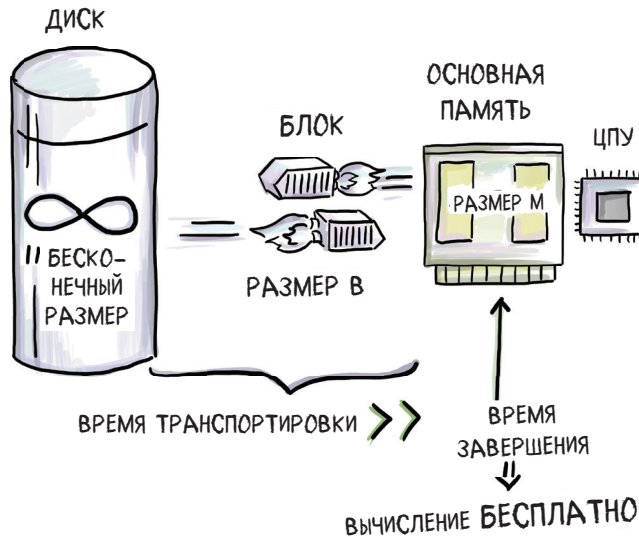
Рисунок 9.1 Модель внешней памяти. Эта модель подходит для анализа приложений по обработке массивных данных, в которых затраты на вычисления в оперативной памяти поглощаются гораздо большими затратами на передачу данных с диска в основную память и обратно. Вычисления не совсем бесплатны, но они настолько дешевле, чем стоимость передачи данных, что во многих приложениях они фактически бесплатны
