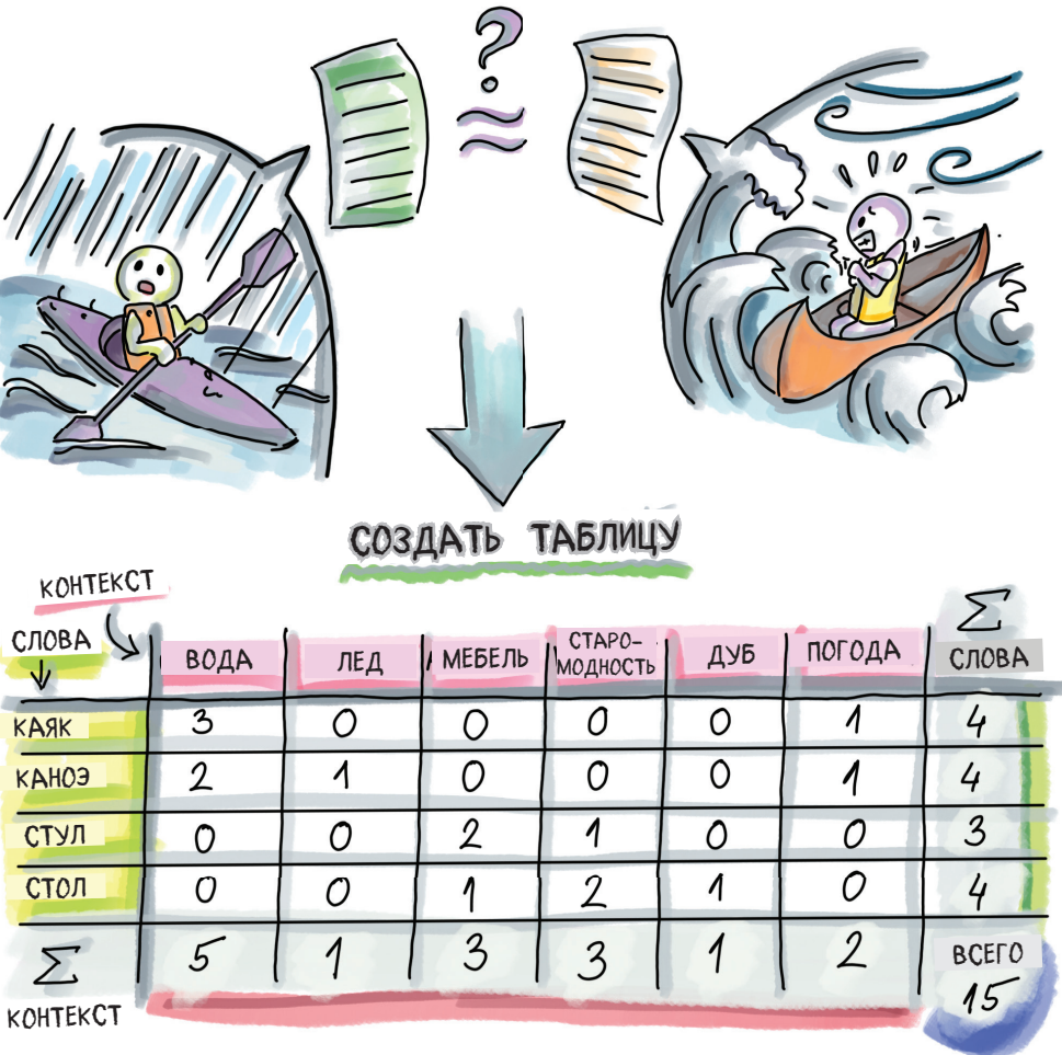
Рисунок 4.6 Создание матрицы M , в которой запись M[A][B] содержит число появлений слова A в контексте B , является одним из способов предобработки текстового массива для вычисления поточечной взаимной информации.
