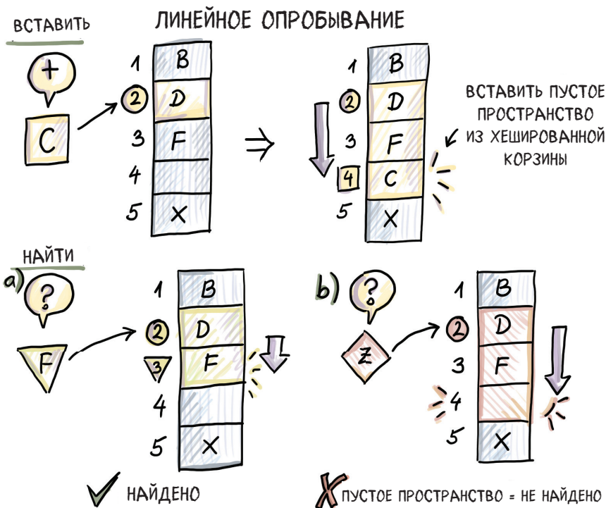
Рисунок 2.9 Пример вставки и поиска в линейном опробывании
