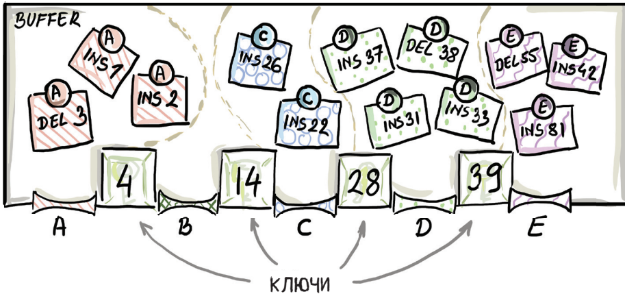
Рисунок 10.10 Узел B e -деревя имеет ключи и буферы.
