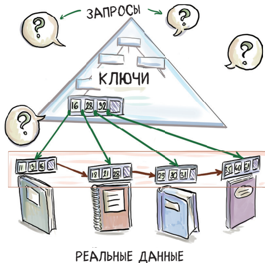
Рисунок 10.8 Организация В + -дерева. Внутренние узлы просты и содержат ключи, которые маршрутизируют запросы к листьям, в которых содержится более подробная информация о каждом ключе
