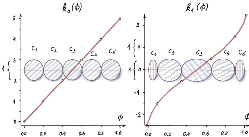
Рисунок 8.3 \mathcal{K}^{k_1} и \mathcal{K}^{k_0} различаются между k_1 и k_0 . k -размеры в обеих функциях отводят пять кластеров (оба t-дайджеста показаны в виде упорядоченного набора полностью слившихся кластеров; никакие два поочередных кластера нельзя объединить без нарушения весовой границы). Кластеры k -размера в обоих случаях равны 1; тем не менее сообщаемые кластерами подынтервалы различны, и для k_1 они переменны, при этом меньшие кластеры расположены по краям, а большие – в середине. Для k_1 они сообщают о подынтервалах одинаковой ширины, равной [0,1]
