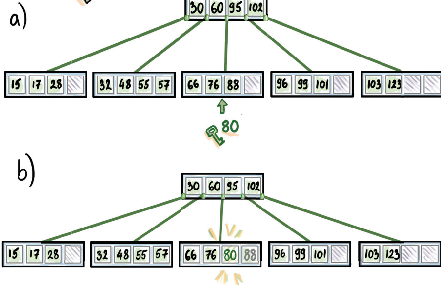
Рисунок 10.3 Вставка в В-дерево, когда указанный лист не заполнен
