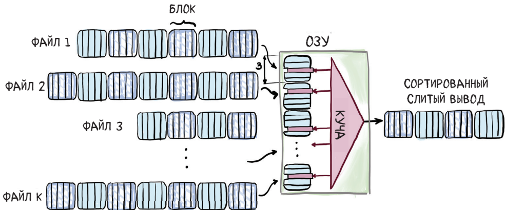
Рисунок 9.7 K -путное слияние сортированных файлов. Каждому файлу отведен один блок данных в основной памяти, и через этот блок каждый файл отправляет оставшиеся минимумы в кучу. Минимумы многократно извлекаются из кучи и отправляются в вывод. Эта схема работает независимо от общего накопленного размера файлов, при условии что K = O(M/B)
