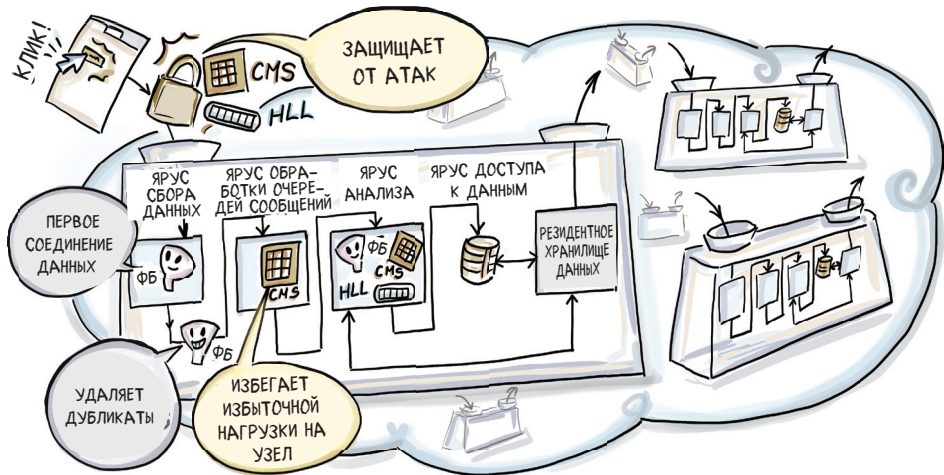
Рисунок 6.5 Архитектура облачных вычислений, обслуживающая разные клиентские конвейеры данных. Приложение мониторинга сетевого трафика, установленное для отслеживания обмена между производителями данных (или любых попыток обмена, исходящих из-за пределов облака), реализовано с помощью наброска count-min. Набросок count-min идентифицирует сетевые потоки, которые проявляют скорости, превышающие определенный заранее установленный порог, и действует соответствующим образом. Схожие задачи балансировки нагрузки между брокерами яруса обработки очередей сообщений решаются аналогичным образом применением еще одного наброска count-min в узле балансировки нагрузки на ярусе обработки очередей сообщений. Обратите внимание, что оба этих наброска count-min оперируют на заголовках пакетов/сообщений и что полезная нагрузка пакетов/сообщений, а именно данные о производимых пользователем кликах, не анализируется до тех пор, пока они не достигнут яруса анализа. Там вычисляются другие фильтры Блума, массивы HyperLogLog, процедуры взятия выборок или иные резюме/сводки
