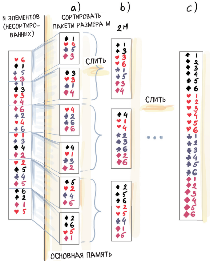
Рисунок 11.3 Двупутная сортировка слиянием, адаптированная к внешней памяти.
