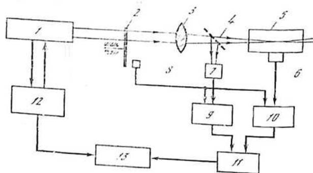
6.12. rasm. Lazerli atom-akustik spektrometrning umumiy sxemasi: 1-bo'yoq lazeri, 2-modulyator, 3-linza, 4- yarimtinik plastinka, 5- OA detektor, 6- akustik datchik, 7- fotopriyomnik, 8- generator, 9-10-kuchaytirgichlar, 11- nisbatni o'lchovchi asbob, 12-programmashtirish bloki, 13- qayd qilish sistemi.
