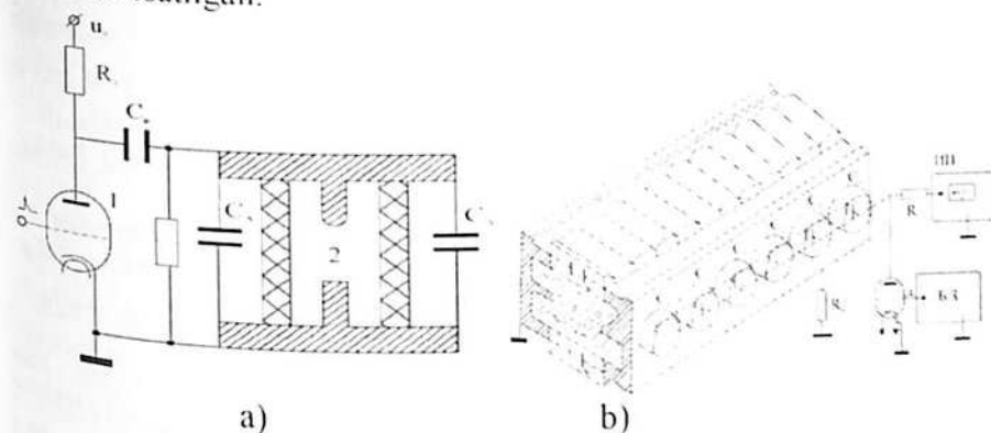
3.24-rasm. Azot lazerining ishlash va tuzilish sxemasi. a)-tiratron lampasi, b)-lazer kamerasi, U, yuqori kuchlanishli elektr manbai, S_n - yig'uvchi kondensator, S_1 - keskinlashtiruvchi kondensator
