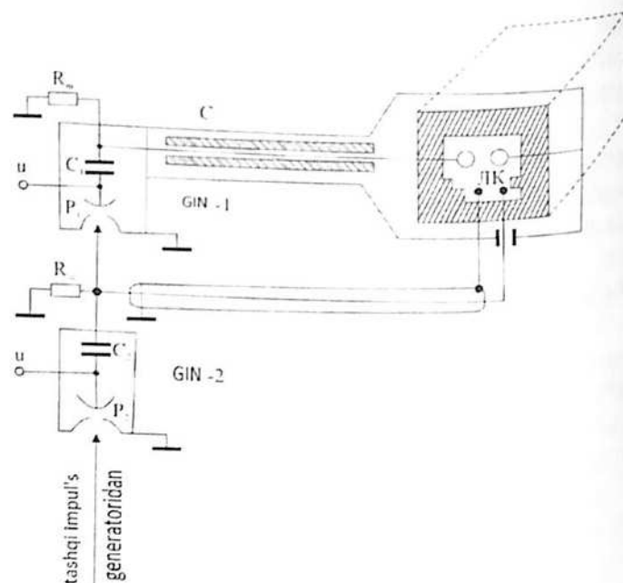
3.37- rasm. Eksimer lazerining elektr sxemasi. U-yuqori kuchlanish elektr manbai, R_{sh} - shuntlangan qarshilik, R_1 - razryadnik, C_1, C_2 - elektr energiyasini yig'uvchi kondensator, C_L - kondensator, LK - lazer kamerasi, GIN-1, GIN-2 impulsli kuchlanish beradigan generatorlar.
