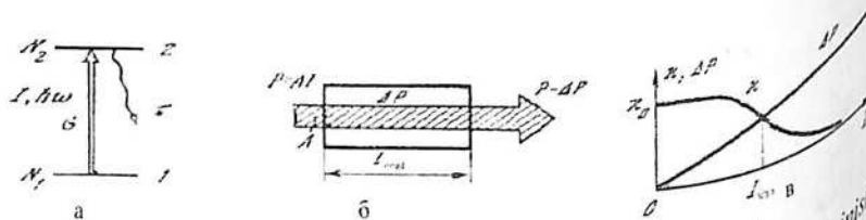
4.3 rasm. Metodning sezgirlik darajasini baholash: a-kvant o'tishlar sxemasi, b-o'lchash geometriyasi, v- yutilish va to'yinish ko'effitsientlarining yorug'lik intensivligiga bog'lanishi.
