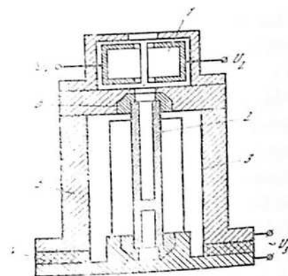
6.4 rasm. Elektrotermik atomizatorning konstruktiv sxemasi: 1-ion himoyasi, 2-grafit tigel, 3- ekran, 4-izolyator, 5-atomizator korpusi, 6-grafit elektrodlar.
