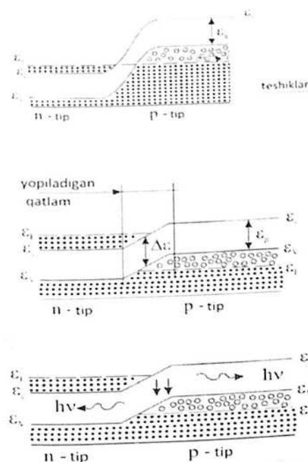
3.33-rasm. Kuchli legirlangan p - n -o'tishda yarim o'tkazgichlarning energetik zonalarini va kvant nurlanish sxemasi. a) elektr maydoni ta'siri bulmaganda zonalarining siljishi kuzatilmaydi. b) elektr maydoni ta'sirida zonalarining p -tip tomonga siljishi. v) Rekombinatsiya paytida yopiladigan qatlamdan kvant nurlanishi.
