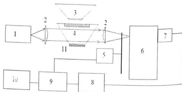
6.9 rasm. Atom absorbsion analizda qo'llaniladigan spektrometr sxemasi: 1-lazer, 2-yig'uvchi va sochuvchi linzalar, 3-bo'sh kyuveta, 4-gaz qamalgan kyuveta, 5-modulyator, 6-monoxromator, 7-fotoelektron ko'paytirgich, kuchaytirgich, 9-sinxron detektor, 10-qayd qiluvchi samopisssets, 11-atom bug'larini hosil qiluvchi atomizator.
