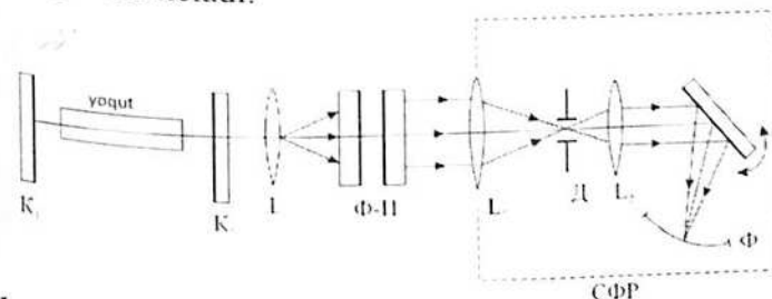
3.11-rasm. Yoqut lazeri generatsiyasining spektrini o'rganish sxemasi.
