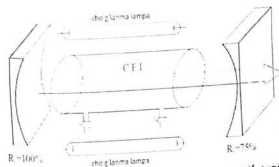
3.35-rasm. Kimyaviy yod lazerining sxematik tuzilishi.
