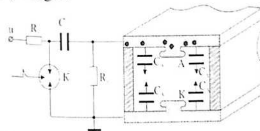
3.21-rasm. CO_2 lazerning sxematik tuzilishi. Shu tuzilishi va impuls rejimda ishlashni ta'minlaydi.
