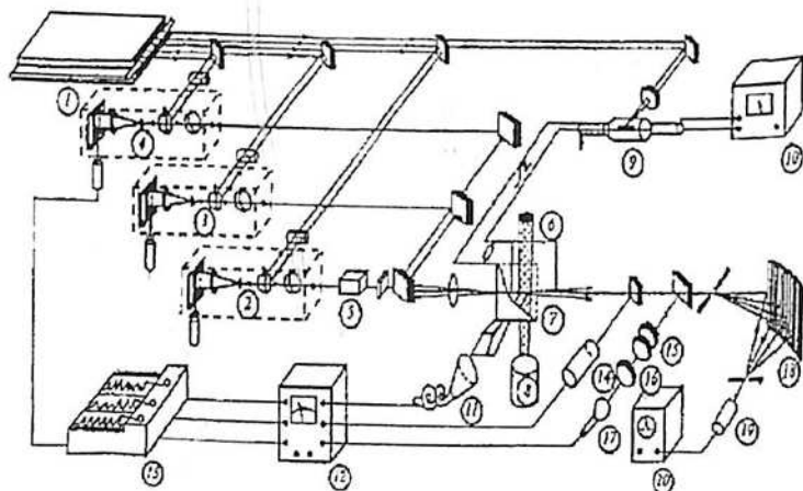
6.3 rasm Lazer fotoionizatsion spektrometrining umumiy sxemasi. 1- azot lazeri, 2-4 bo'yoq lazerlari, 5- nohiziqli Kristal, 6- atom dastasi, 7- elektrodlar, 8- atomizator, 9- impulsli kuchlanish generatori, 10- yuqori kuchlanishli tok manbasi, 11- fotoelektron ko'paytirgich, 12- strobintegrator, 13- o'zi yozuvchi qurilma, 14- LPS tipli lampa, 15- Fabri- Pero interferometri, 16- linza, 17- fotoelektron ko'paytirgich, 18- monoxromator, 19- fotodiod, 20- ossilograf
