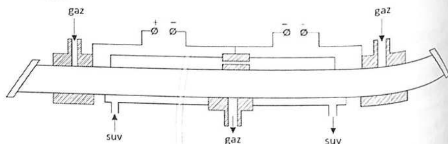
3.22-rasm. CO 2 lazerining uzluksiz rejimda ishlash sxemasi.
