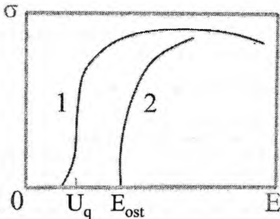
5.8-rasm. Ekzotermik va endotermik yadro reaksiyalarining uygʻonish funksiyalari.
