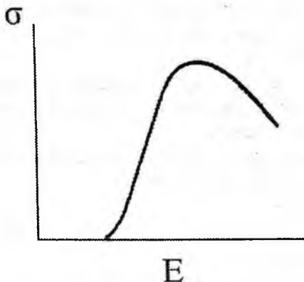
5.7-rasm. Reaksiya kesimining zaryadlangan zarra energiyasiga bog'lanishi.
