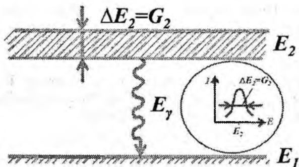
4.11-rasm. Uyg‘ongan holat sath va chiziqlining tabiiy kengliklari.
