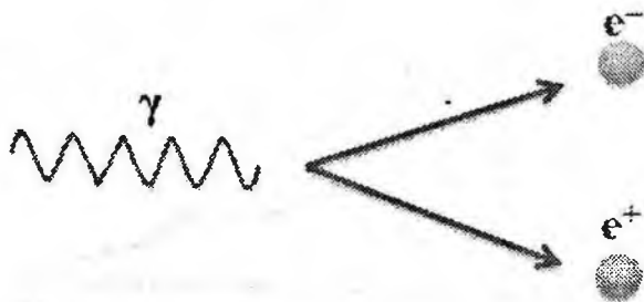
6.10-rasm. Elektron-pozitron jufti hosil bo'lish sxemasi.
