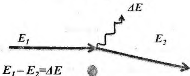
6.3-rasm. Yadro maydonida elektron tormozlanishi.
