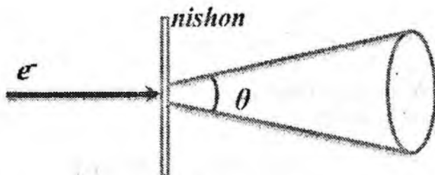
6.6-rasm. Tormozli nurlar burchak taqsimoti.
