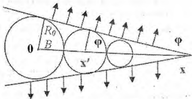
6.7-rasm. Vavilov-Cherenkov nurlanishi vujudga kelish sxemasi. 1-muhitda harakatlanayotgan zarra vujudga keltirgan nurlanish to'liqlarining fronti bo'lib, u zarra tezligi vektoriga \varphi burchak ostida yo'nalgan bo'ladi.
