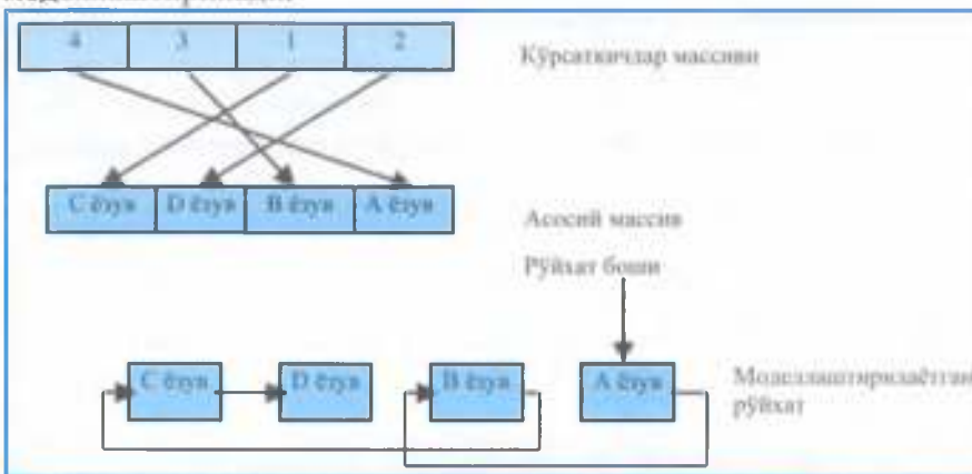
5.11-расм. Боғланган рўйхатни массив тузилмаси ёрдамида моделлаштириш
