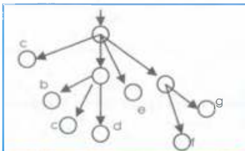
7.20-расм. Рўйхатли тузилмани граф кўринишида тасвирлаш этиши
