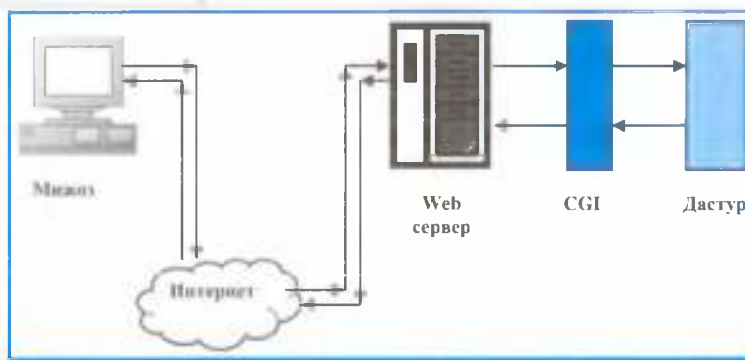
Рис. 4. CGI дастурлари маълумотлар оқимининг схемаси.
