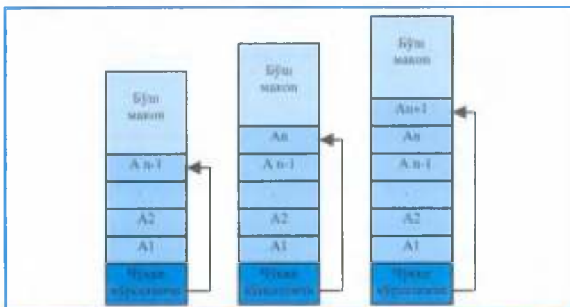
6.2-расм. Стекни кетма-кет тақдим этганда унинг ортинги ва камайини
