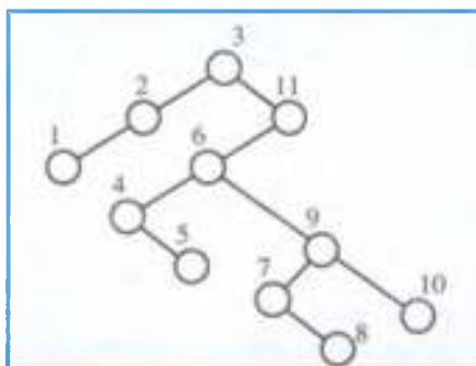
10.6-расм. Саралаш дарахтини тузиш
