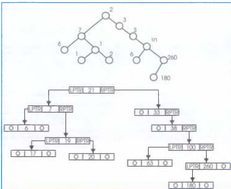
7.14-расм. Иккилик дарахт ва уш икки боғли рўйхат куринишида сақлаш тузилмаси
