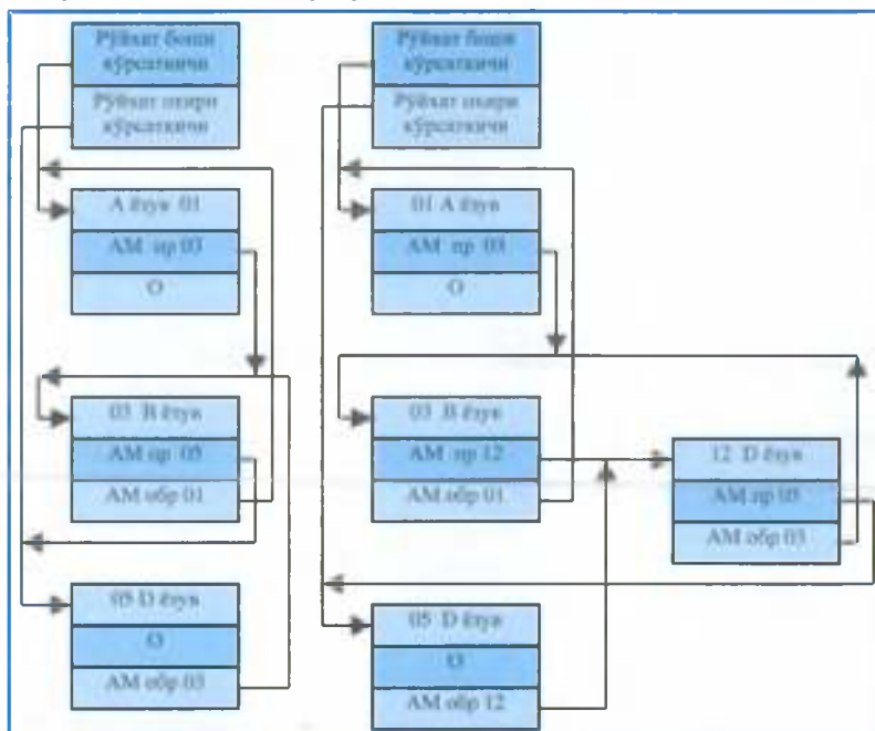
5.10-расм. Икки йўналишли рўйхат, а) дастлабки рўйхат, б) янги ёзув рўйхатига киритини.
