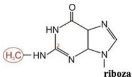
N 2 -Metilguanozin
