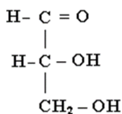
D-glitseraldegid
