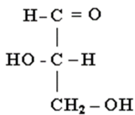
L-glitseraldegid
