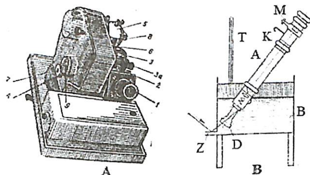
B- Pulfrich refraktometning ishchi qismini sxematik tuzilishi
