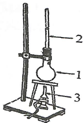
8-rasm. Oqsilni gidrolizlash uchun qurilma: 1-yumaloq tubli kolba, 2-havo sovitgichi, 3-gaz gorelka.
