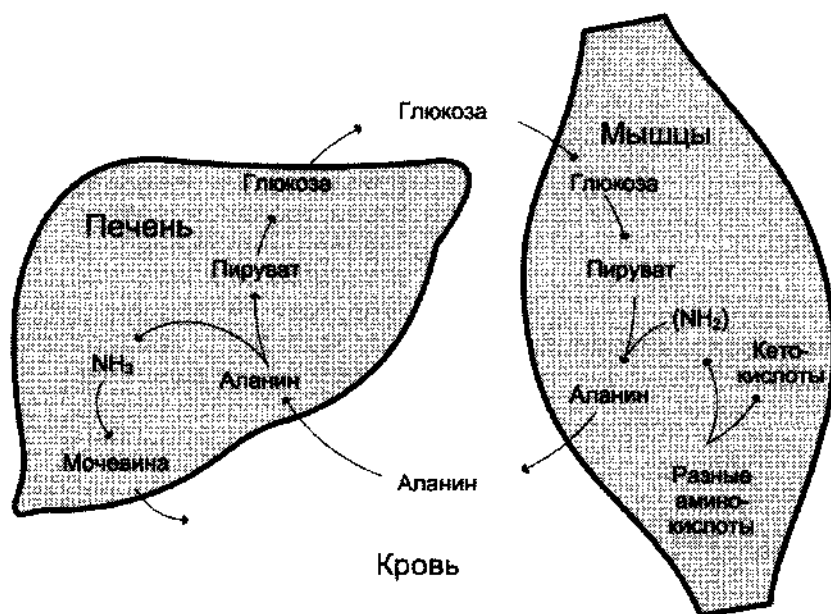
Рис. 9-13. Глюкозо-аланиновый цикл.
