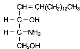
Сфингозин
