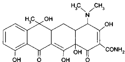
Тетрациклин
