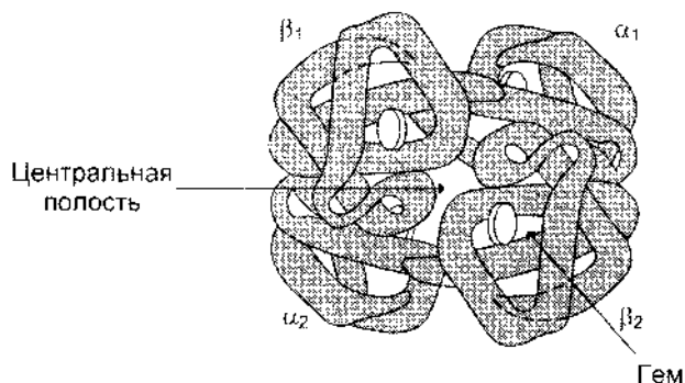
Рис. 1-32. Строение гемоглобина.
