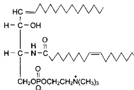
Сфингомиелин
