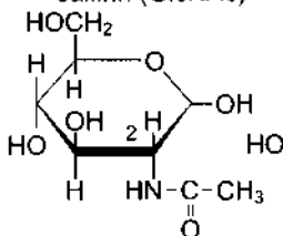
N-ацетил-D-глюкозамин (GlcNAc)
