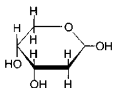
2-дезоксид-D-рибоза (dRib)
