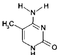
5-Метилцитозин
