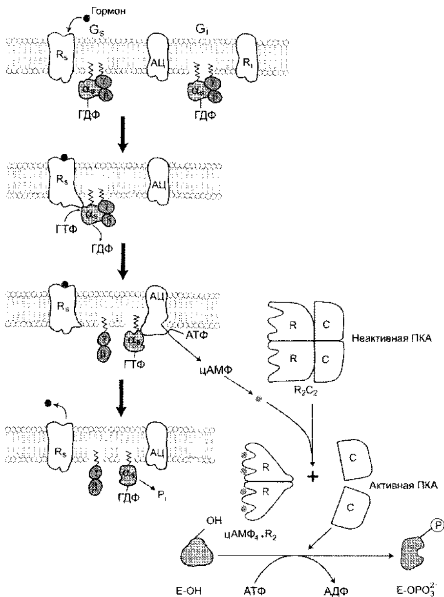
Рис. 5-41. Аденилатциклазная система.
