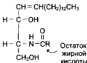
Церамид N-ацилсфингозин
