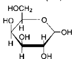
D-галактоза (Gal)
