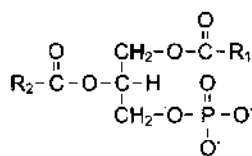
Фосфатидная кислота
