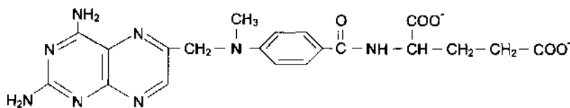
Метотрексат
