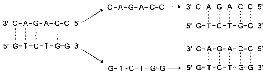
Рис. 4-14. Полуконсервативная репликация.
