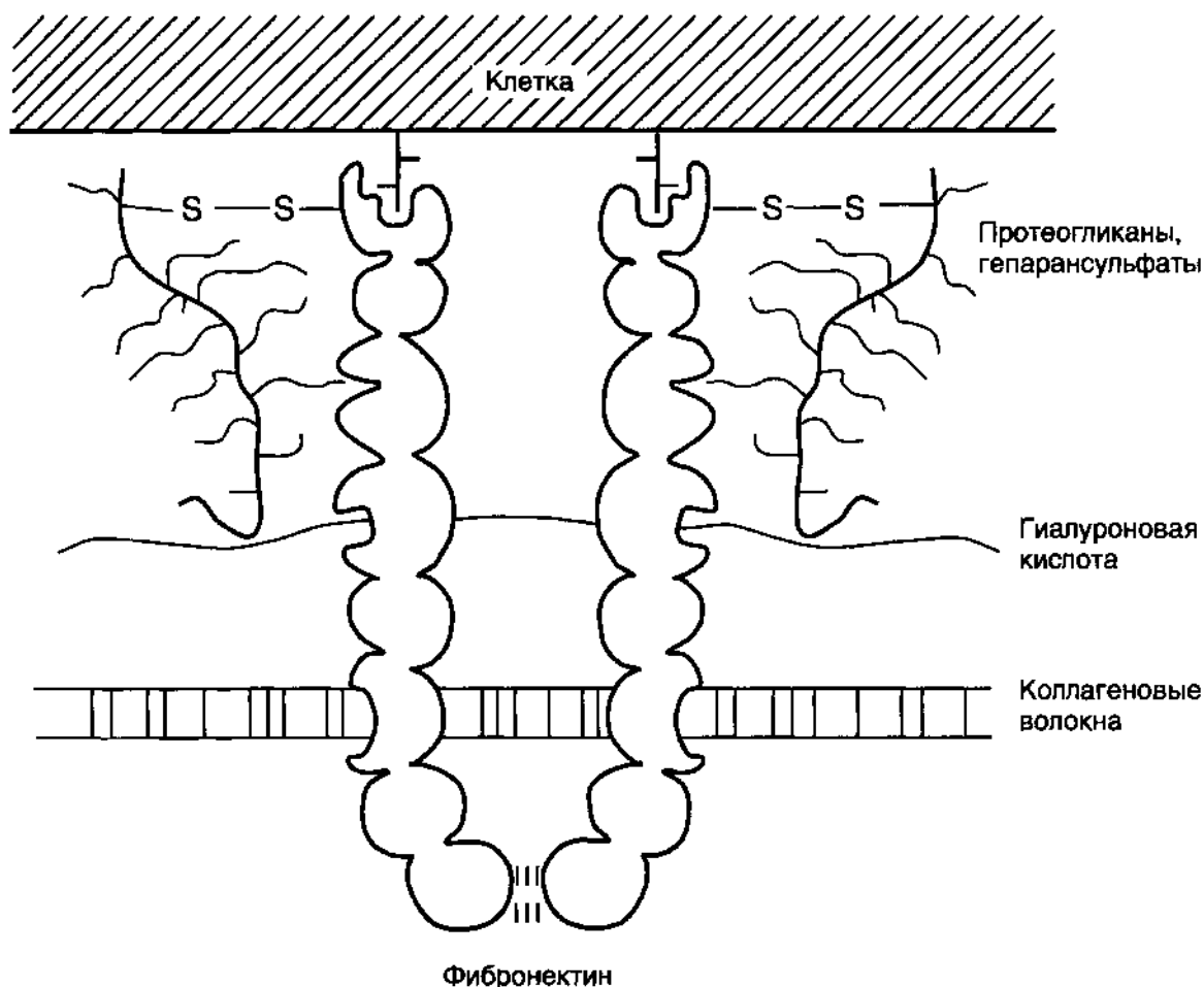
Рис. 15-19. Строение фибронектина.
