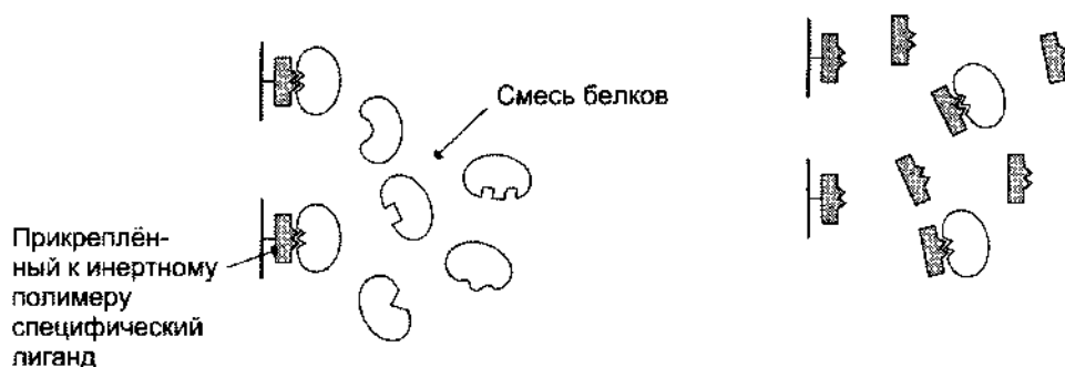
Рис. 1-58. Аффинная хроматография.
