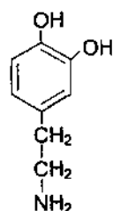
Дофамин
