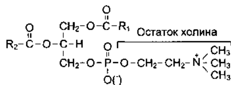
Фосфатидилхолин
