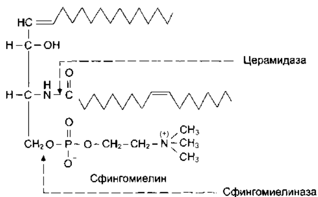
Рис. 8-63. Гидролиз сфингомиелина.
