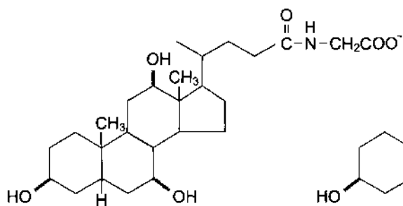
Гликохоле́вая кислота
