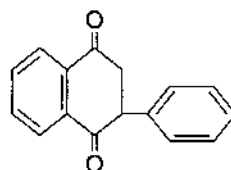
Флавоны
