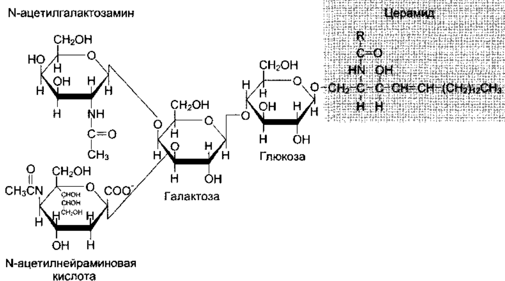
Рис. 8-8. Ганглиозид G_{m2} .
