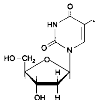
5-йод-2'-дезоксисуридин
