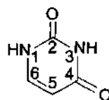
Псевдоурацил
