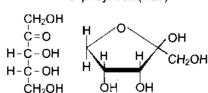
D-рибулоза (Rub)
