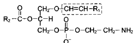
А. Фосфатидальэтаноламин
