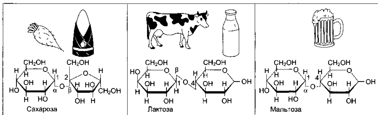
Рис. 7-8. Дисахариды пищи.
