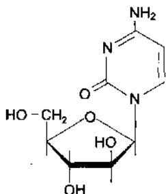
Цитозинарабинозид
