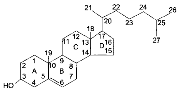
Холестерол
