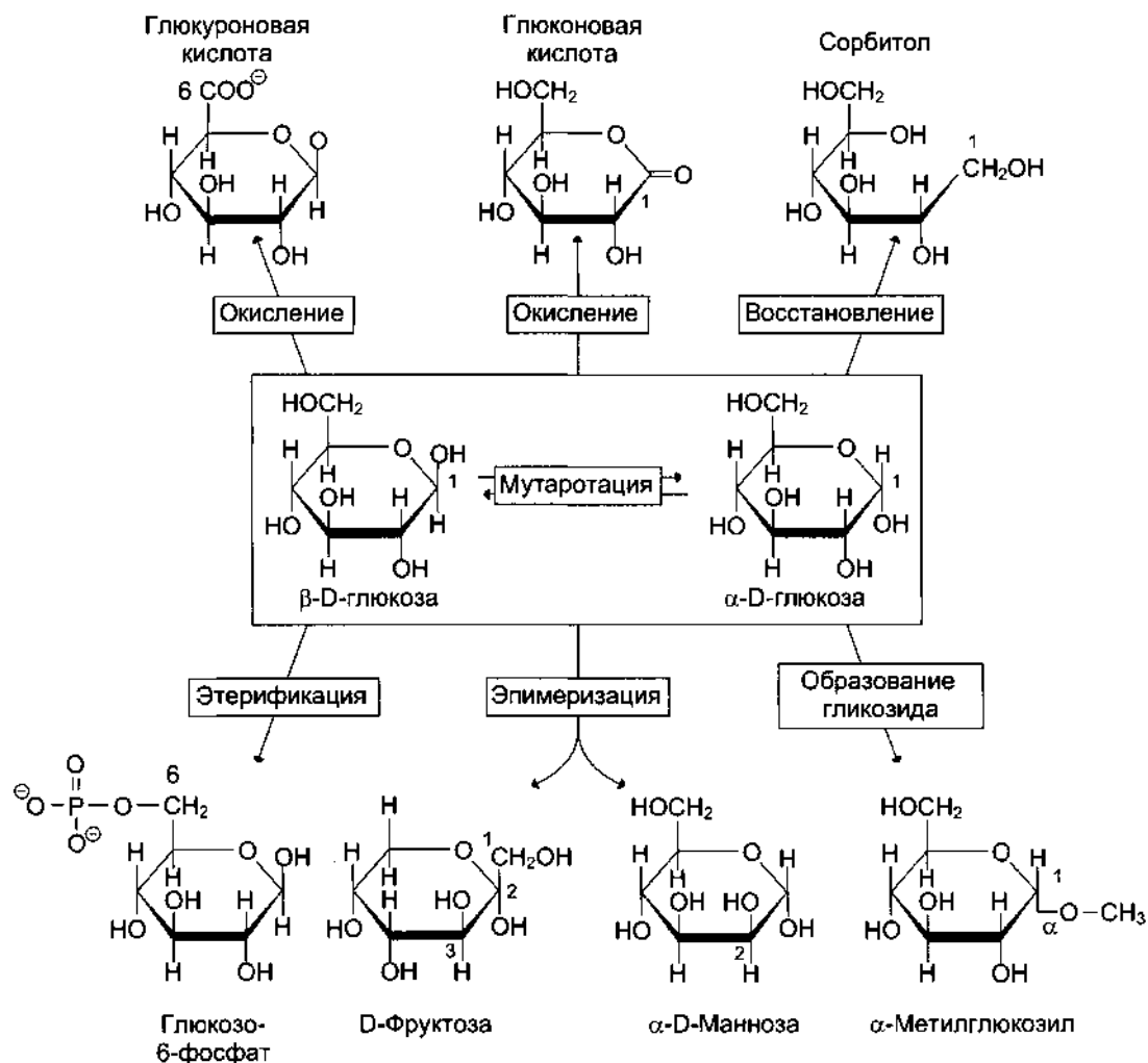
Рис. 7-5. Реакции моносахаридов.
