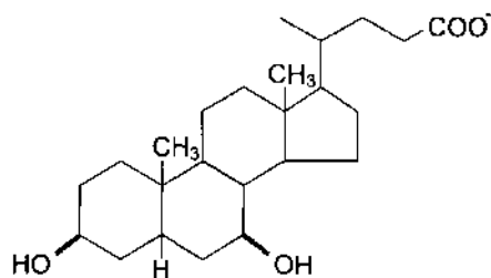
Хенодезоксиколе́вая кислота
