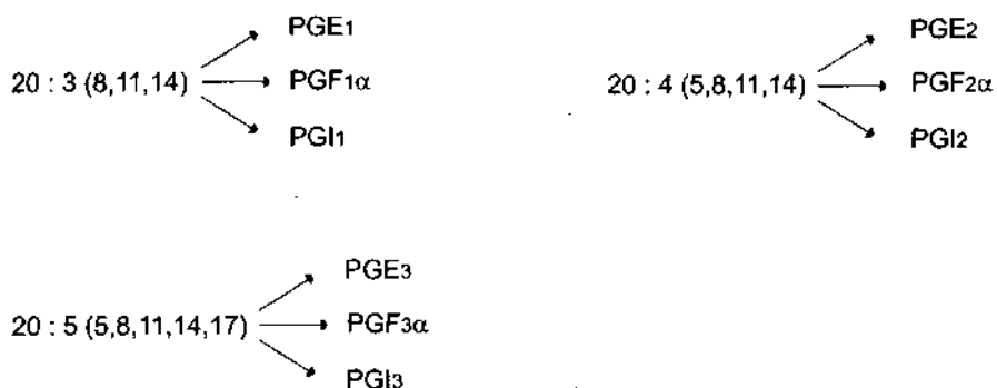
Рис. 8-45. Семейства простагландинов.
