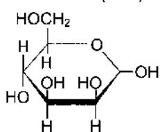
D-манноза (Man)
