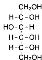
D-сорбит
