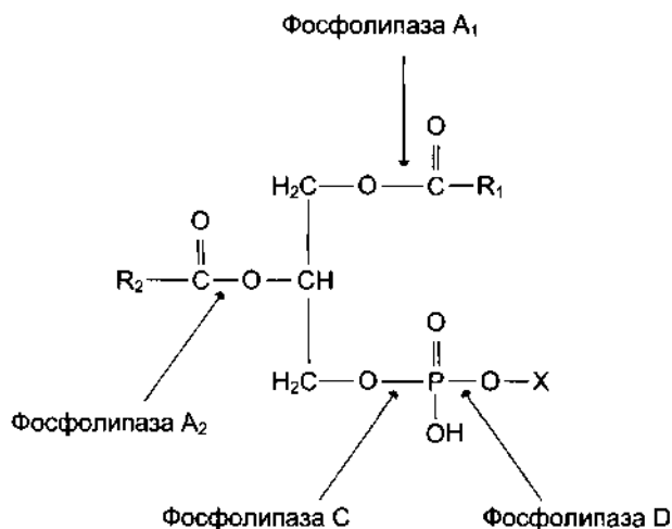
Рис. 5-37. Действие фосфолипаз.
