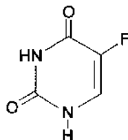
5-Фторурацил
