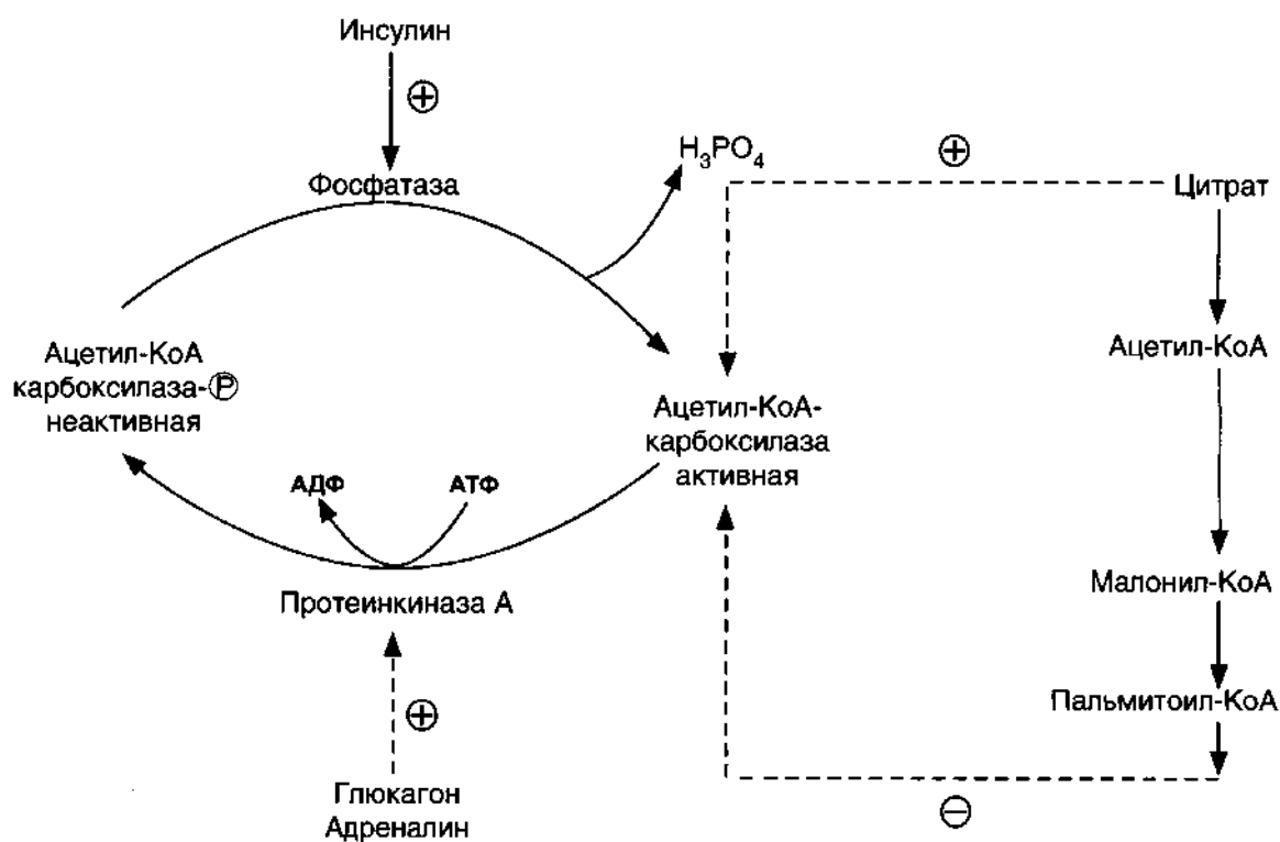
Рис. 8-41. Регуляция ацетил-КоА-карбоксилазы.
