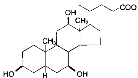
Холе́вая кислота
