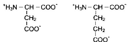
Аспартат
