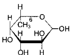
L-фруктоза (Fuc)
