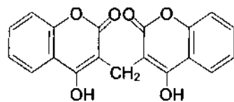
Дикумарол
