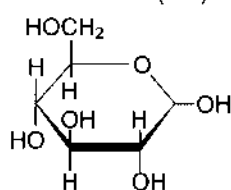
D-глюкоза (Glc)
