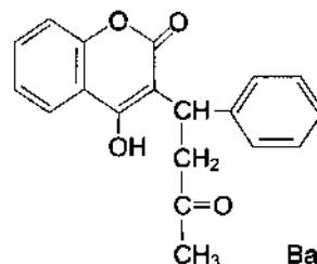
Варфарин
