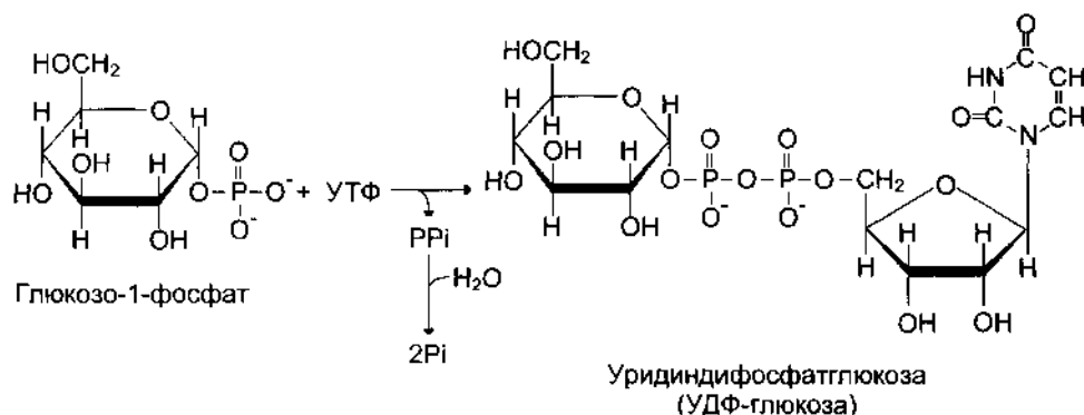
Рис. 7-24. Образование УДФ-глюкозы.
