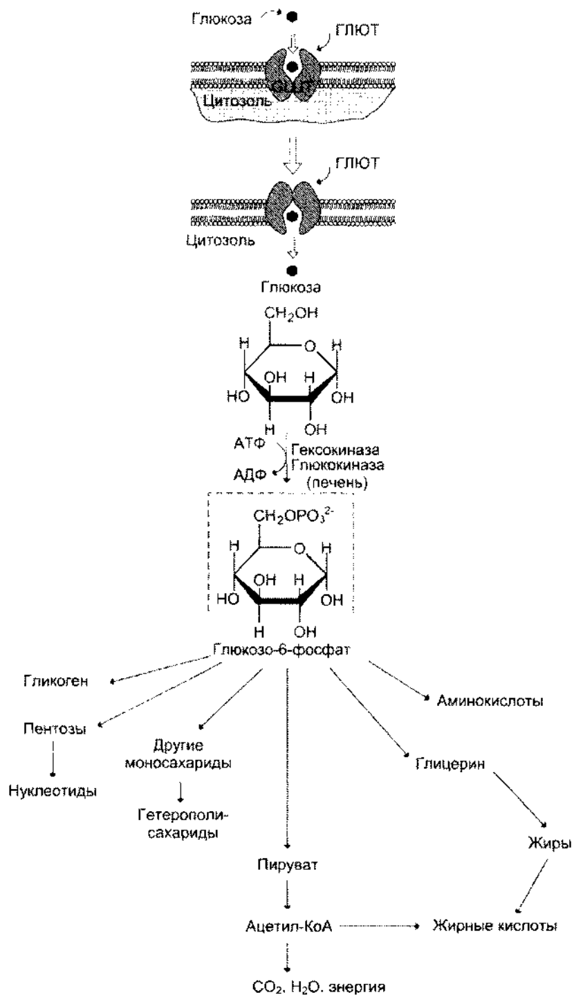
Рис. 7-20. Метаболизм глюкозо-6-фосфата.
