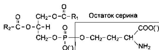
Фосфатидилсерин
