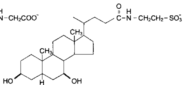
Таурохенодезоксиколе́вая кислота
