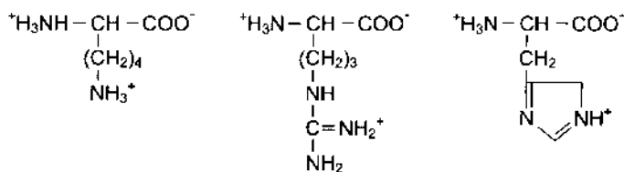
Лизин
