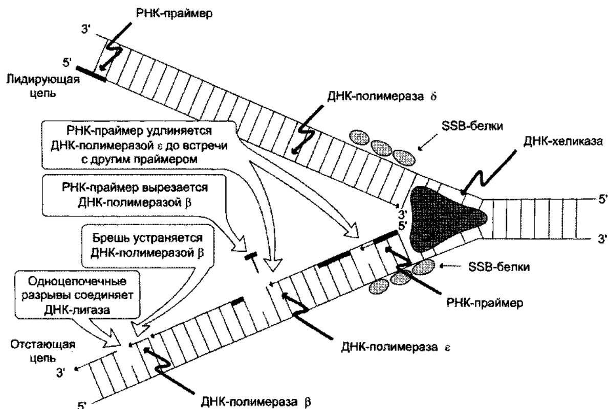
Рис. 4-16. Репликация.
