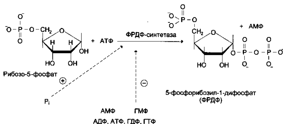
Рис. 10-2. Образование 5-фосфорибозил-1-дифосфата.
