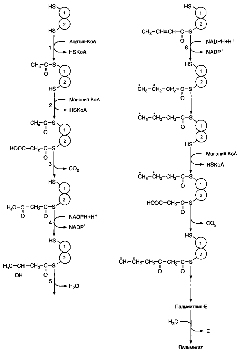
Рис. 8-38. Синтез пальмитиновой кислоты. Синтаза жирных кислот: в первом протомере SH-группа принадлежит цистеину, во втором — фосфопантетеину. После окончания первого цикла радикал бутирила переносится на SH-группу первого протомера. Затем повторяется та же последовательность реакций, что и в первом цикле. Пальмитоил-Е — остаток пальмитиновой кислоты, связанный с синтазой жирных кислот. В синтезированной жирной кислоте только 2 дистальных атома углерода, обозначенные *, происходят из ацетил-КоА, остальные — из малонил-КоА.
