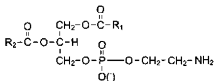
Фосфатидилэтаноламин
