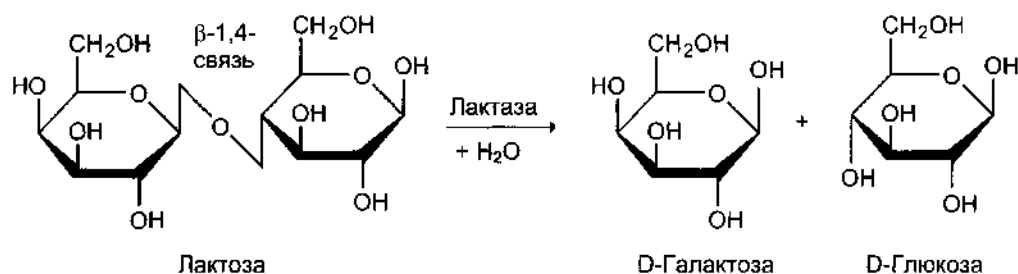
Рис. 7-15. Действие лактазы.
