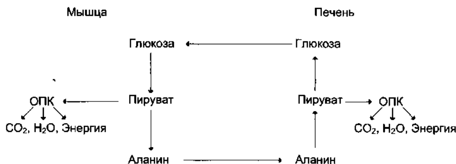
Рис. 7-52. Глюкозо-аланиновый цикл.
