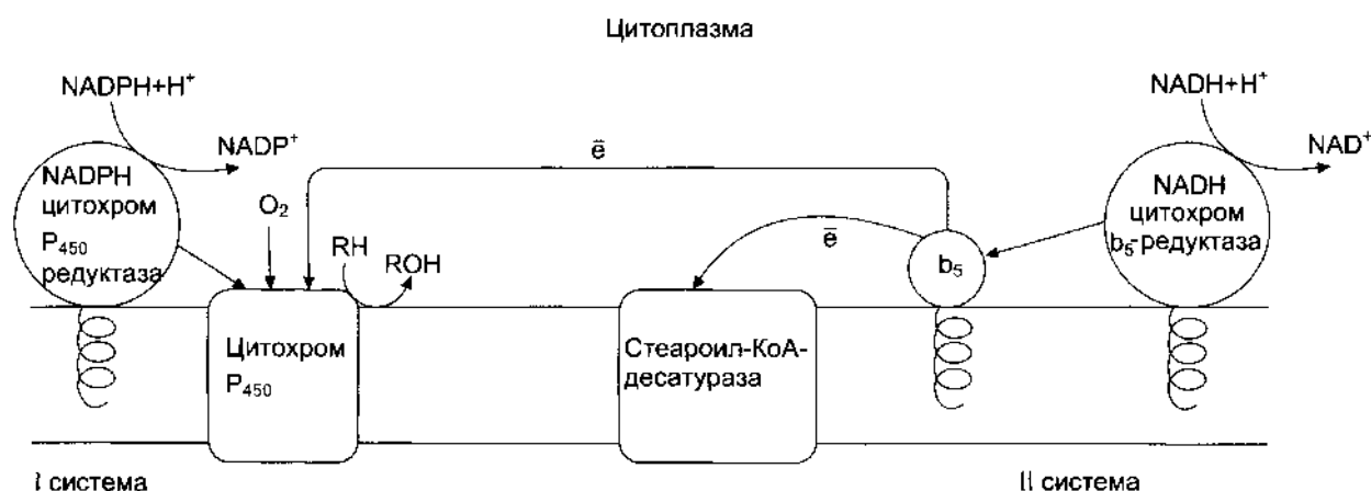
Рис. 12-2. Электронотранспортные цепи ЭР. RH — субстрат цитохрома \text{P}_{450} ; стрелками показаны реакции переноса электронов. В одной системе NADPH окисляется NADPH цитохром \text{P}_{450} -редуктазой, которая затем передаёт электроны на целое семейство цитохромов \text{P}_{450} . Вторая система включает в себя окисление NADH цитохром \text{b}_5 -редуктазой, электроны переходят на цитохром \text{b}_5 ; восстановленную форму цитохрома \text{b}_5 окисляет стеароил-КоА-десатураза, которая переносит электроны на \text{O}_2 .
