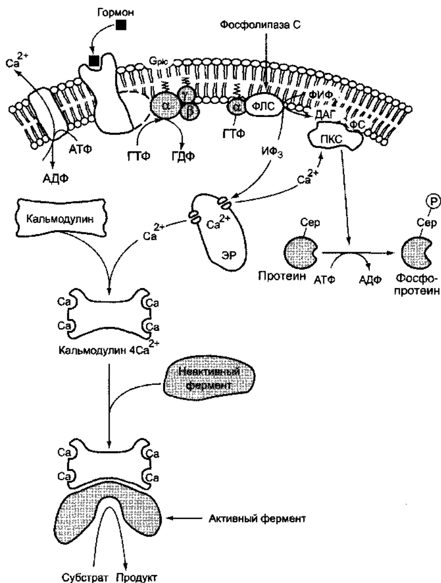
Рис. 5-42. Инозитолфосфатная система.
