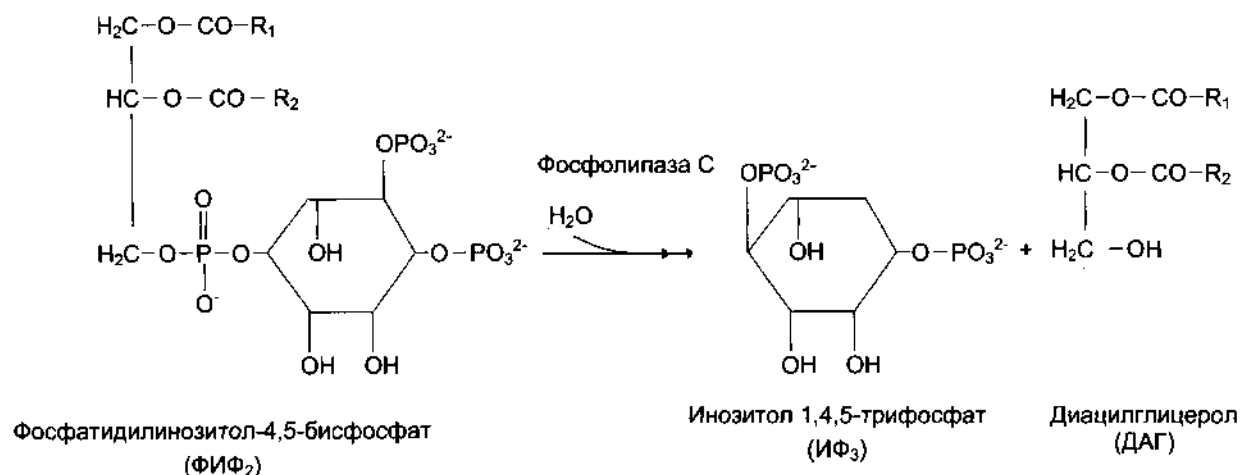
Рис. 5-8. Гидролиз фосфатидилинозитол-4,5-бисфосфата.
