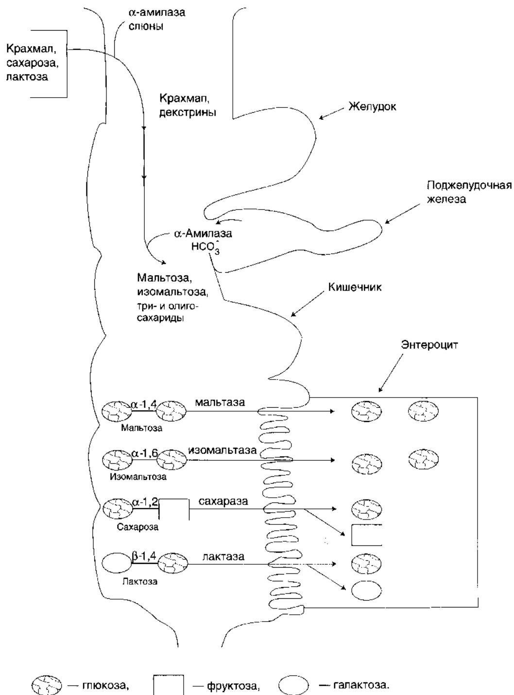
Рис. 7-17. Переваривание углеводов.
