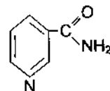
Никотинамид
