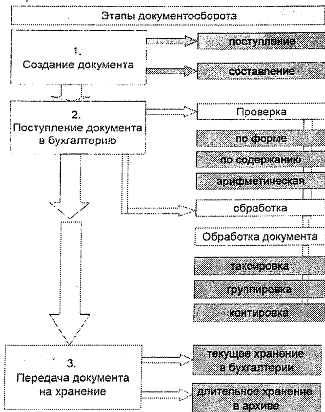
Рисунок 7. Этапы документооборота
