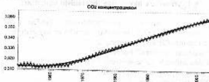
8.2 - rasm. Karbonat anhidrid miqdorining o'zgarishi.
