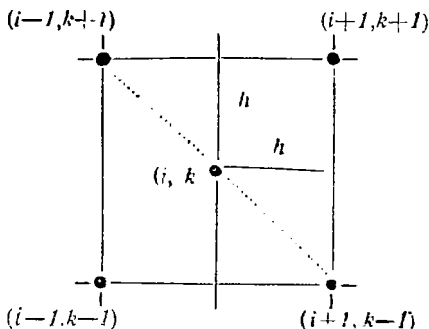
4- чизма
