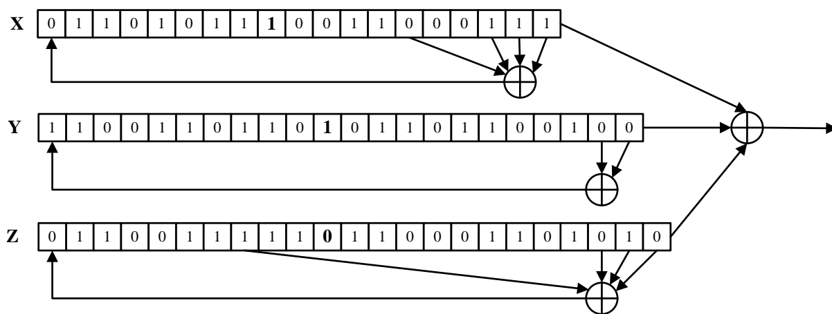
13 - rasm. A5/1 ketma-ketlik generatori
