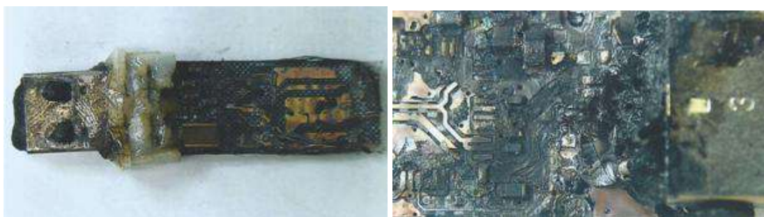
28-rasm. Kuchli magnit maydoni natijasida USB flesh saqlagichining o'zgarishi
