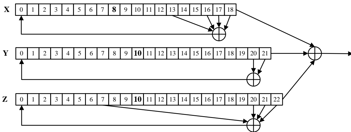
12 -rasm. A5/1 ketma-ketlik generatori
