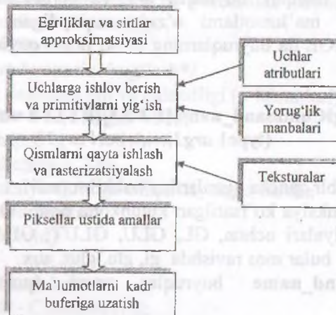
3.2-rasm. OpenGL konveyerining funkcionallashuvi.
