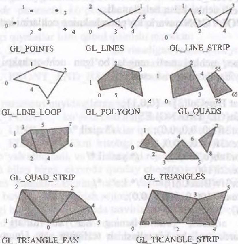
3.3-rasm. OpenGL primitivlari.
