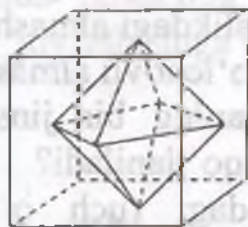
2.4-rasm. Oktaedr.
