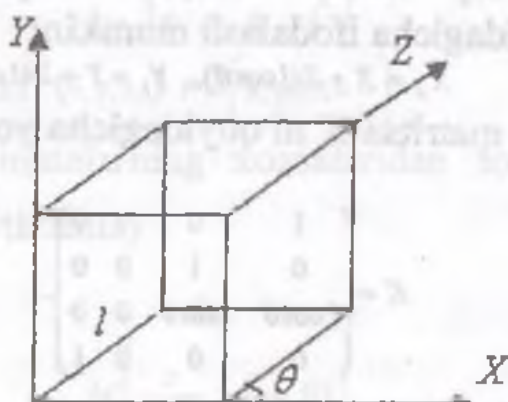
2.7-rasm. Kubning qiya burchakli proeksiyasi.
