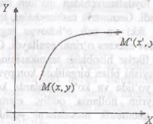
2.1-rasm. Tekislikdagi (ikki o'lchovli) almashtirish.
