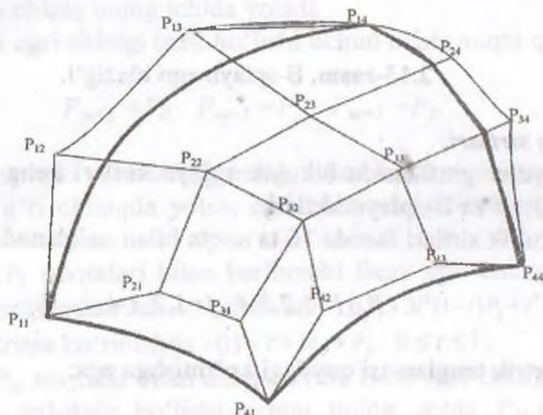
2.14-rasm. Beze splayn sirti.
