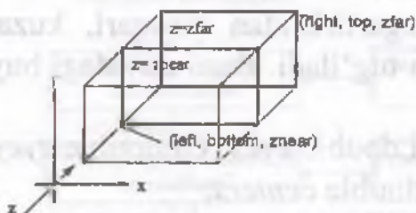
3.6-rasm. Ortografik proeksiya.
