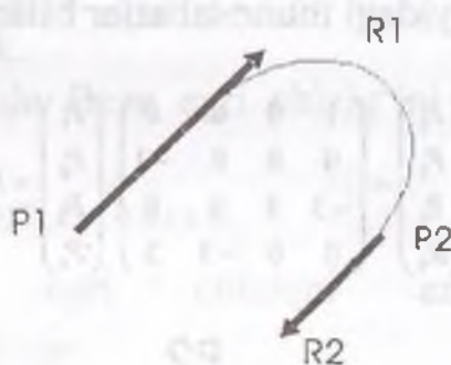
2.11-rasm. Ermit egri chizig'i.
