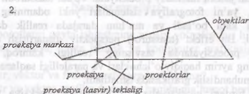
2.5-rasm. Parallel va markaziy proeksiyalar.
