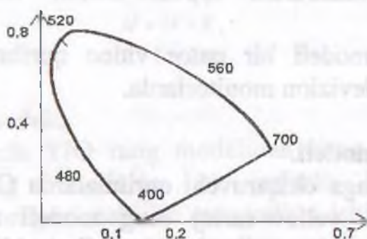
2.28-rasm. Yoritish bo'yicha halqaro komissiyaning rang grafigi.
