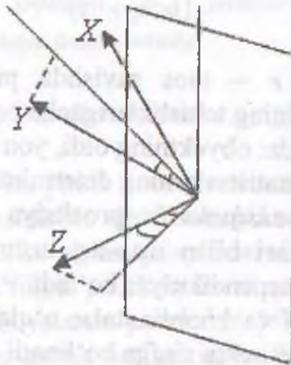
2.6-rasm. Oksonometrik proeksiya.
