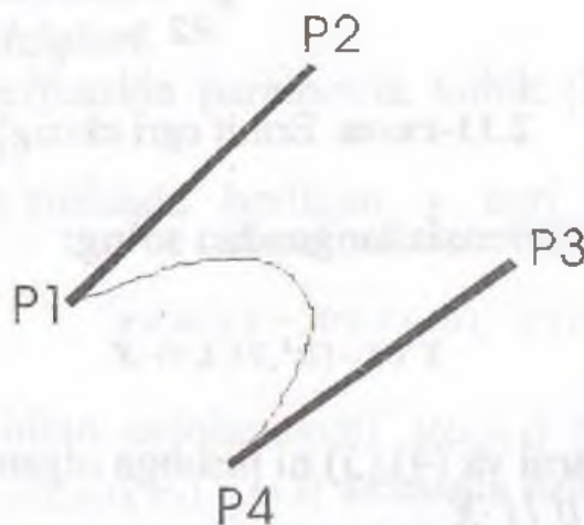
2.12-rasm. Beze egri chizig'i.
