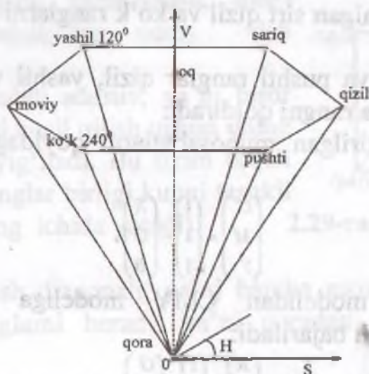
2.30-rasm. HSV olti qirrali konussimon rang modeli.
