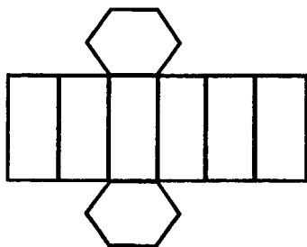
prizma yoyilmasi
