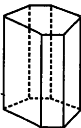
to'g'ri prizma
