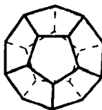
Dodekaedr
