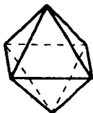
Oktaedr
