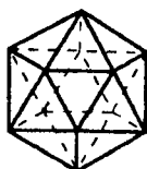
Ikosaedr
