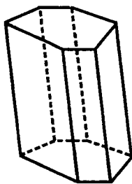
og'ma prizma
