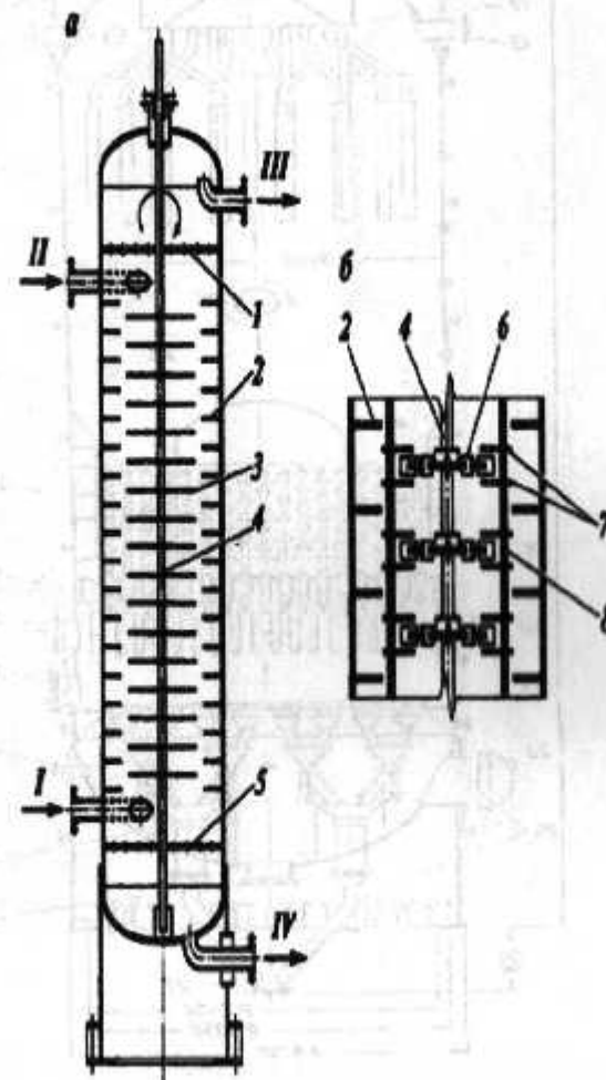
30-rasm. Rotor diskli ekstraktor tuzilishi:
