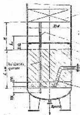
1.5 – rasm. Vertikal suyuqlik yig'gich sxemasi
