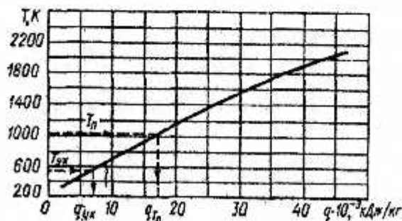
Harorat –entalpiya bog'liqlik grafigi
