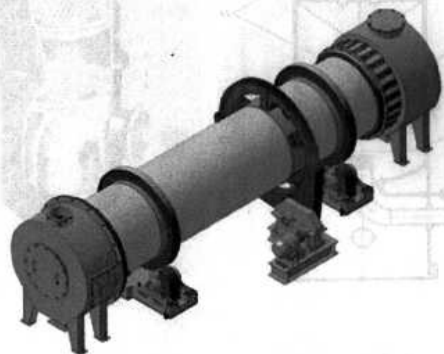
28-rasm. Barabanli quritgich: 1-yuklash kamerasi; 2-qiya tarnov; 3-bandaj; 4-baraban; 5-tishli toj; 6-halqali qoplamalar; 7-tushirish kamerasi; 8-tirgovchi roliklar; 9-uzatma; 10-tayanch roliklari; 11-sektorli nasadka; 12-ko'rakchali nasadka. Oqimlar: I-issiqlik tashuvchi; II-dastlabki mahsulot; III-issiqlik tashuvchi va suv bug'lari aralashmasi; IV-tayyor mahsulot.
