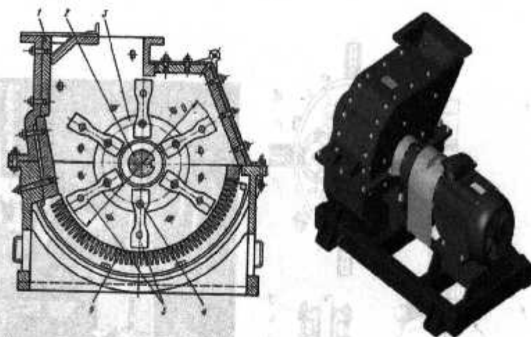
16-rasm. Bolg'ali maydalagich tuzilishi:
