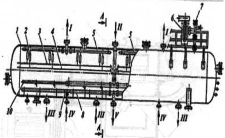
14-rasm. EG200-10 gorizontaal elektrodegidratator tuzilishi:
