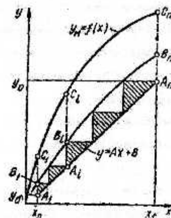
4.11-rasm. Qarama-qarshi yo'nalishli ekstraktorlarda tarelkalar sonini aniqlash
