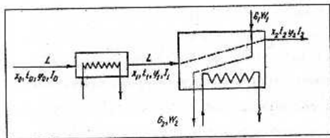
4.3-rasm. Haqiqiy quritgichni hisoblashga doir.
