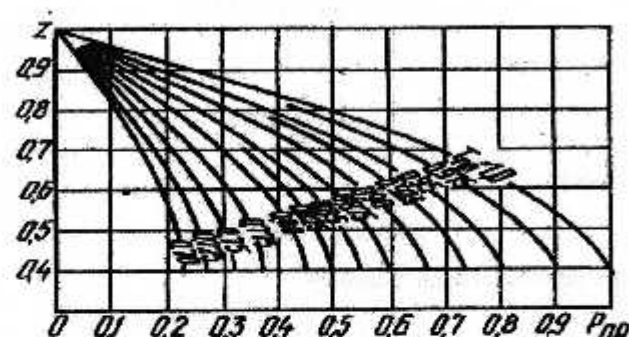
5.3 - rasm. Uglevodorod saqllovchi gazlari past bosimlarda siqiluvchanlik koeffitsientini aniqlash grafigi.
