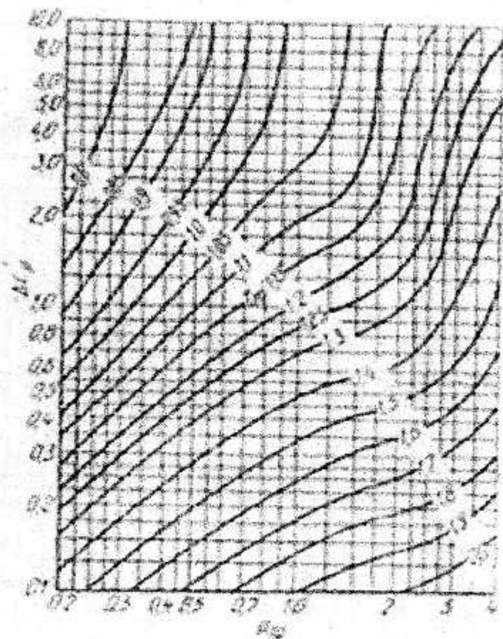
8-rasm. Gazlarni issiqlik saqlashdagi \Delta C_p tuzatmasini aniqlash uchun nomogramma.
