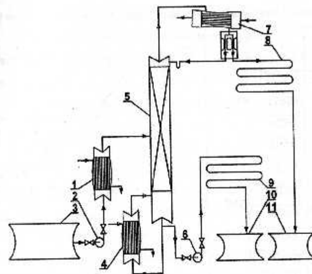
4.15-rasm. Rektifikatsion qurilmaning prinsipial sxemasi:
