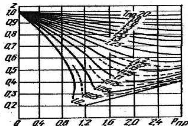
5.4- rasm. Uglevodorod saqllovchi gazlarni yuqori bosimlarda siqiluvchanlik koeffitsientini aniqlash grafigi.
