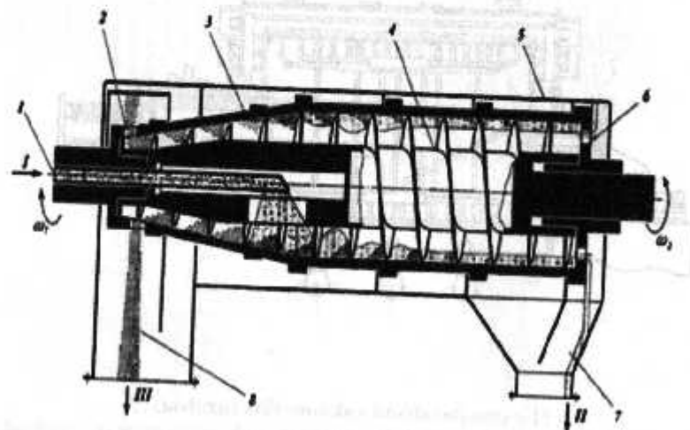
12-rasm. Cho'kmani shnekli tushiruvchi gorizontal cho'ktiruvchi sentrifuga sxemasi: 1-iste'mol trubasi; 2-to'ldirish darchasi; 3-rotor; 4-shnek; 5-qobiq; 6- tushirish darchasi; 7-fugat kamerasi; 8- cho'kma kamerasi. Oqimlar: I – suspenziya; II – fugat; III – cho'kma.
