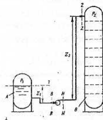
1.1 - rasm. Nasos qurilmasi sxemasi
