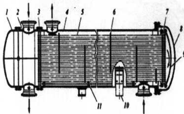
21-rasm. Suzuvchan kallakli qobiq trubali isitkich tuzilishi: 1-taqsimlash kamerasi qopqog'i; 2-taqsimlash kamerasi; 3- qo'zg'almas truba to'ri; 4-qobiq; 5- issiqlik almashinish trubalari; 6- ko'ndalang to'siq; 7- qo'zg'aluvchan truba to'ri; 8- qobiq qopqog'i; 9- suzuvchan kallak qopqog'i; 10- tayanch; 11- trubalar to'plamining aylanuvchi tayanchi.
