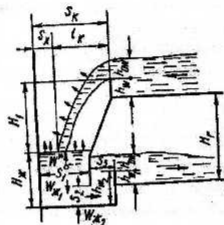
4.12-rasm. Quyilish qurilmalari asosiy kattaliklarining gidravlik hisobi
