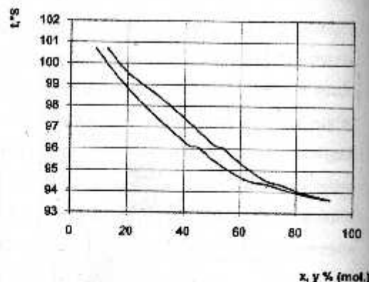
4.16-rasm. t-x,y koordinatalarda doimiy bosim ostida bug' va suyuqlikning muvozanati diagrammasi.
