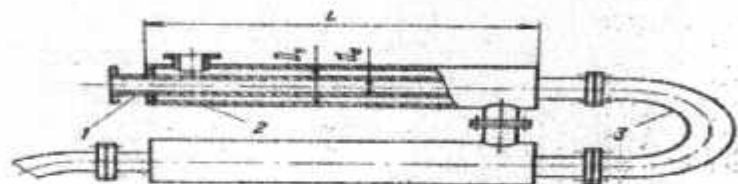
24- rasm. Qo'shtirballisliqlik mashinasi apparati: 1- ichki (kichik) tuba; 2- tashqi (katta) tuba – kojux; 3- kalach.
