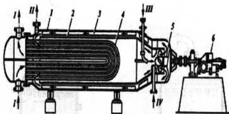
35-rasm. Gorizontal alkillash reaktori tuzilishi: 1-qobiq; 2-sirkulyariya trubasi; 3- qaytarish to'siqlari; 4- trubalar to'plami; 5- parrakli aralashtirgich; 6-uzatma. Oqimlar: I – sovutuvchi agent; II – reaksiya mahsulotlari; III – xom-ashyo.
