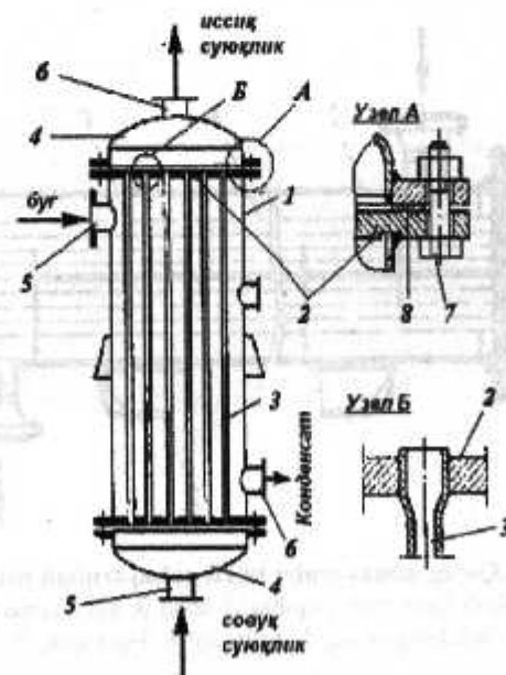
19-rasm. Bir yo'lli qobiq quvurli isitkich:
