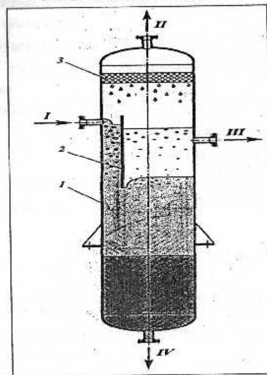
1.4-rasm. Gazoseparator – suv ajratgichning sxemasi:
