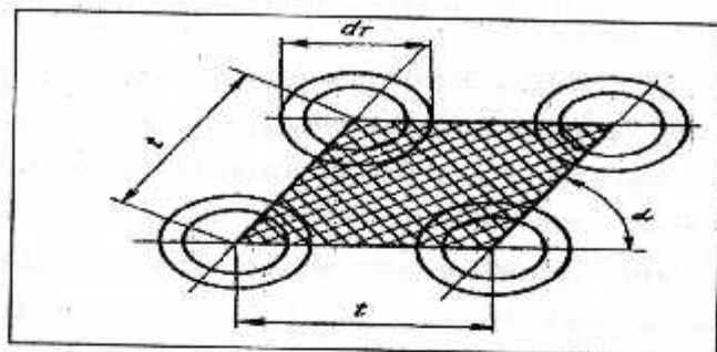
3.2-rasm. Bitta quvur uchun to'ring foydali maydonini aniqlashga doir.
