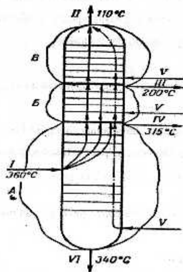
4.13-rasm. Kolonnaning ishlash sxemasi:
