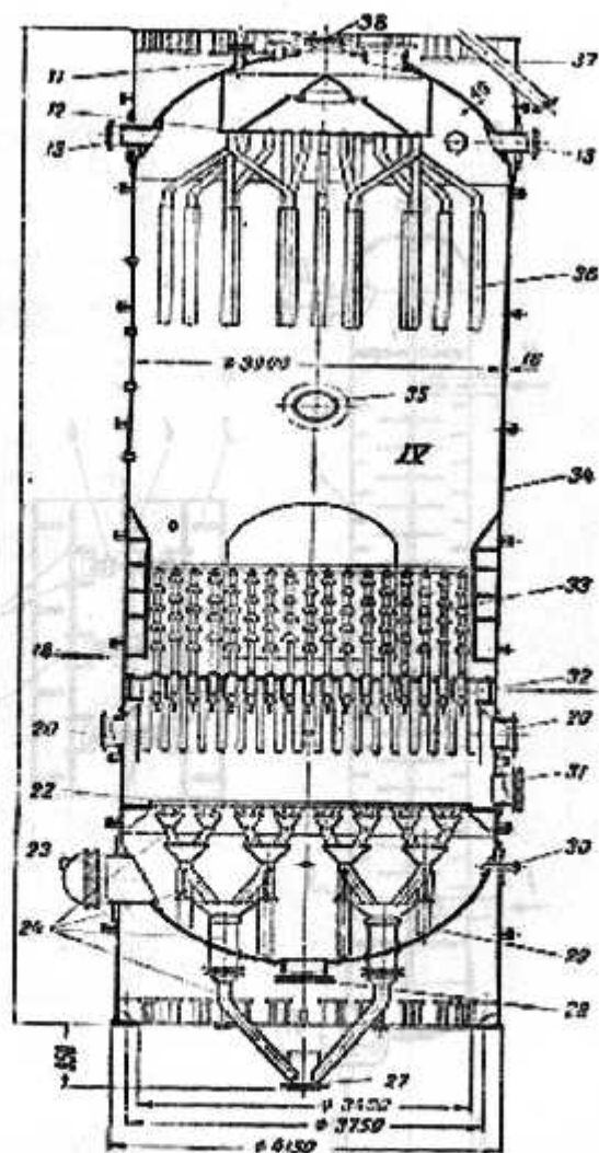
31-rasm. Sharikli katalizatorli kreking qurilmasi reaktori
