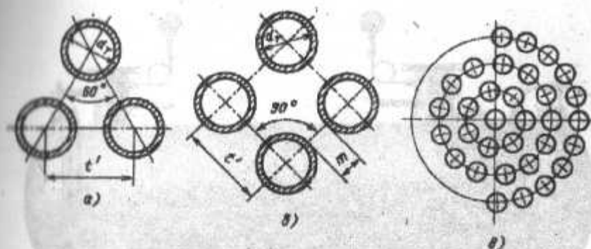
18-rasm. Trubalar chamberagi bo'ylab issiqlik uzatuvchi trubalarni joylashtirish sxemalari: a- olti burchak (teng tomonli uchburchak) kirralari bo'ylab; b- kvadrat kirralari bo'ylab; v- konsentrik aylanalar bo'ylab.
