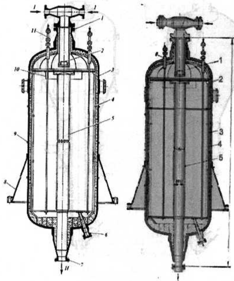
33-rasm. Xomashyo radial harakat qiluvchi katalitik riforming reaktori: 1-xomashyoning kirishi uchun shtuser; 2-xomashyo taqsimlagichi; 3-qobiq; 4-quticha; 5-reaksiya mahsulotlari yig'gichi; 6-katalizatorni tushirish uchun shtuser; 7-reaksiya mahsulotlarini tushirish uchun shtuser; 8-tayanch; 9-termopara uchun mufta; 10-silindrsimon stakan; 11-ko'p zonali termopara. Oqimlar: I-xomashyo; II-reaksiya mahsulotlari.
