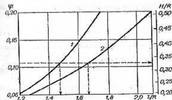
4.5-rasm. O'txona to'ldirish ko'effitsienti \varphi ning material qatlami xordasi l_{xm} (1) va material yoyining uzunligi l_{dm} bilan bog'liqligi.
