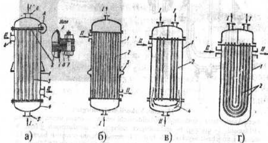
17-rasm. Kojux-trubali issiqlik almashinish apparatlari: a- bir yo'lli; b- linzasimon kompensatorli; v- harakatchan qopqoqli; g- U shaklidagi trubkali; 1- kojux; 2- issiqlik o'tkazuvchi trubalar; 3- linzasimon kompensator; 4- harakatchan qopqoq; 5- trubalar chamberagi; 6- qopqoq; 7,8- shtutserlar; 9- bolt; 10- qistirma.
