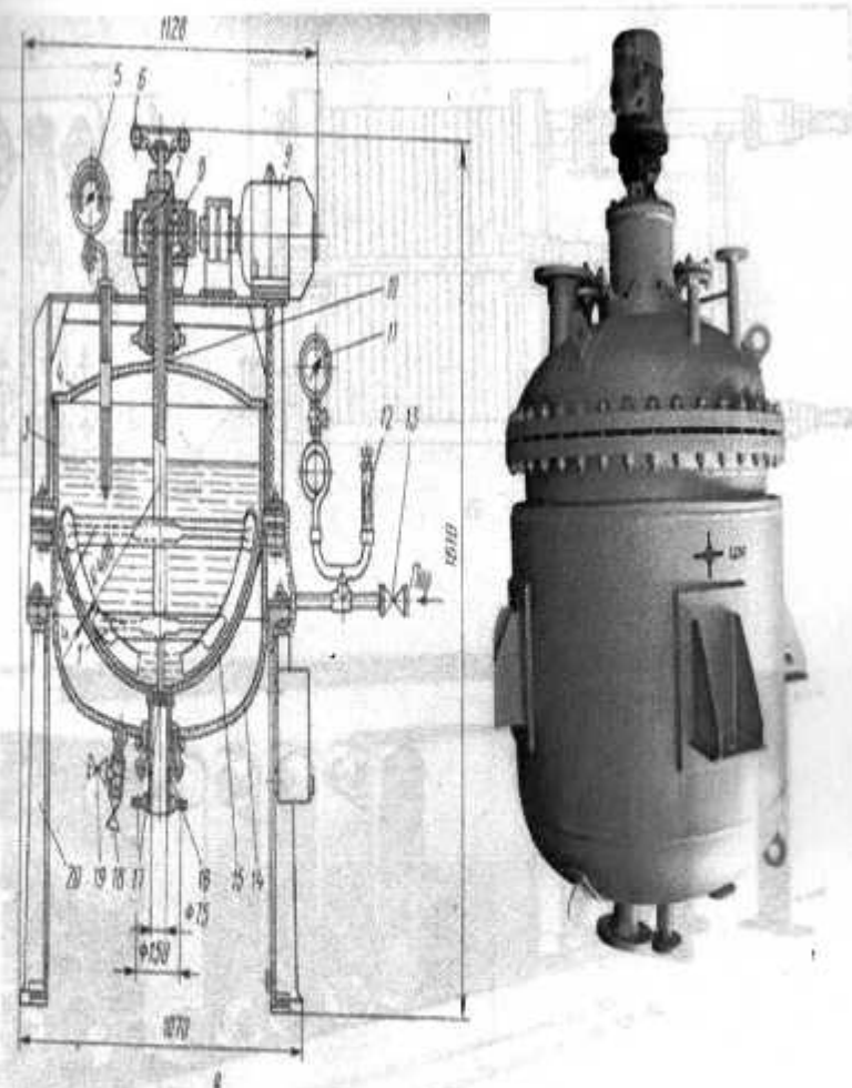
26- rasm. Davriy ishlovchi qizdirish apparat: 1- yakorli-parrakli aralashtirgich; 2- parrak; 3- obechayka; 4- qopqoq; 5- manometrik termometr; 6- maxovikcha; 7- vint; 8- chervyakli reduktor; 9- elektrodvigatel; 10- ichi bo'shval; 11- manometr; 12- muhofaza klapani; 13- bug' ventili; 14- metall qobiq; 15- sferik misqozon; 16- mahsulotni tushirishpa trubkasi; 17- klapan; 18,19- kondensat ventili; 20- cho'ya nasoslar.
