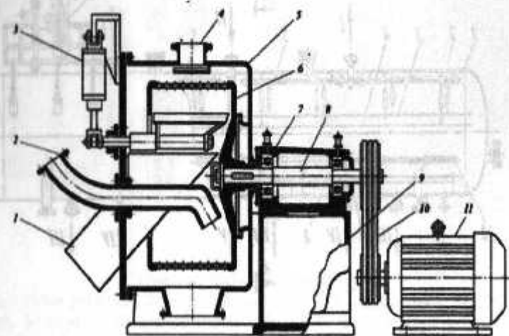
13-rasm. Cho'kmani pichoq yordamida tozalovchi gorizontal sentrifuga tuzilishi: 1-bo'shatish bunkeri; 2- to'ldirish trubkasi; 3- cho'kmani kesish mexanizmi; 4- havoni chiqarish trubkasi; 5-qobiq; 6-rotor; 7-val tayanchlari; 8-val; 9-stanina; 10- tasmali uzatma; 10-elektrodvigatel.
