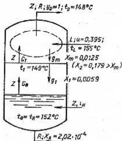
4.14-rasm. bug'lash (maydon) kolonnasi shoxiga doir (masalaga qarang)
