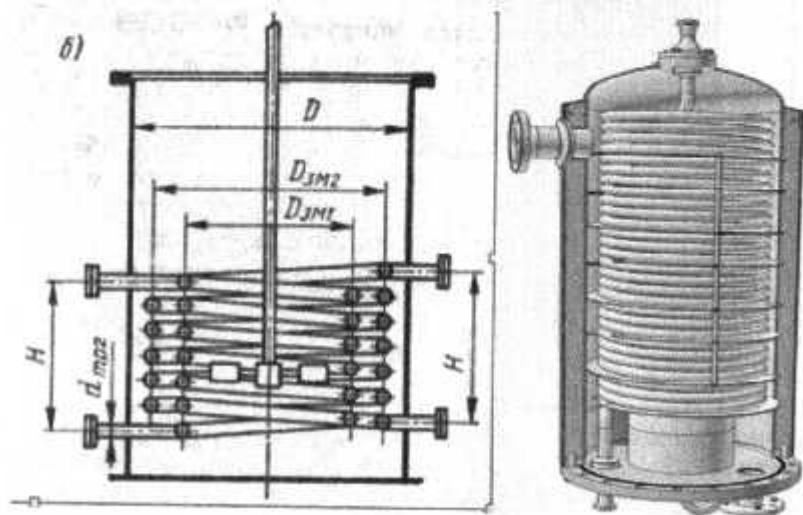
25- rasm. Zmeevikli apparat sxemasi: a- bir o'ramli; b- ikki o'ramli; D- apparatni ichki diametri; D_{zm1} - zmeevik o'rami diametri; D_{zm2} - tashqi zmeevik o'rami diametri; d_{m1} , d_{m2} - zmeevik trubasining diametri; H- zmeevik balandligi; Z - zmeevik o'ramining qadami.
