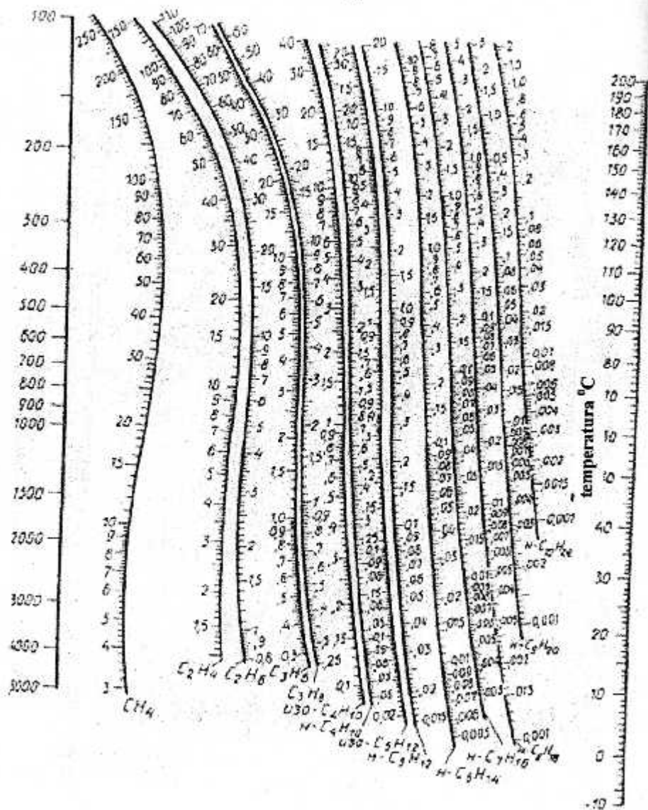
2-rasm. Yuqori haroratlarda uglevodorodlar fazoli tenglik konstanti aniqlash uchun nomogramma.
