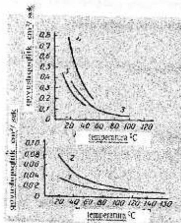
1.2-rasm. Neft va neft mahsulotlari kinematik qovushqoqligining haroratga bog'liqligi.
