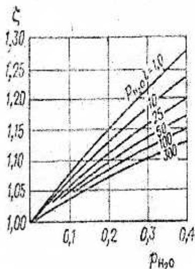
4.8-rasm. Tuzatish koeffitsienti \zeta ni aniqlash grafiki.
