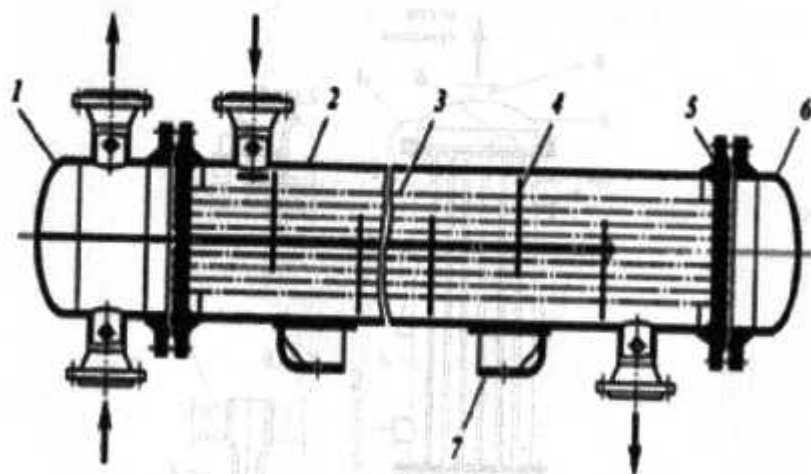
20-rasm. Qo'zg'almas truba to'ri qobiq trubali isitkich tuzilishi: 1-taqsimlash kamerasi; 2-qobiq; 3-issiqlik almashinish trubkalari; 4-ko'ndalang to'siq; 5- truba to'ri; 6-qopqog; 7-tayanch.
