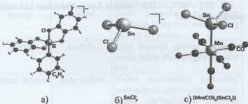
4.9-rasm. Komplekslarning tuzilishi
