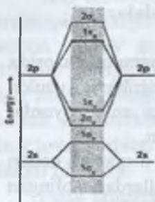
2.8-rasm. 2-davr elementlari F_2 va N_2MO diagrammalari
