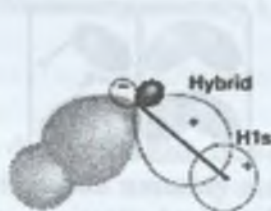
2.24-rasm. H_2O dagi OH lokallashgan orbitallari hosil bo'lishida O atomining gibrid orbitallari va H1s qatnashadi. Bu gibrid orbitallar sp^3 shaklda bo'lishi 2.6- rasmda ko'rsatilgan.
