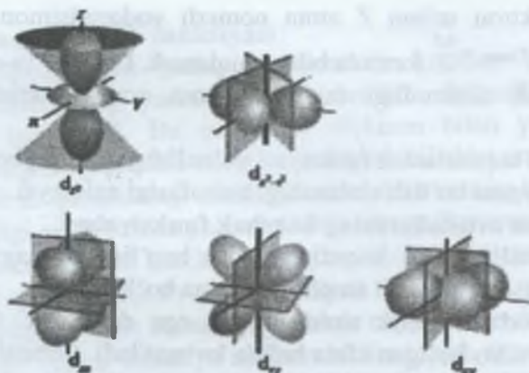
1.13-rasm. d-orbitallarning chegara tekisliklari ko‘rinishlaridan biri. To‘rtta orbitallar ikkita o‘zaro perpendikulyar yadro orqali o‘tuvchi tugun yuzalariga ega. d_{x^2} – orbitali uchlari yadroda birlashadigan konussimon tugun yuzalariga ega.
