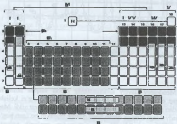
1.20-rasm. Davriy sistemaning asosiy shakli
