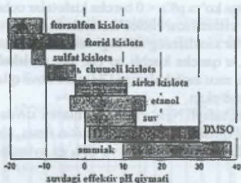
4-rasm. Har xil erituvchilardagi kislota va asoslarning kuchlari diapazoni. Diapazon kengligi erituvchining avtoprotoliz doimiyligiga ( pK_{sol} )
