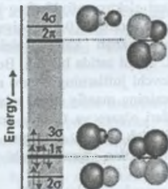
2.14-rasm. CO ning molekulyar orbitallarning sxematik tasviri, atom o'chamlari bilan magnit hossalarini tasviri bilan bog'liqligi.
