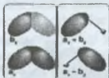
2.23-rasm. H_2O molekulasida ikkita band 1a_1 va 1b_2 orbital-larning yig'indisi va ayirmasi.
