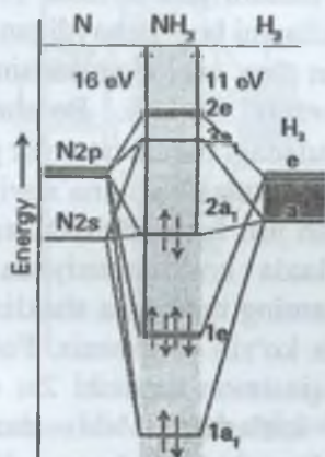
2.21-rasm. NH_3 ning molekuly orbitalarning elektron holatlar diagrammasi.
