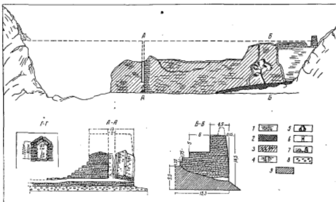
Abdullaxonbandining fasadi va ko'ndadalang kesimlari 27
