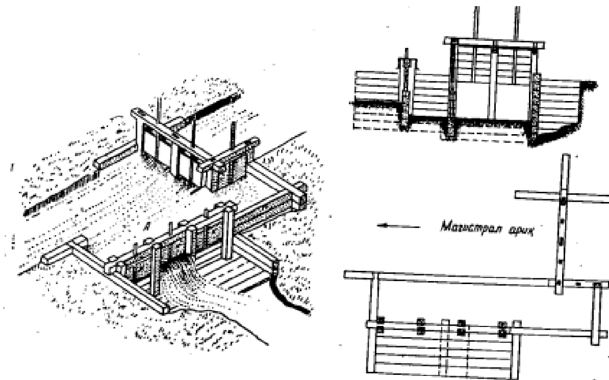
1899 yilda Samarqand irrigatsiya sestemalariga oʻrnatilgan dastlabki injenerlik tipidagi inshootlar. 38
