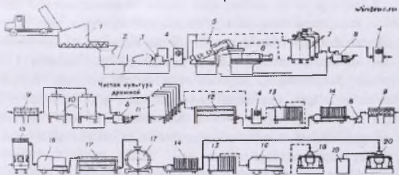
7-rasm. Nimnordon va nimshirin vinolarni kupaj yo'li bilan tayyorlash sxemasi: 1 - qabul qilish bunker; 2- valkli uzum maydalagich; 3- mezonasos; 4- sulfitodozator; 5- stekatel; 6 - press; 7 - sharbatni mezgada damlash uchun rezervuarlar; 8 - nasos; 9 - ingredientlar dozatori; 10 - sharbatni tindirish uchun moslamasi; 11- bijg'itish qurilmasi; 12 - ultrasovutkich; 13 - pasterizator; 14 - filtr; 15 - vinoni potokda tindirgich; 16 - diatomit filtri; 17 - past haroratda saqlash uchun
