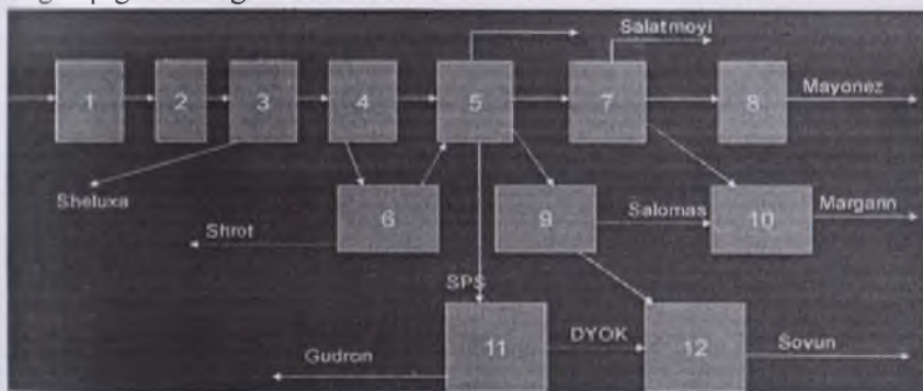
6-rasm. Yog'-moy kombinatining umumiy sxemasi quyidagi sxemada keltirilgan bo'lib, unda xomashyo va material harakati bo'yicha ishlab chiqarish bo'limlarining ketma-ketligi
