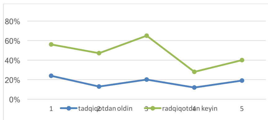
2.4-rasm. Natijalarni taqqoslash uchun chiziqli grafikdan foydalanish usuli
