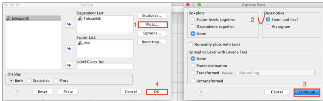
18.32. Rasm. «Novdasimon va yaproqsimon» diagrammani qurish.
