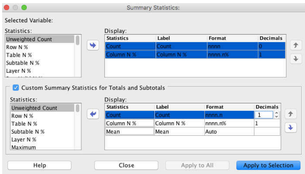
26.18. Rasm. Mobil jadvallardagi qiymatlarni bir xil ko`rinishga keltirish uchun o`nliklarni belgilash.
