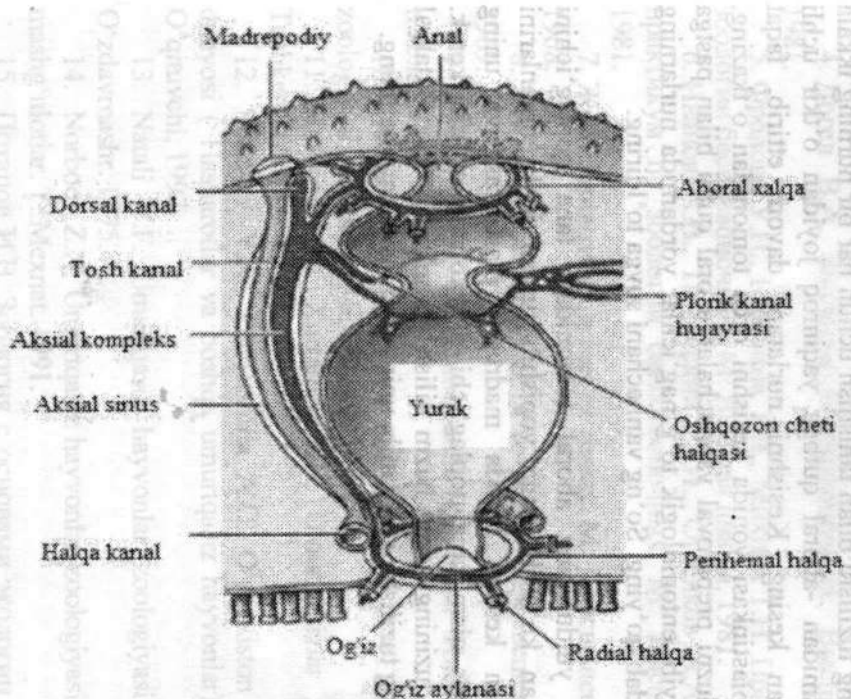
78-rasm. 44 Dengiz yulduzining markaziy qismini ichki tuzilishi.
