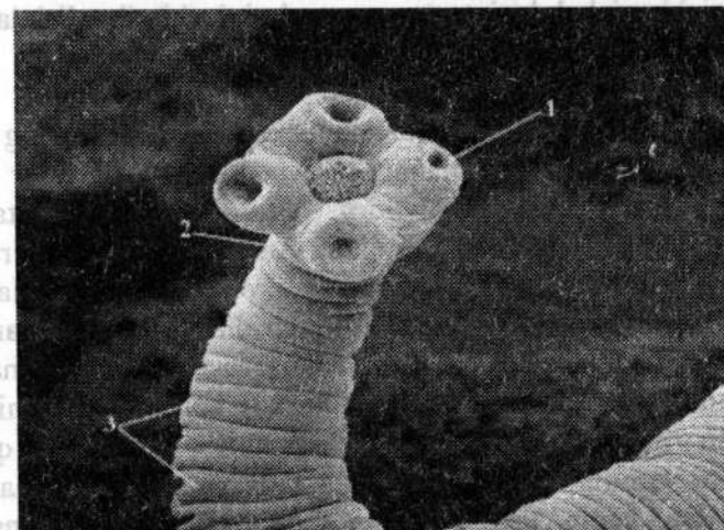
34-rasm 23 . Qoramol solityori ( Taeniarhynchus saginatus ) bosh (skoleks)ning ustki tomonidan ko‘rinishi: 1- so‘rg‘ich; 2-bo‘yin qismi; 3-bo‘g‘imlar.
