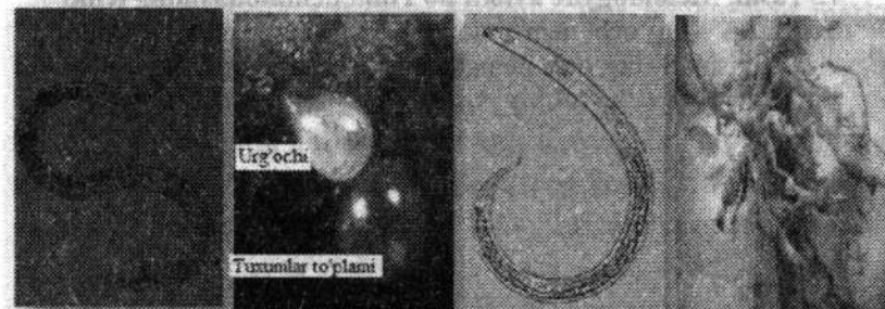
74-rasm. Meloidogyne avlodi bo'rtma nematodasining tashqi tuzilishi va zararlagan ildiz
