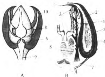
Dengiz tipratikanining zaharli globifer peditsellyariyasi (A) va uning tuzilishining sxemasi (B): 1-eshik uchi; 2-bezli epiteliy; 3-sensor tuklar; 4-asab tolasi; 5-halqasimon mushak; 6-zaharli bez ichi; 7-paylar; 8-keltiruvchi mushak; 9-ohakli shox; 10-eshik.
